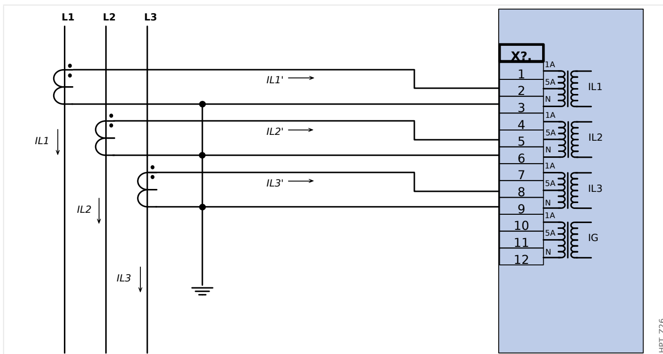
Fig. 23: Mesure de courant triphasé; In sec = 5 A
