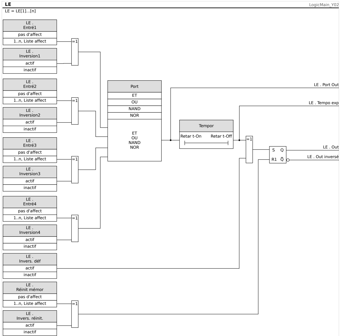
Fig. 89: Présentation détaillée - Diagramme logique global.
