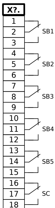
Fig. 14: RO-5 - Marquage des bornes
