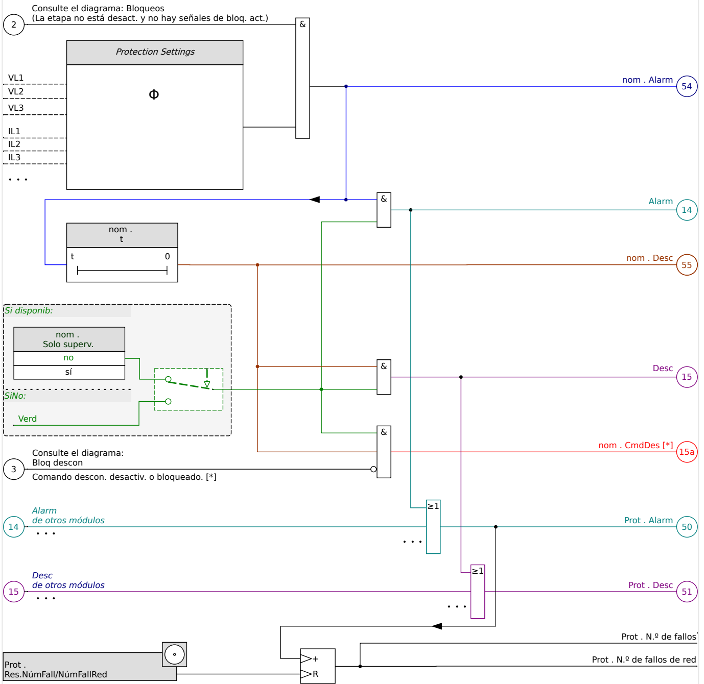
Fig. 49: Descripción a grandes rasgos de la funcionalidad de cualquier elemento de protección de HighPROTEC.
