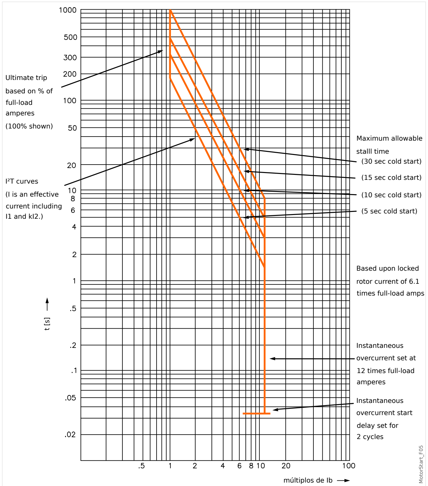
Fig. 57: Curva de protección de motor (ejemplo 1).
