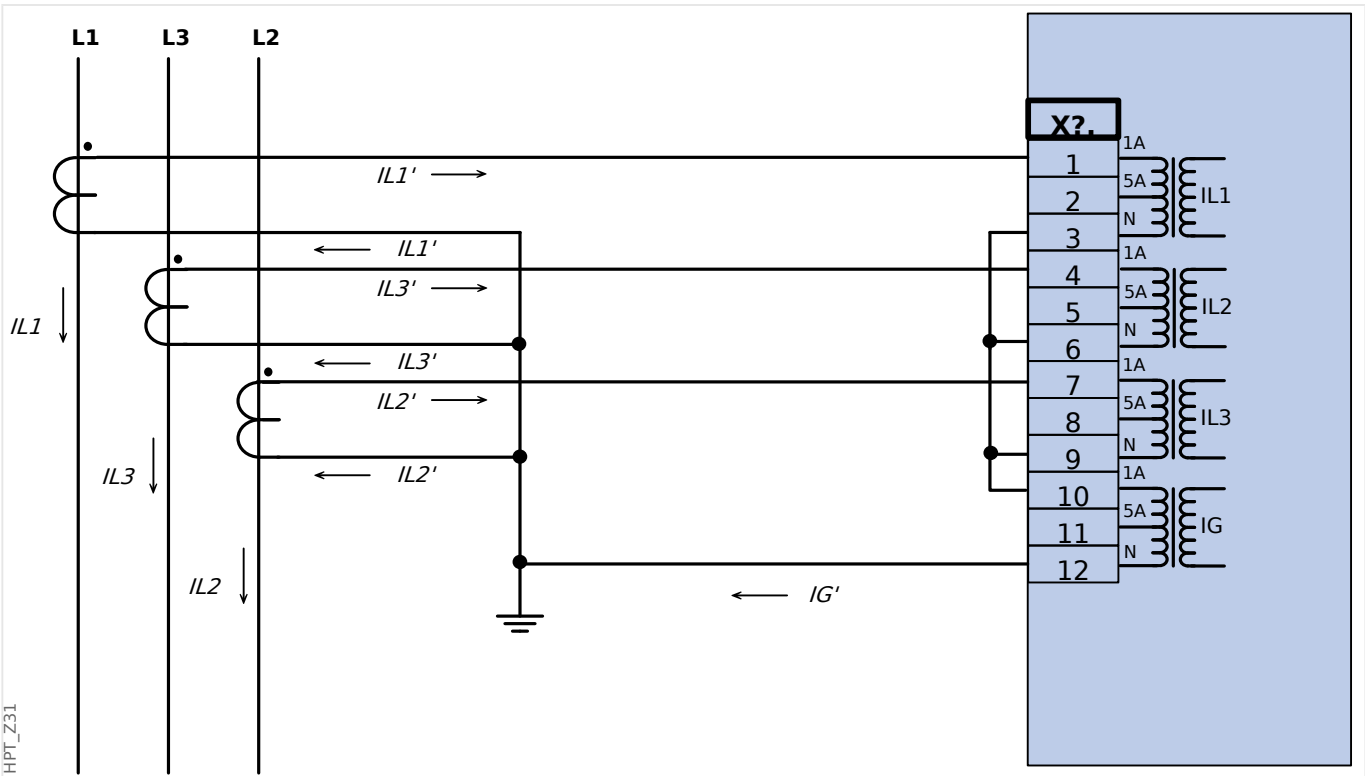
Fig. 28: Medida corriente trifásica; En secundario = 1 A. Medic corr de tierra mediante conexión Holmgreen; IGnom secund = 1 A.
