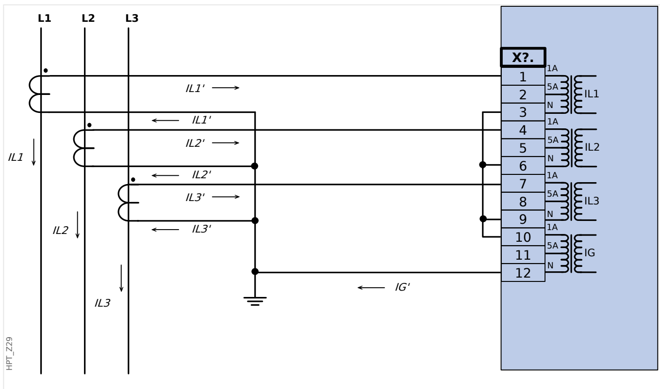
Fig. 26: Medida corriente trifásica; En secundario = 1 A. Medic corr de tierra mediante conexión Holmgreen; IGnom secund = 1 A.
