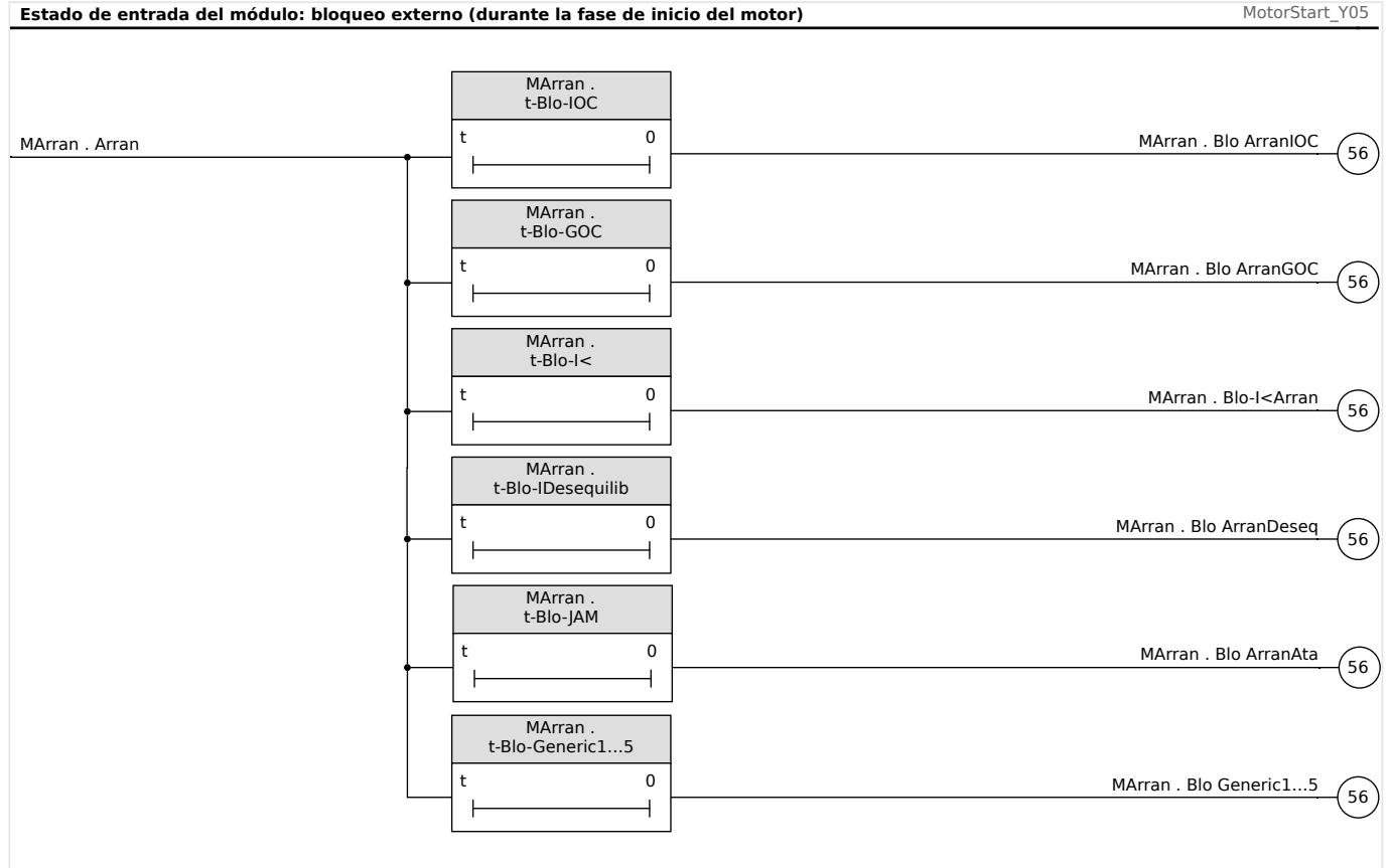
Fig. 51: Bloqueo temporal de las funciones de protección de corriente durante el arranque del motor.
