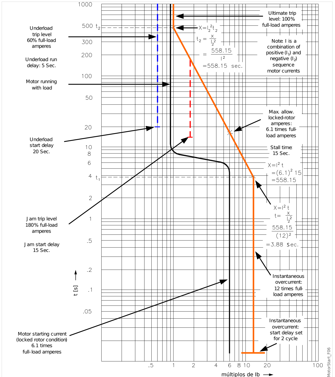
Fig. 58: Curva de protección de motor (ejemplo 2 sin RTD).
