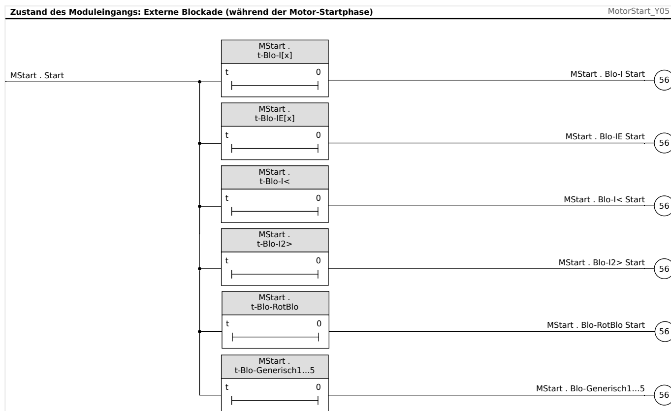
Abb. 51: Temporäre Blockade von Stromschutzfunktionen während Motorstarts.
