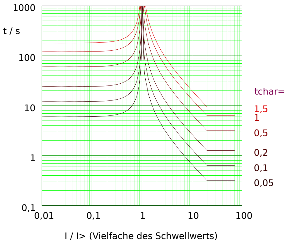
Abb. 65: LINV: Rückfallverzögerung (linke Hälfte, I < I_{max} ) und Auslöseverzögerung (rechte Hälfte, I > I_{max} ), Beispieldiagramm für I_{max} = 20 \cdot I_{nom} .
