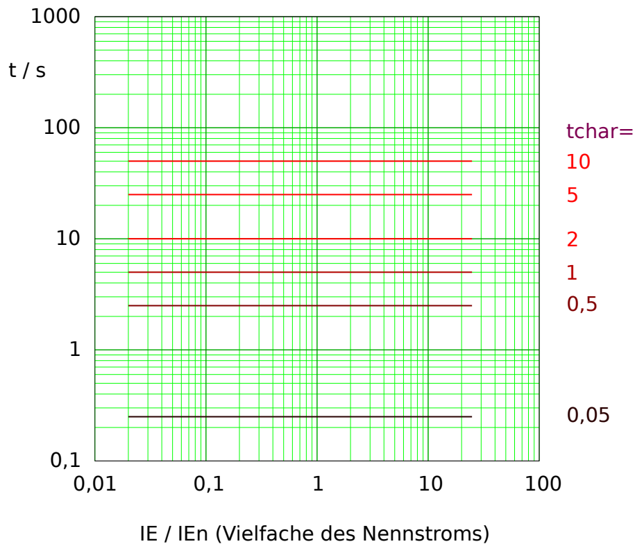
Abb. 83: Auslösekurve „Therm Flat“, wobei nur der Bereich IE > IE> jeweils anwendbar ist. Beispieldiagramm für gemessenen (nicht empfindlichen) Erdstrom.
