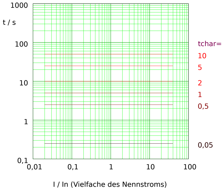
Abb. 70: Auslösekurve „Therm Flat“, wobei nur der Bereich I > I_n jeweils anwendbar ist.
