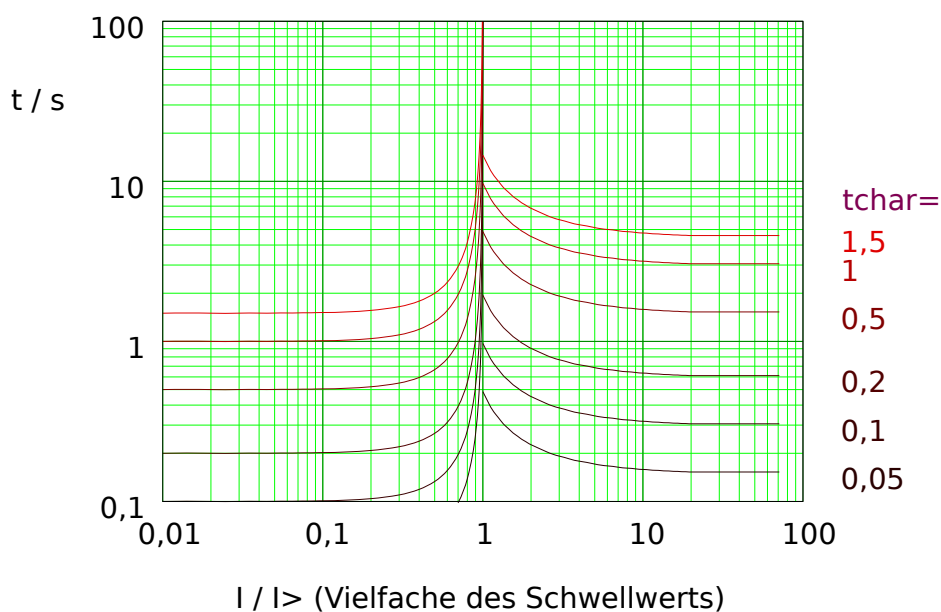
Abb. 69: RINV: Rückfallverzögerung (linke Hälfte, I < I_{max} ) und Auslöseverzögerung (rechte Hälfte, I > I_{max} ), Beispieldiagramm für I_{max} = 20 \cdot I_{nom} .
