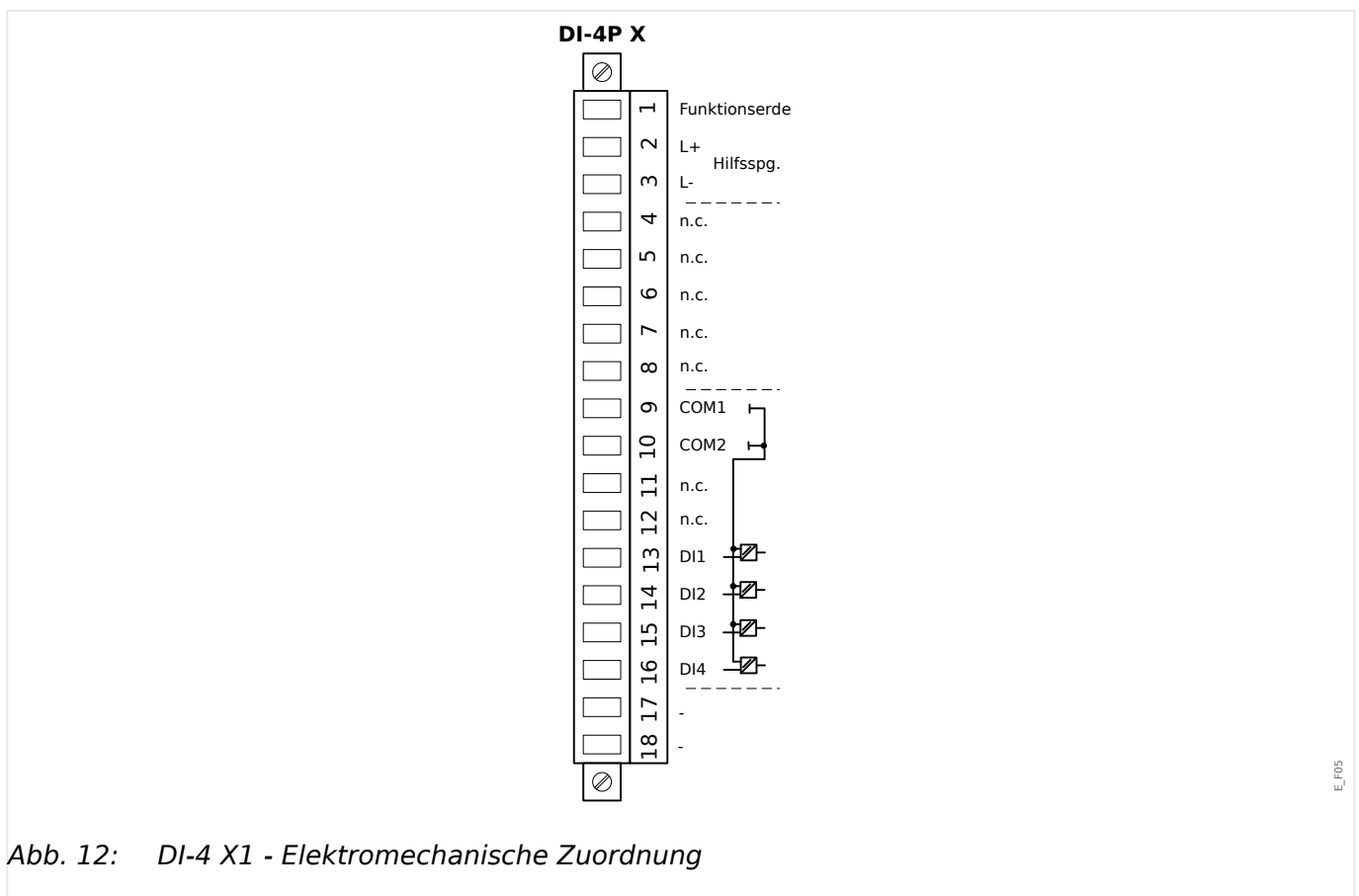
Abb. 11: DI-4 X1 - Klemmenbelegung
