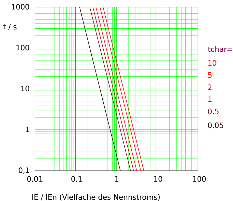
Abb. 86: Auslösekurve „I4T“, wobei nur der Bereich IE > IE_{n> jeweils anwendbar ist. Beispieldiagramm für gemessenen (nicht empfindlichen) Erdstrom.
