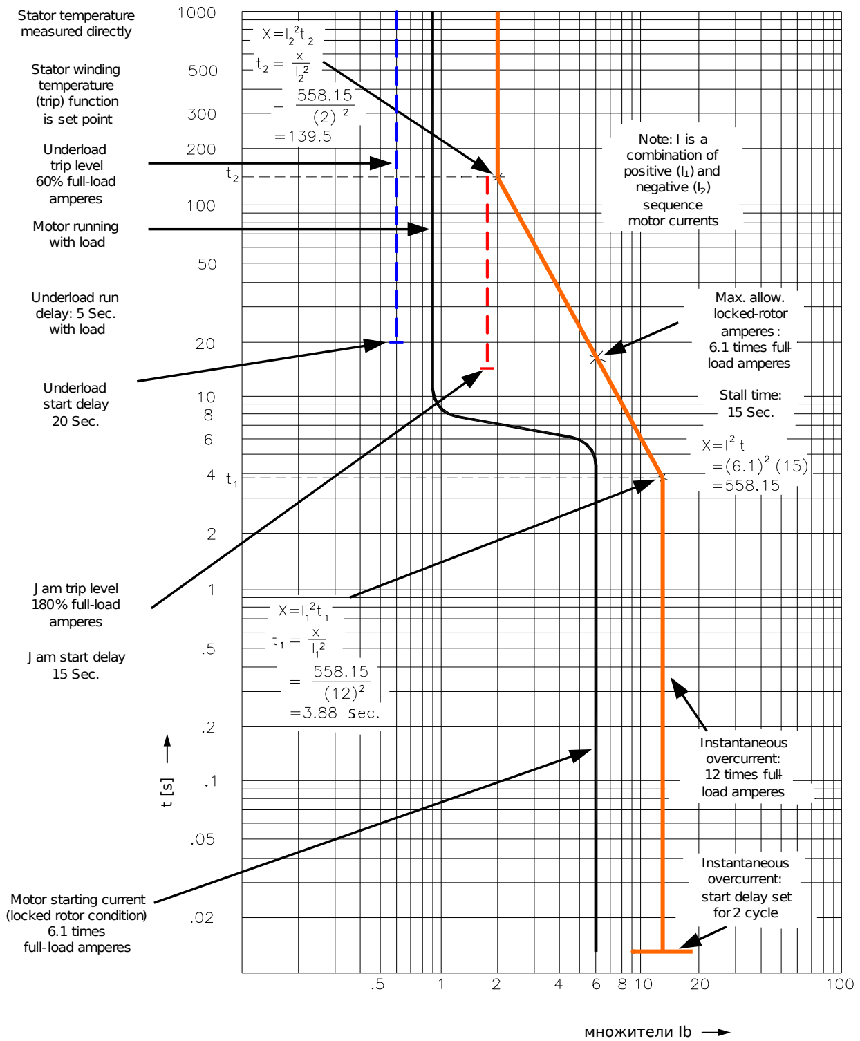
Рис. 57: Кривая защиты двигателя (пример 3 — с ТДС).
