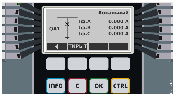
Рис. 67: Пример страницы управления, выключатель в замкнутом положении.
