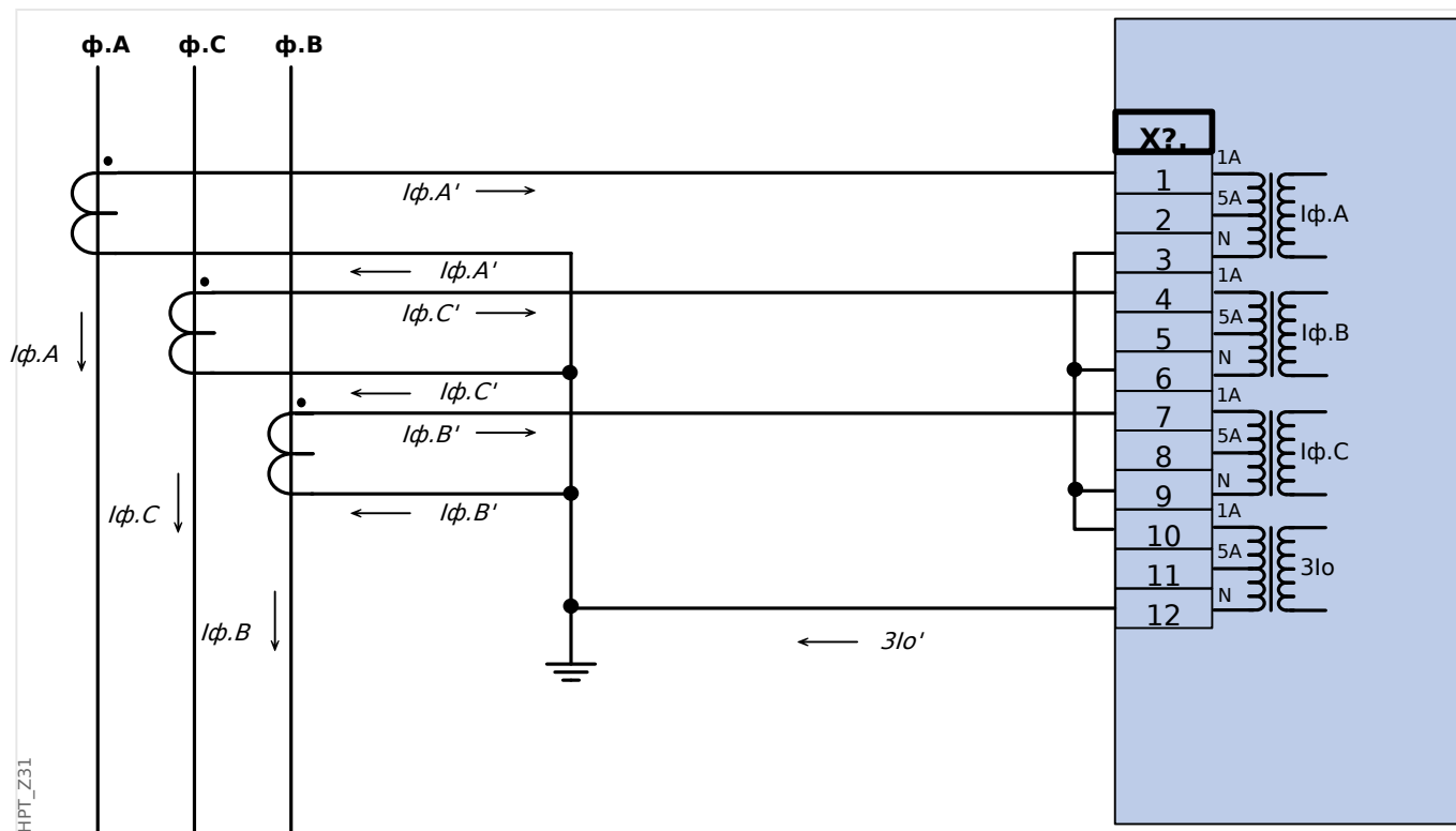
Рис. 28: Измерение фазных токов по схеме «полной» звезды; I_n вторичн. = 1 А. Ток на землю, измеряемый через соединение по схеме Холмгринна 3I_o . ном. втор. = 1 А.
