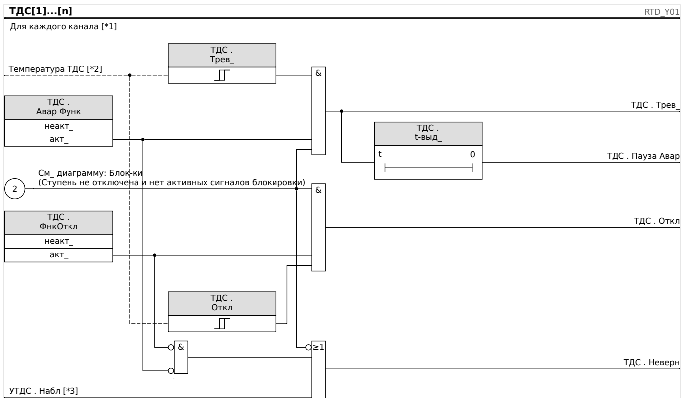
Рис. 63: Общий принцип работы (аварийный сигнал с задержкой, отключение без задержки).
