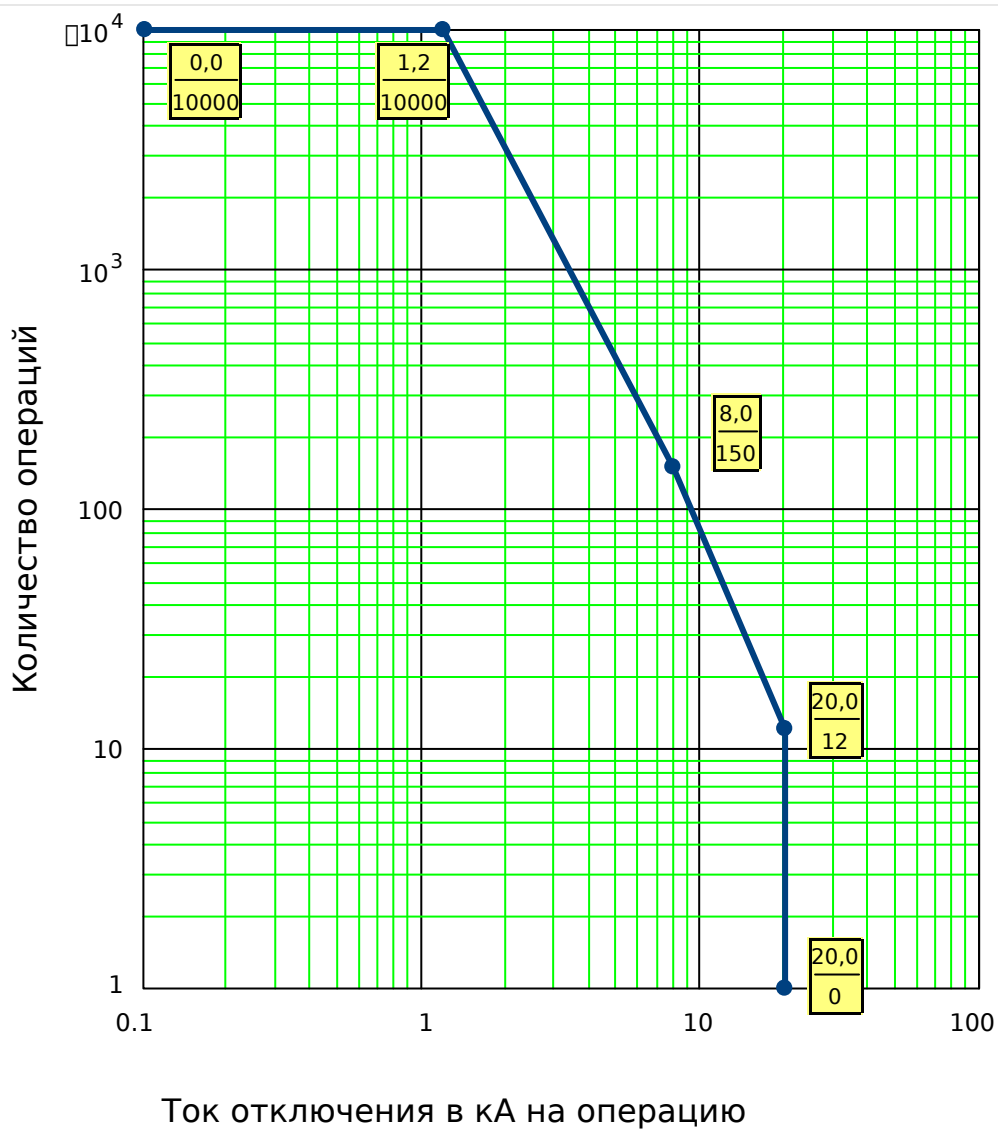
Рис. 72: Эксплуатационная кривая выключателя для типичного выключателя 25кВ
