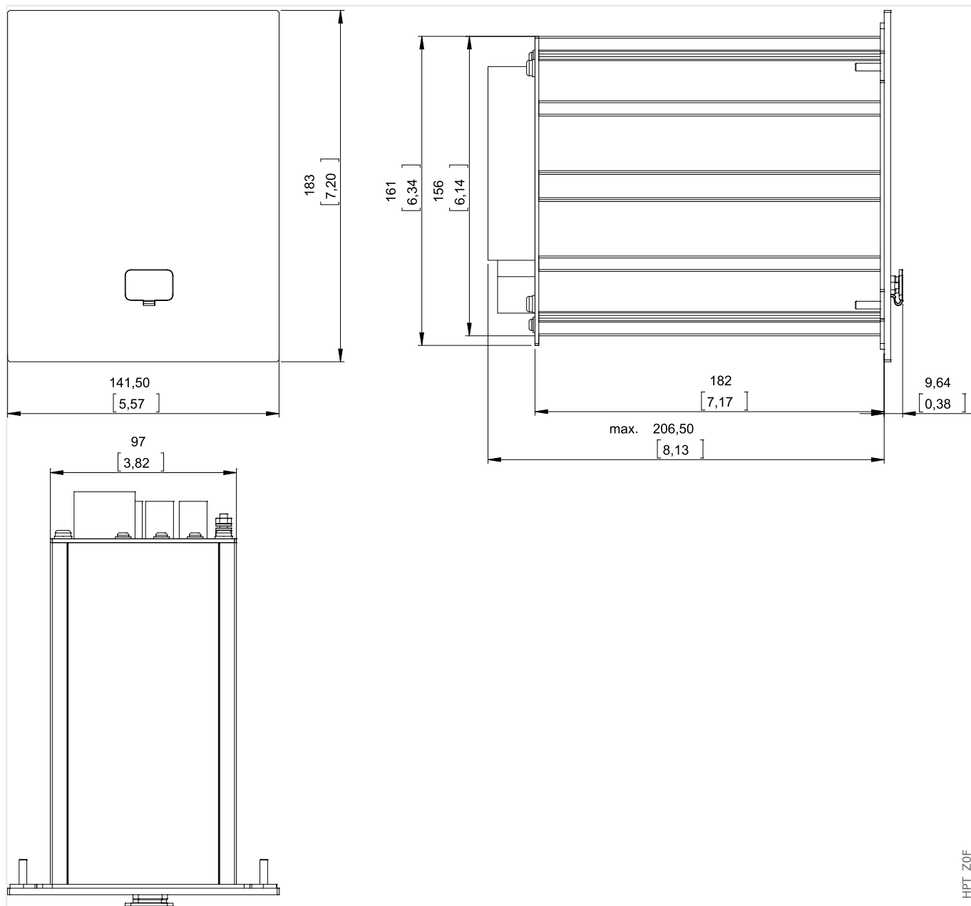
Рис. 5: Корпус В1: внешний вид (устройства с 8 кнопками). (Все размеры указаны в миллиметрах, за исключением размеров в квадратных скобках — [дюймы].)
