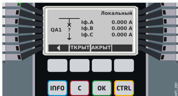
Рис. 68: Пример страницы управления, выключатель в аварийном (недопустимое состояние) положении.
