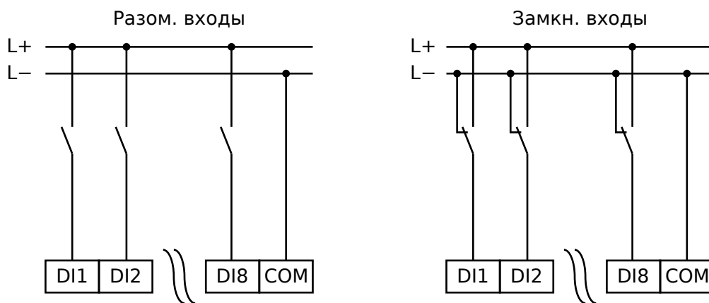
Рис. 88: Безопасное состояние цифровых входов
