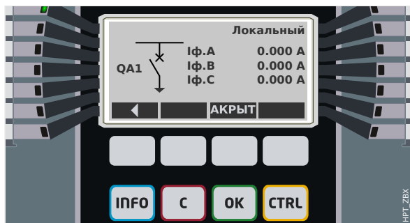
Рис. 69: Пример страницы управления, выключатель в разомкнутом положении.
