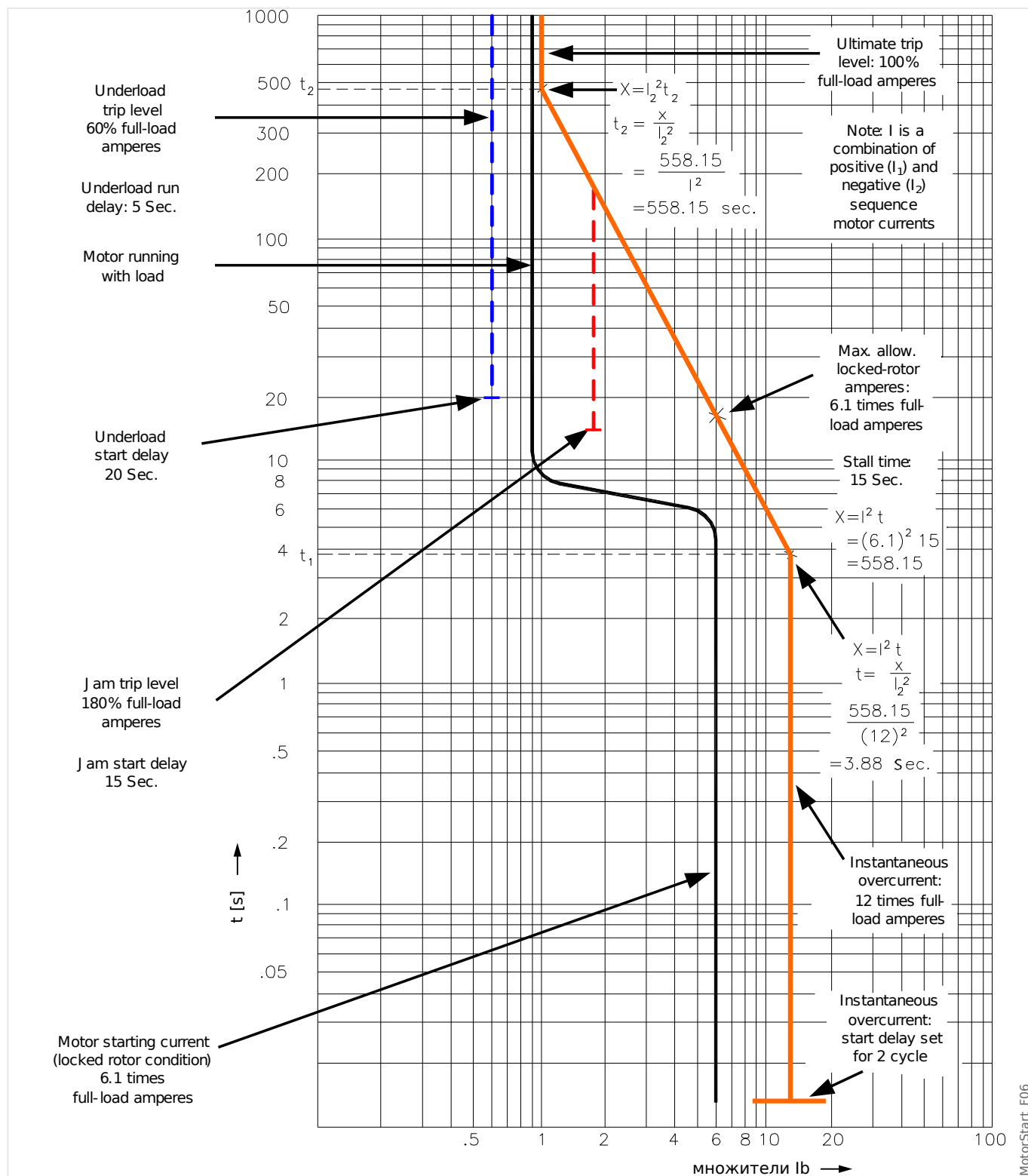
Рис. 56: Кривая защиты двигателя (пример 2 — без ТДС).
