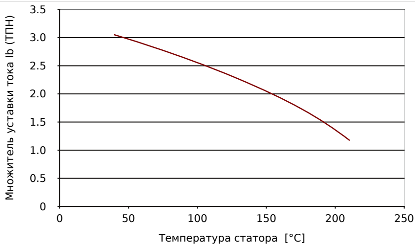
Рис. 52: Эффективная уставка тока по ср. с максимальной температурой статора.
