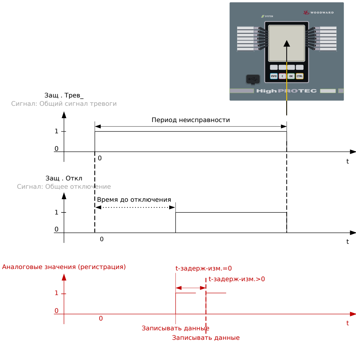
Рис. 77: Регистратор неисправностей: время и длительность.
