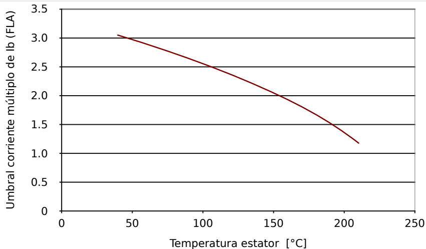
Fig. 52: Umbral corriente efectiva frente a temperatura máxima estator.
