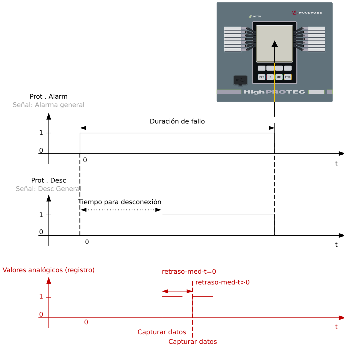
Fig. 77: Registrador de fallos: tiempos y duraciones.
