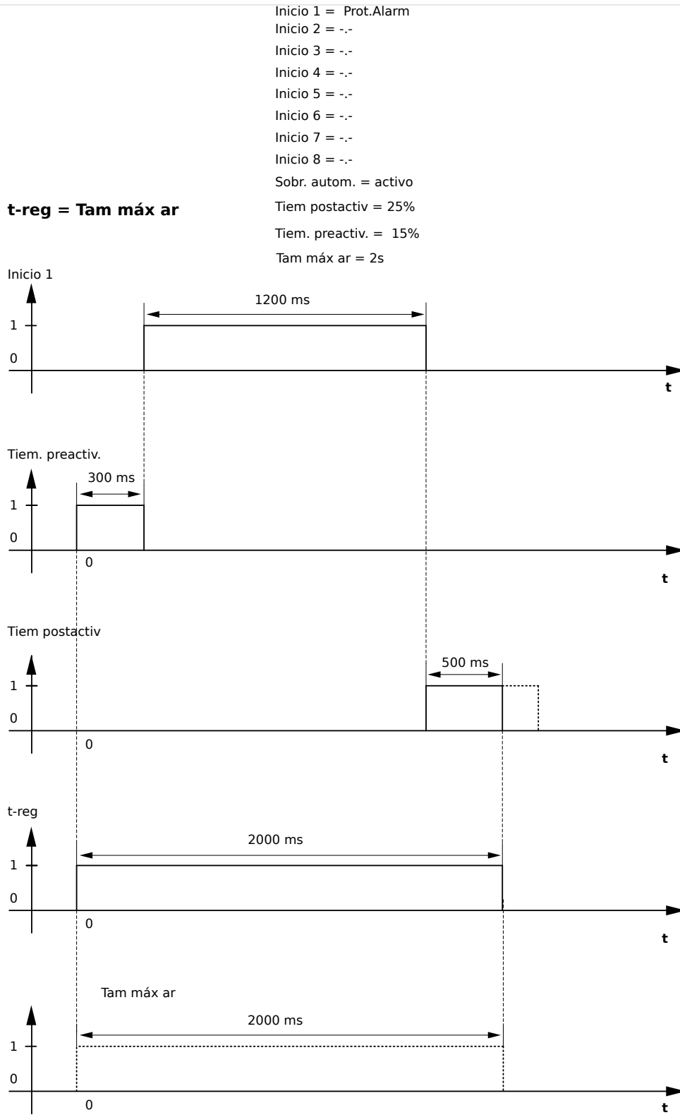
Fig. 75: Ejemplo 1: cuadro de intervalos del registrador de perturbaciones
