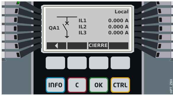
Fig. 69: Ejemplo de página de control, con el circuito en posición abierta.
