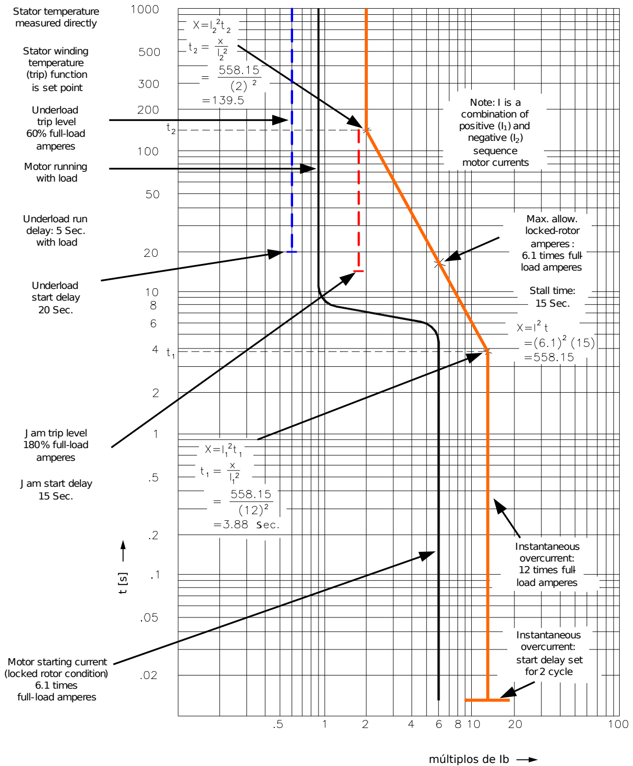
Fig. 57: Curva de protección de motor (ejemplo 3 con RTD).
