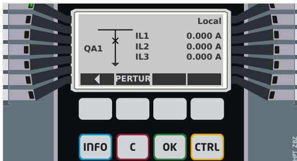
Fig. 67: Ejemplo de página de control, con el circuito en posición cerrada.
