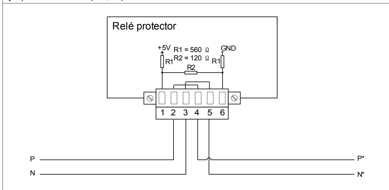
Ejemplo de cableado de tipo 1, Dispositivo en el medio de BUS
