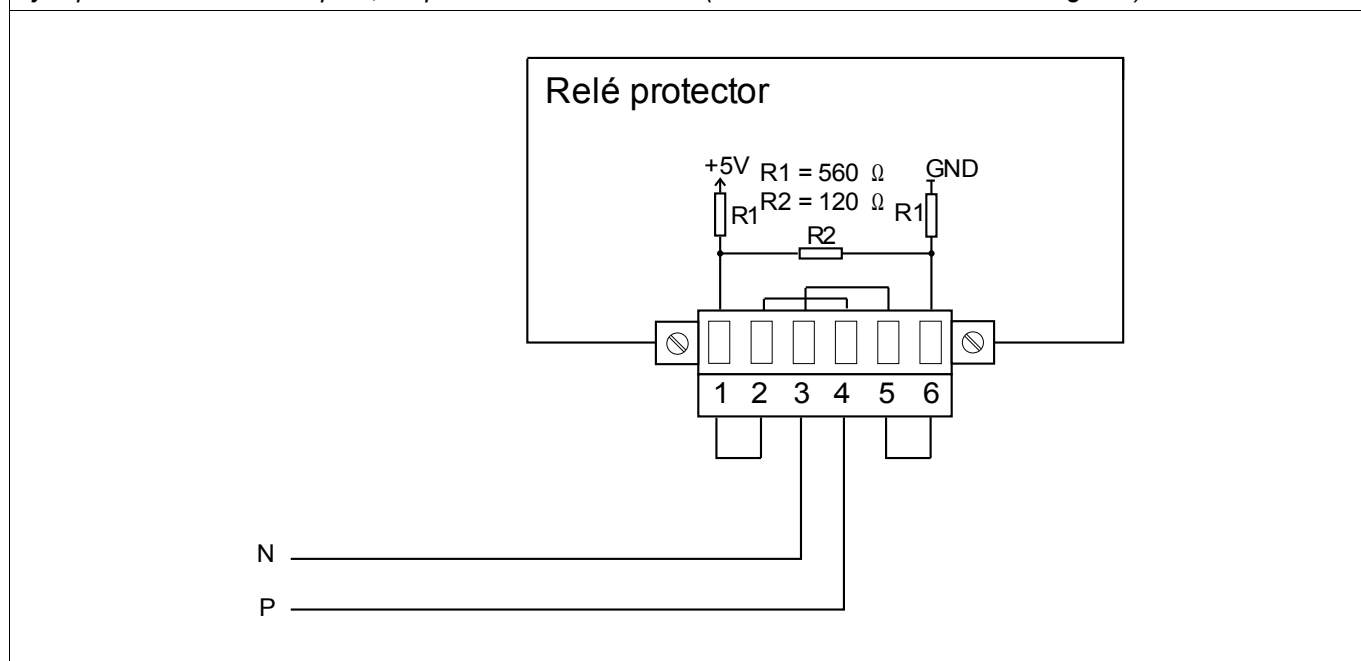
Ejemplo de cableado de tipo 1, Dispositivo al final de BUS (con el resistor de terminal integrado)
