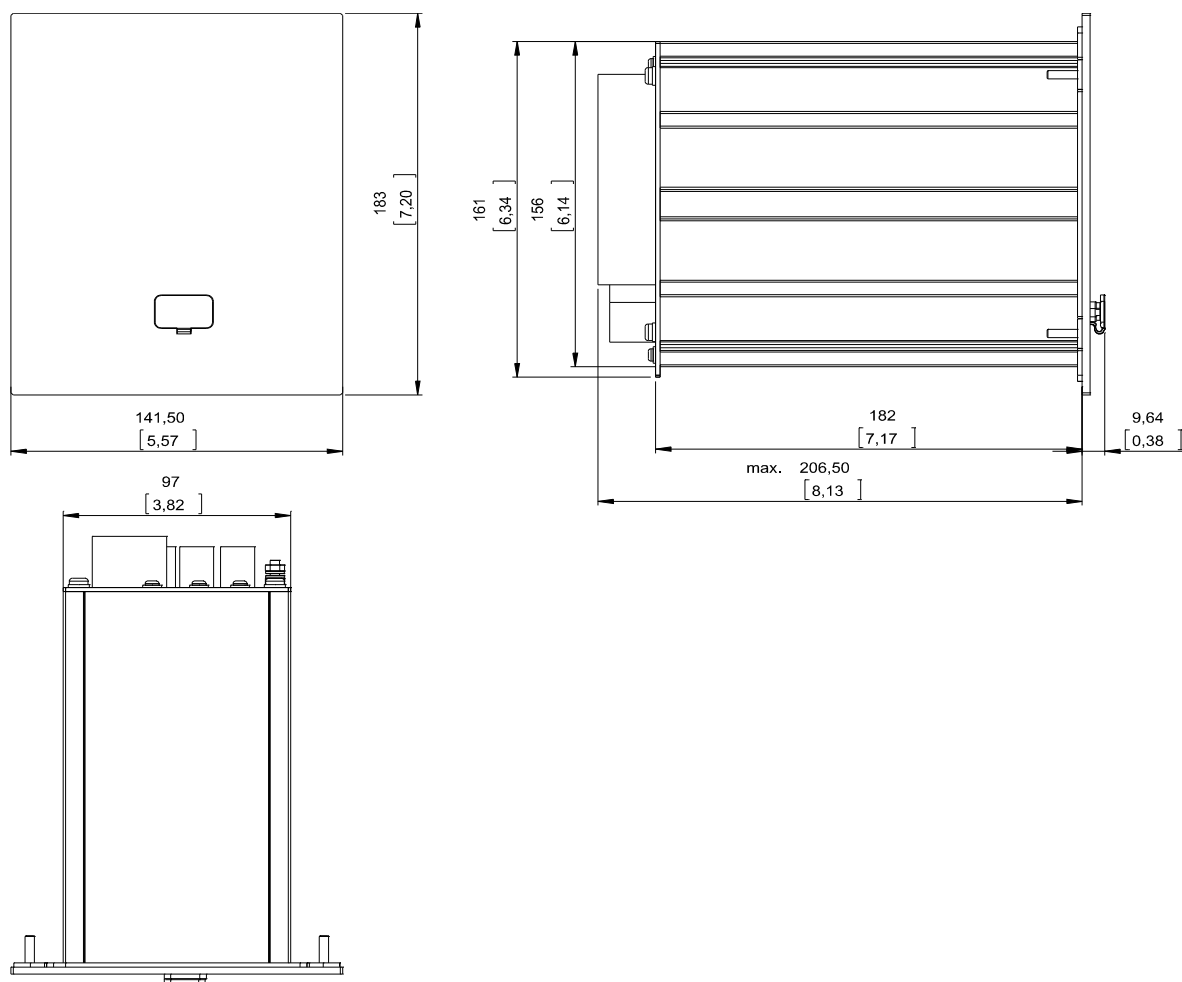
Корпус В1: вид с трех сторон (устройства с 8 кнопками)
