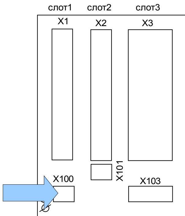
Задняя сторона устройства (слоты)
