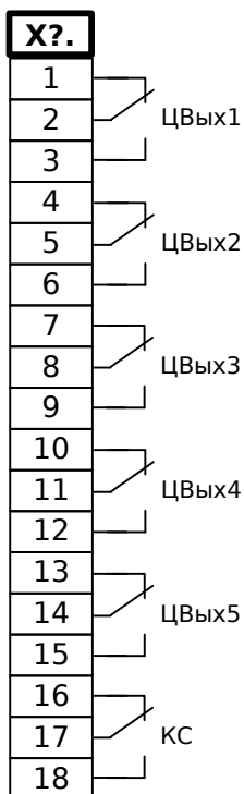
Рис. 12: RO-5 — обозначение разъемов
