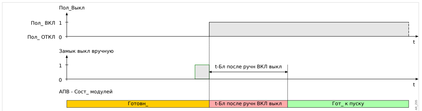
Рис. 60: Состояния автоматического повторного включения во время замыкания выключателя вручную.
