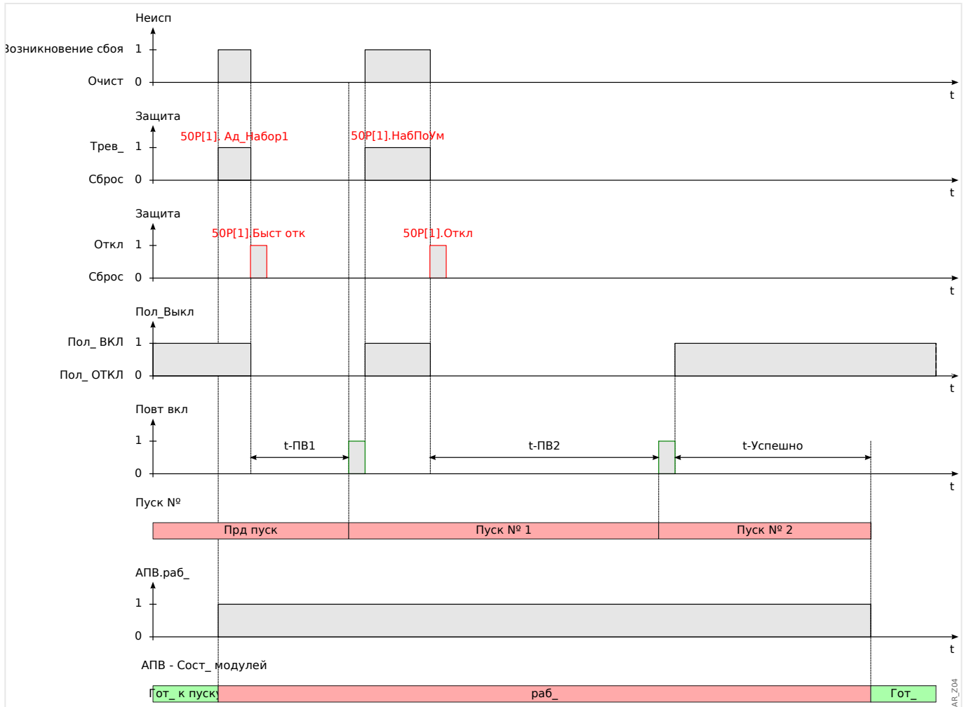
Рис. 59: Диаграмма синхронизации автоматического повторного включения для схемы с 2 успешными попытками автоматического повторного включения и ускорением перед импульсом.
