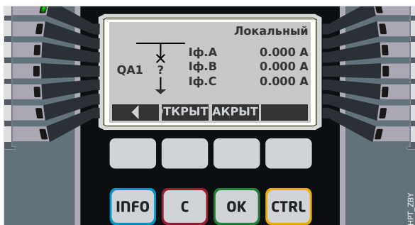
Рис. 70: Пример страницы управления, выключатель в аварийном (недопустимое состояние) положении.
