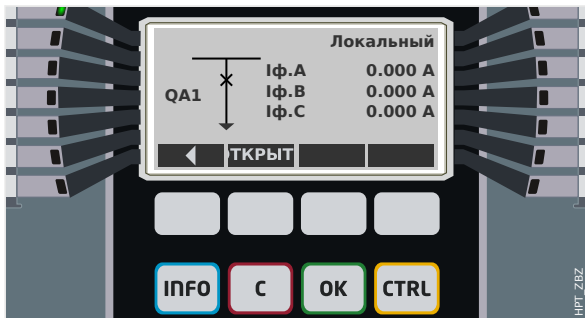
Рис. 69: Пример страницы управления, выключатель в замкнутом положении.
