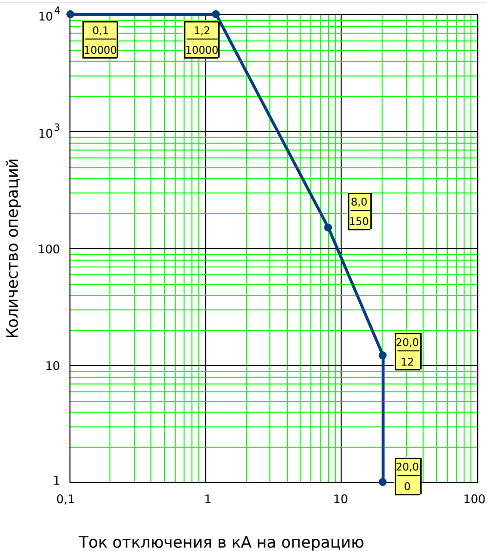
Рис. 74: Эксплуатационная кривая выключателя для типичного выключателя 25кВ
