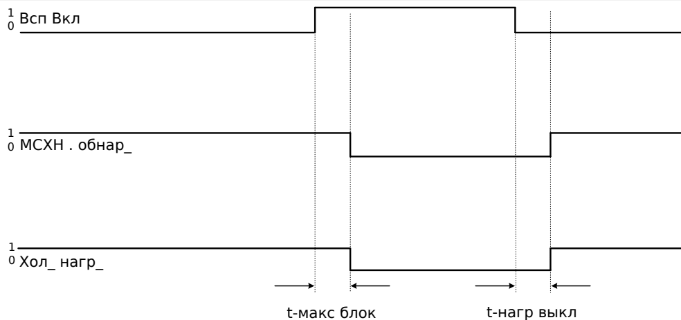
Рис. 64: Пример: Положение выключателя.
