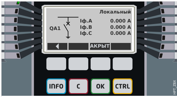
Рис. 71: Пример страницы управления, выключатель в разомкнутом положении.
