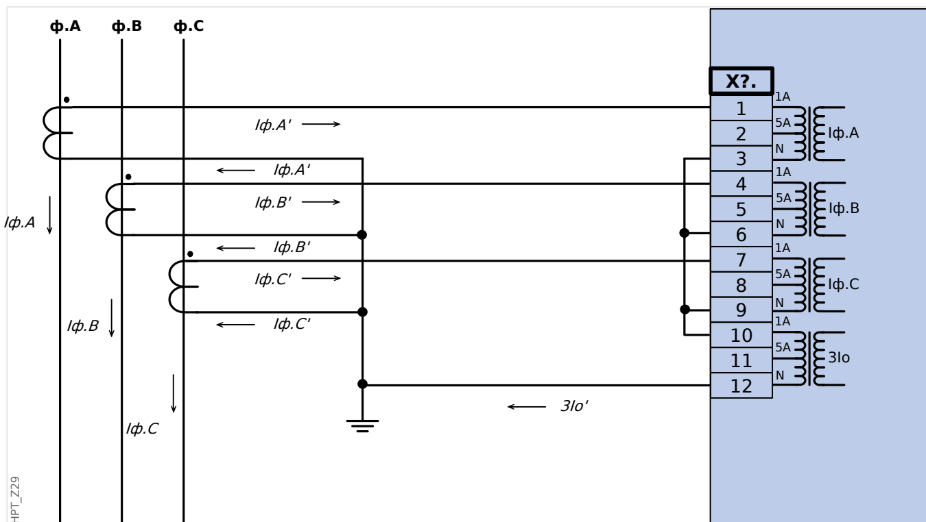
Рис. 22: Измерение фазных токов по схеме «полной» звезды; I n вторичн. = 1 А. Ток на землю, измеряемый через соединение по схеме Холмгриня 3I 0 .ном.втор. = 1 А.
