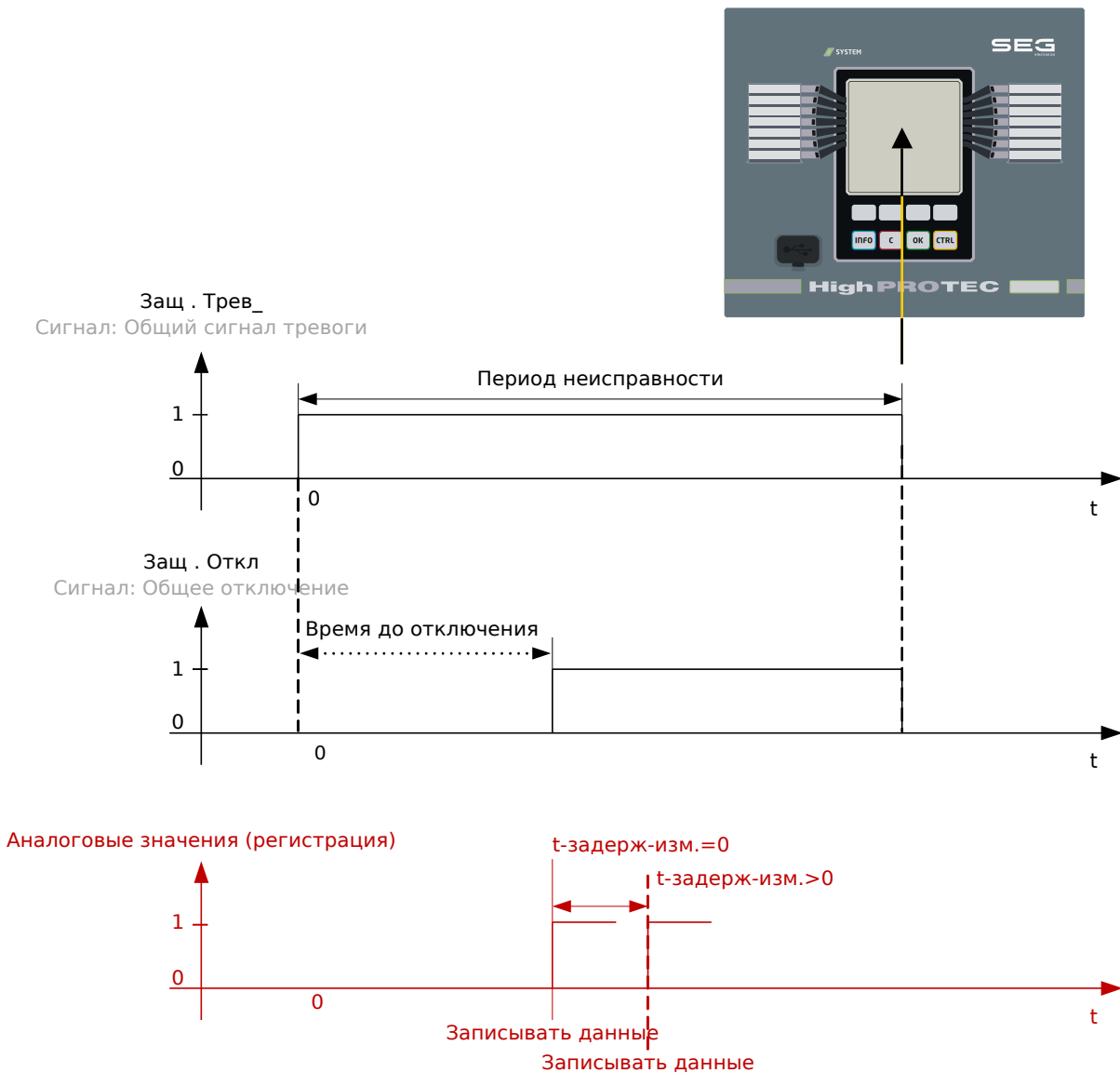
Рис. 79: Регистратор неисправностей: время и длительность.
