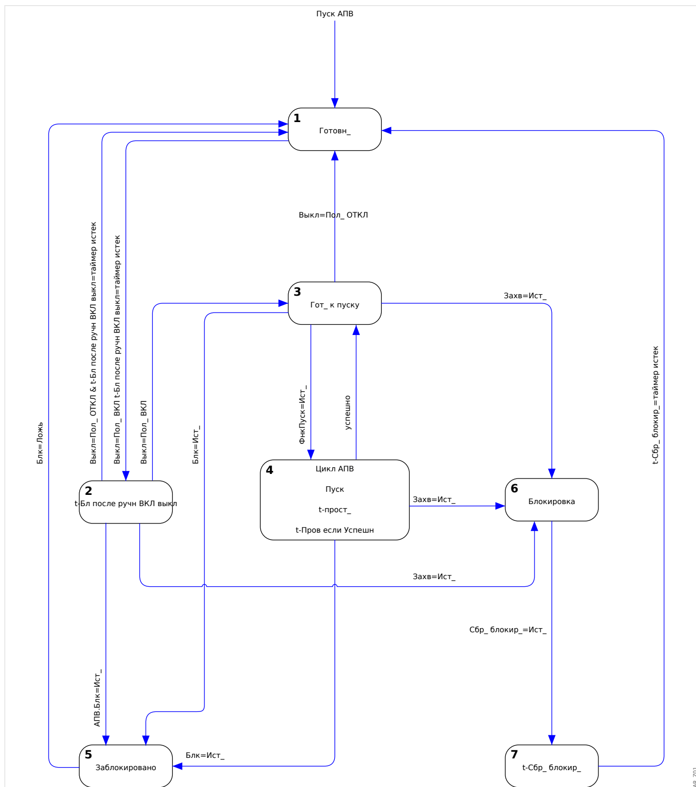
Рис. 56: Диаграмма переходов состояний.
