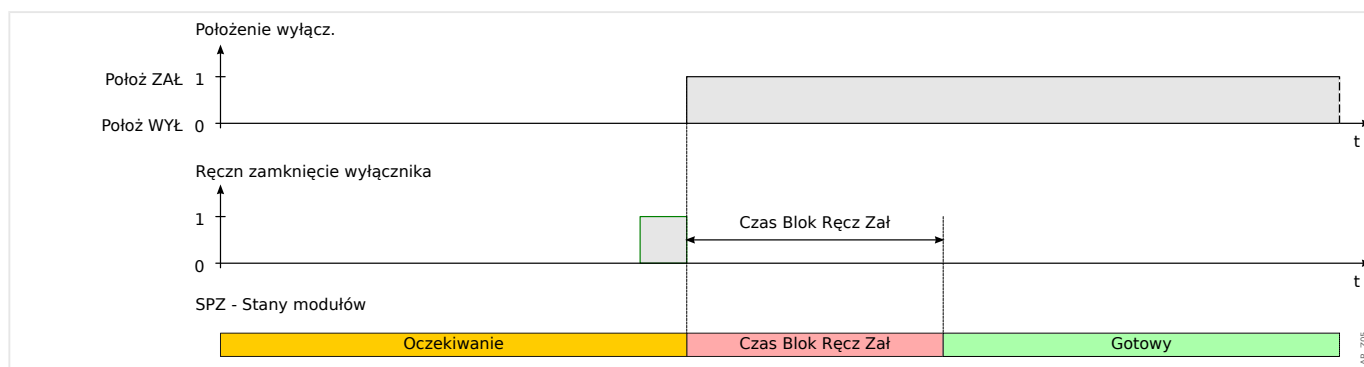
Rys. 60: Stany SPZ podczas ręcznego zamykania wyłącznika.
