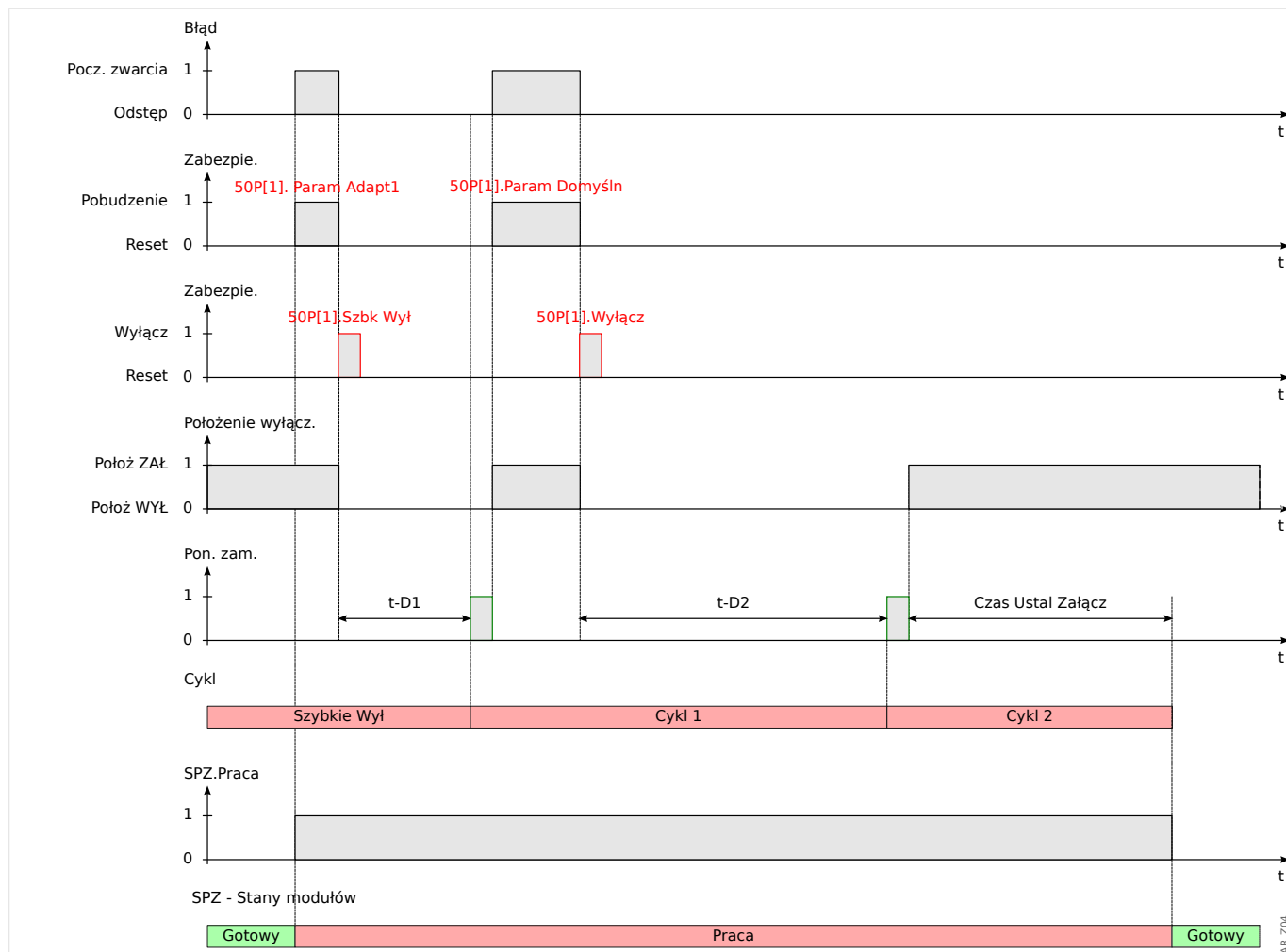
Rys. 59: Schemat czasów SPZ w przypadku udanego planu SPZ z 2 próbami i przyspieszeniem przy próbie wstępnej
