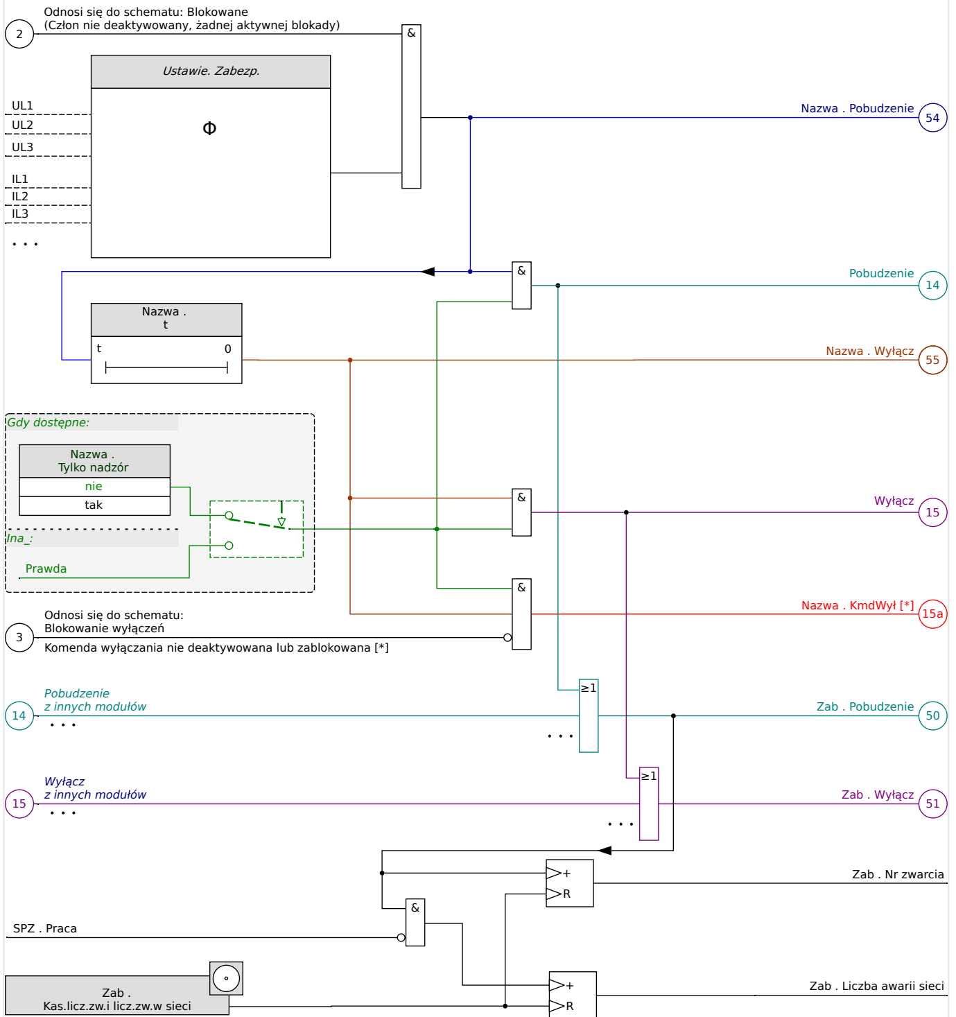
Rys. 43: Schemat ogólny działania każdego elementu zabezpieczającego HighPROTEC.
