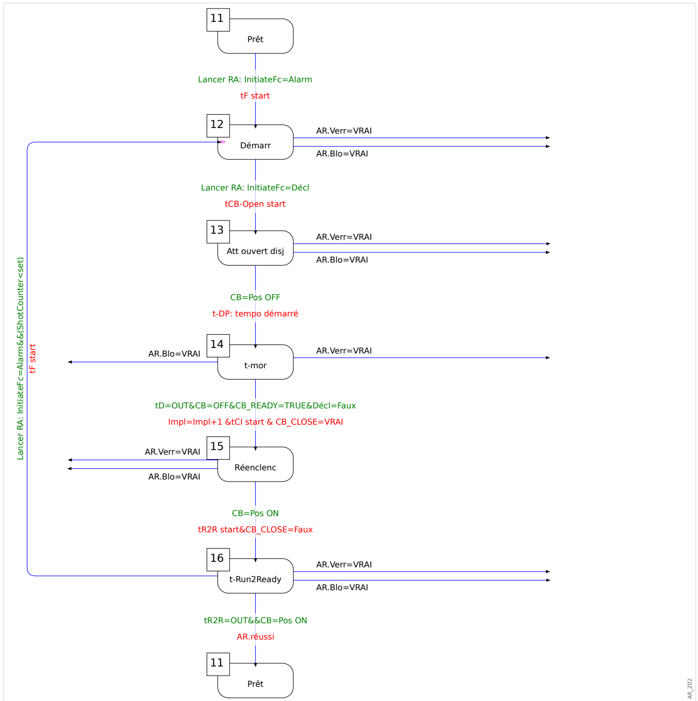
Fig. 57: Cycle d'exécution du AR (état 4).
