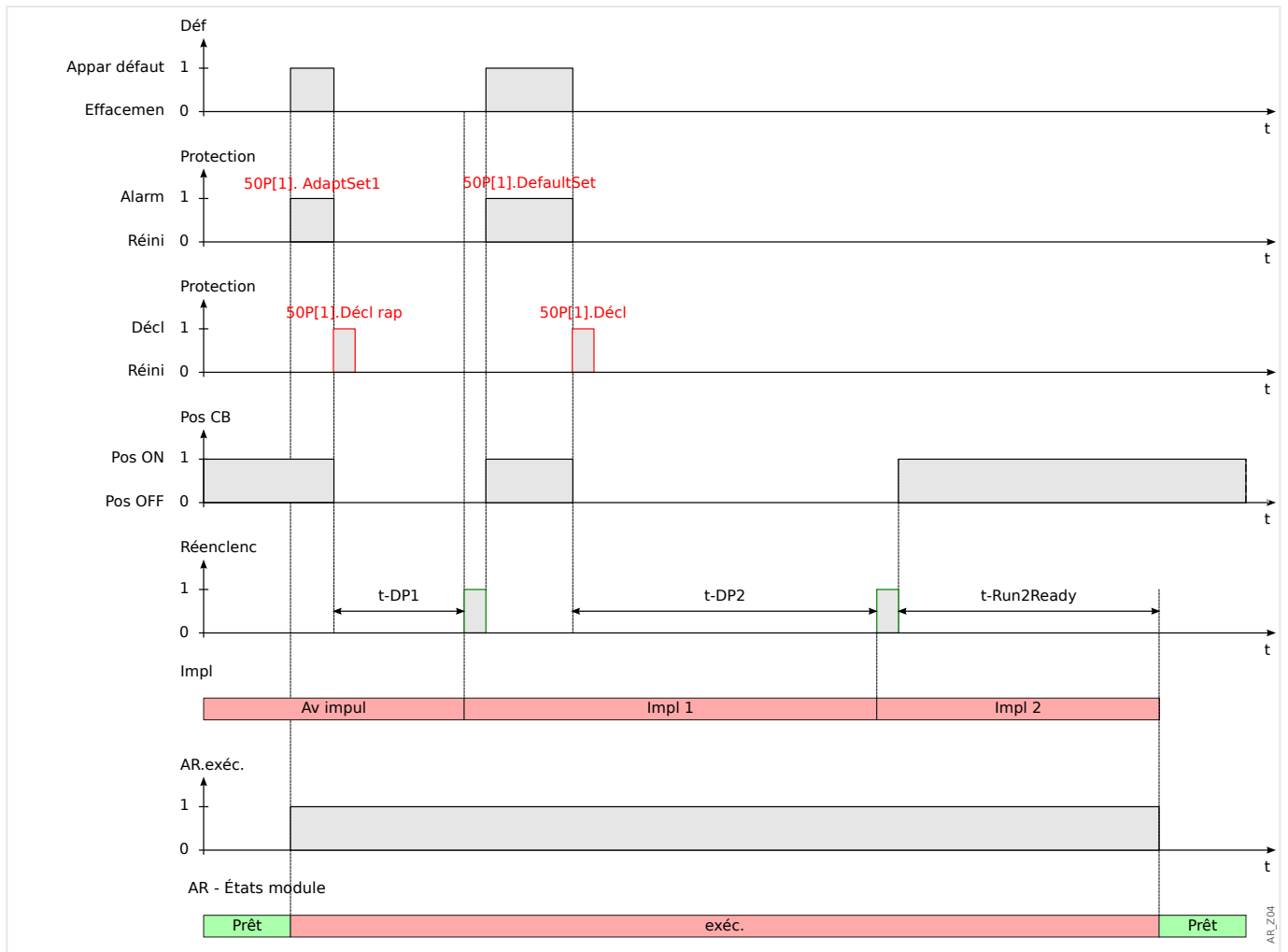
Fig. 59: Diagramme de temporisation de réenclenchement automatique pour un schéma de réenclenchement automatique à 2 impulsions réussi avec une accélération à la pré-impulsion.
