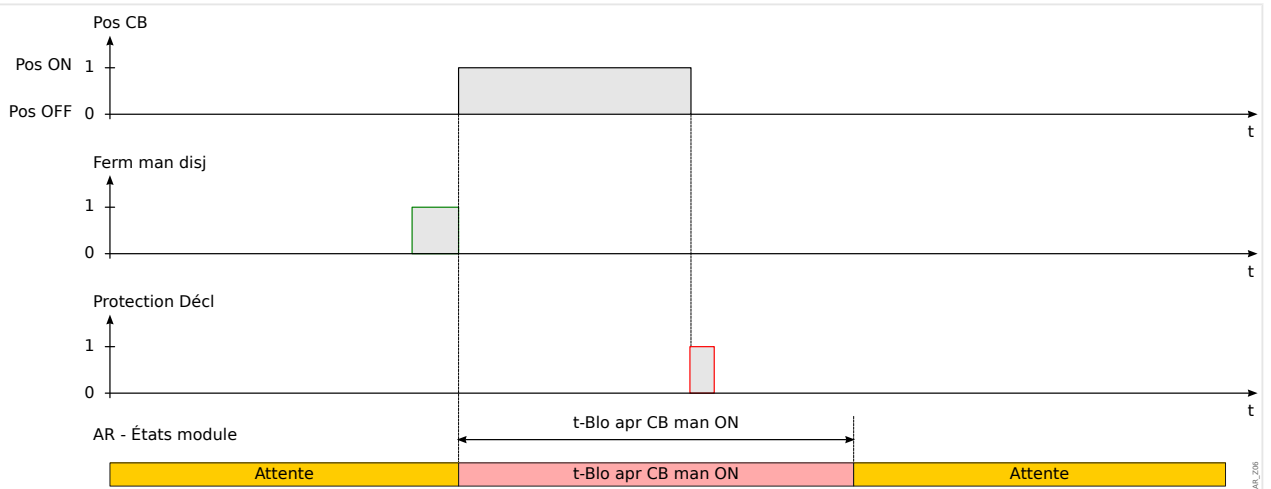
Fig. 61: Déclenchement de la protection pendant l'écoulement de la temporisation du blocage de fermeture manuelle.
