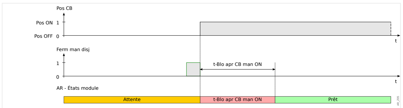
Fig. 60: États du réenclenchement automatique pendant la fermeture manuelle du disjoncteur.
