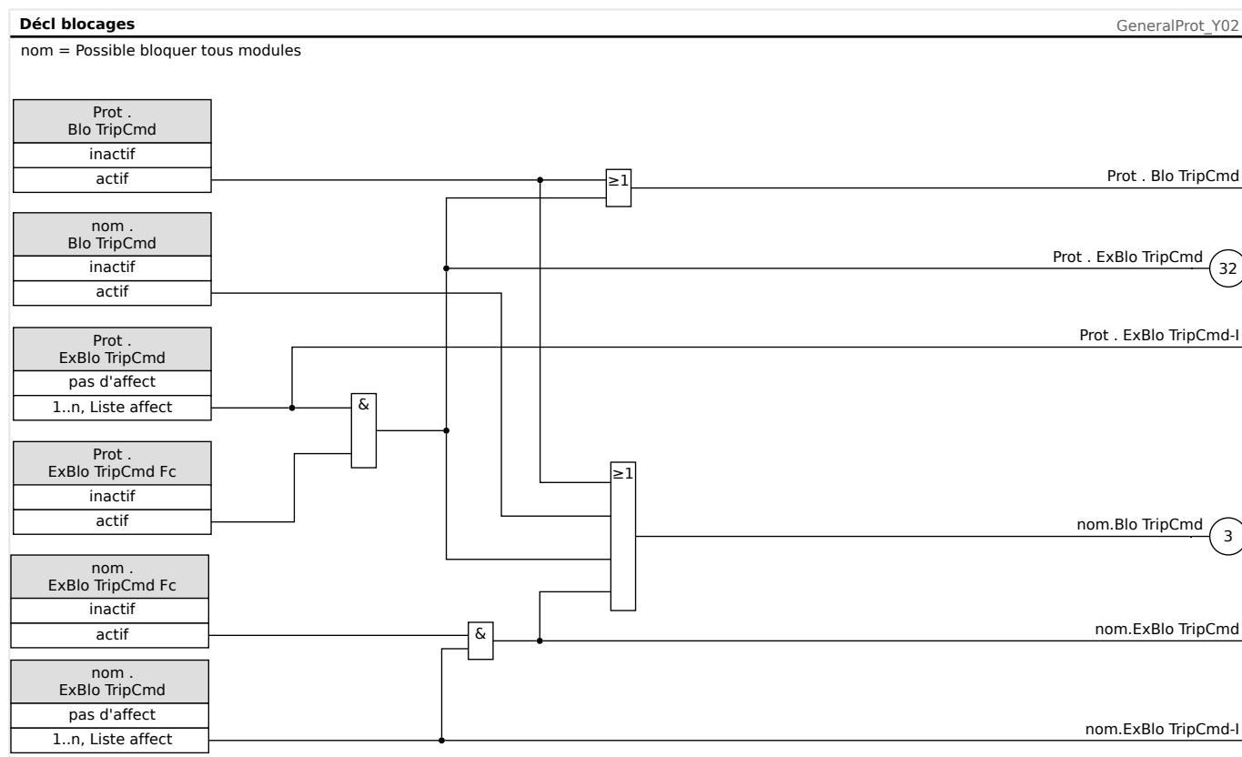
Fig. 44: Activation ou désactivation de la commande de déclenchement d'un module de protection
