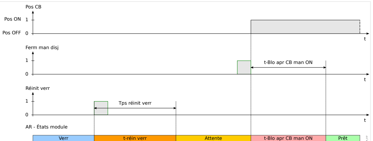
Fig. 62: Logique de réinitialisation du verrouillage du réenclenchement automatique si la réinitialisation du verrouillage se produit avant la fermeture du disjoncteur manuelle.
