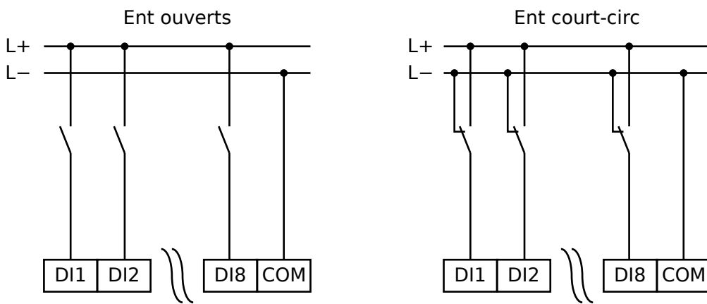
Fig. 88: État sécuritaire des entrées numériques
