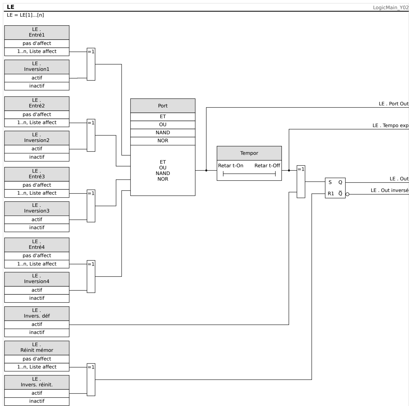
Fig. 81: Présentation détaillée - Diagramme logique global.
