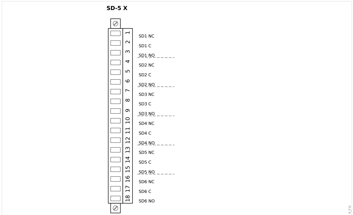
Fig. 13: RO-5 - Asignación de contactos
