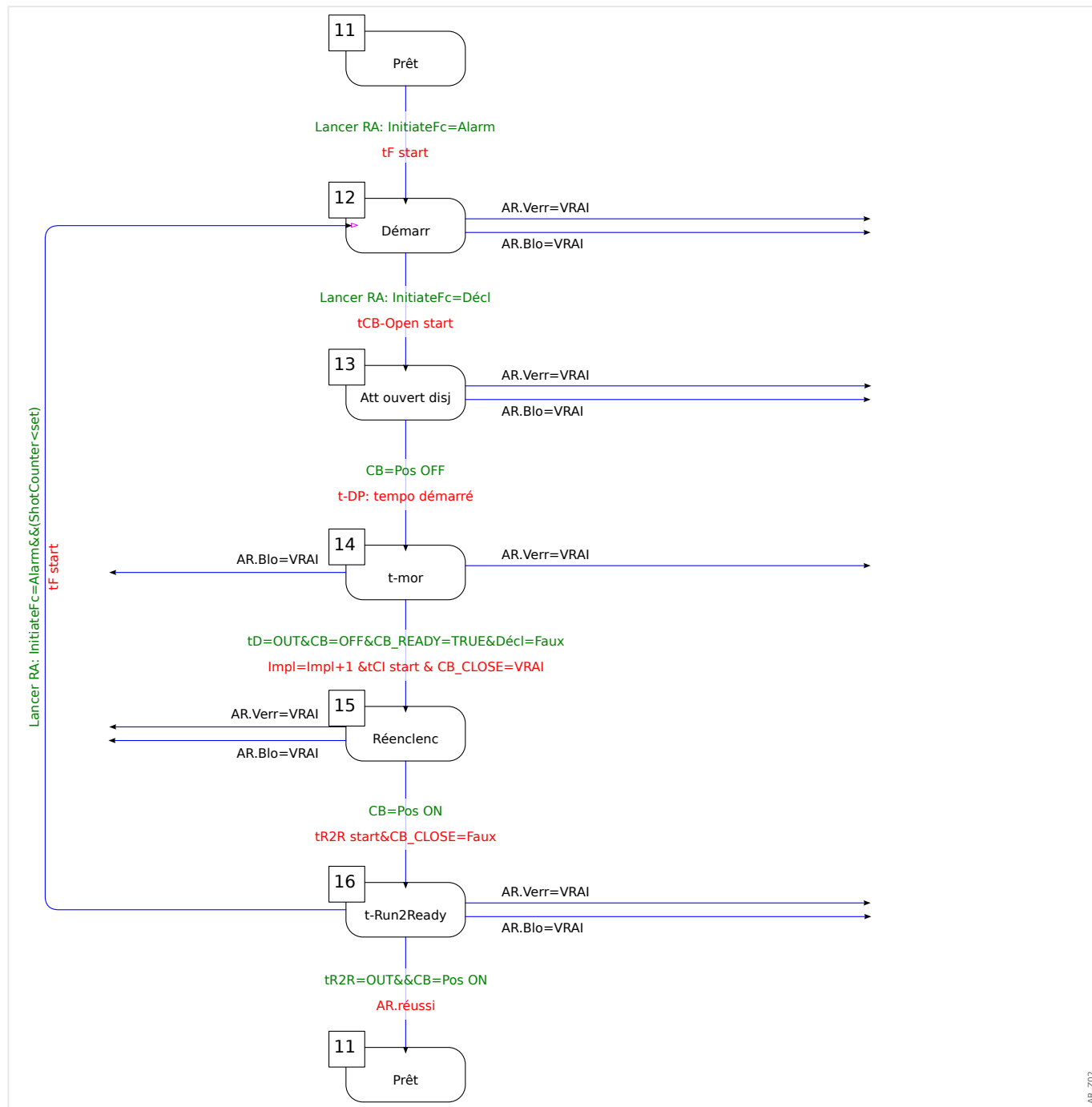
Fig. 48: Cycle d'exécution du AR (état 4).
