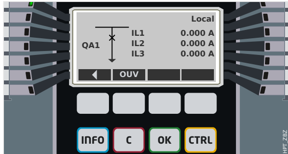
Fig. 60: Exemple de page de contrôle, avec le « disjoncteur » en position fermée.
