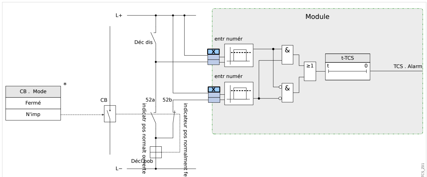
Fig. 57: Exemple de connexion : Surveillance du circuit de déclenchement avec de contacts auxiliaires de disjoncteur «Aux ON» (52a) et «Aux OFF» (52b).
