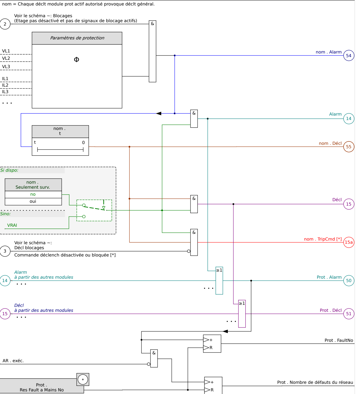
Fig. 42: Schéma de fonctionnalité des éléments de protection HighPROTEC.
