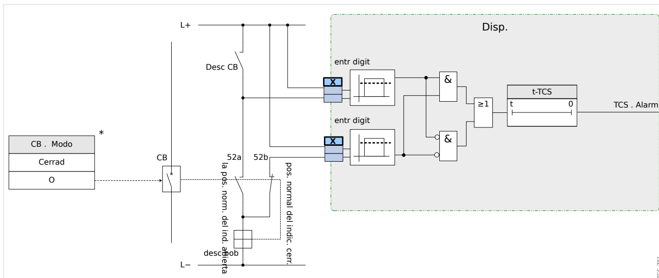
Fig. 57: Ejemplo de conexión: Supervisión del circuito de desconexión con dos contactos auxiliares CB »Aux ON« (52a) and »Aux OFF« (52b).
