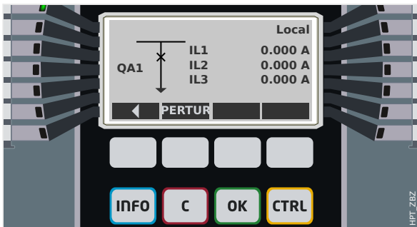
Fig. 60: Ejemplo de página de control, con el circuito en posición cerrada.
