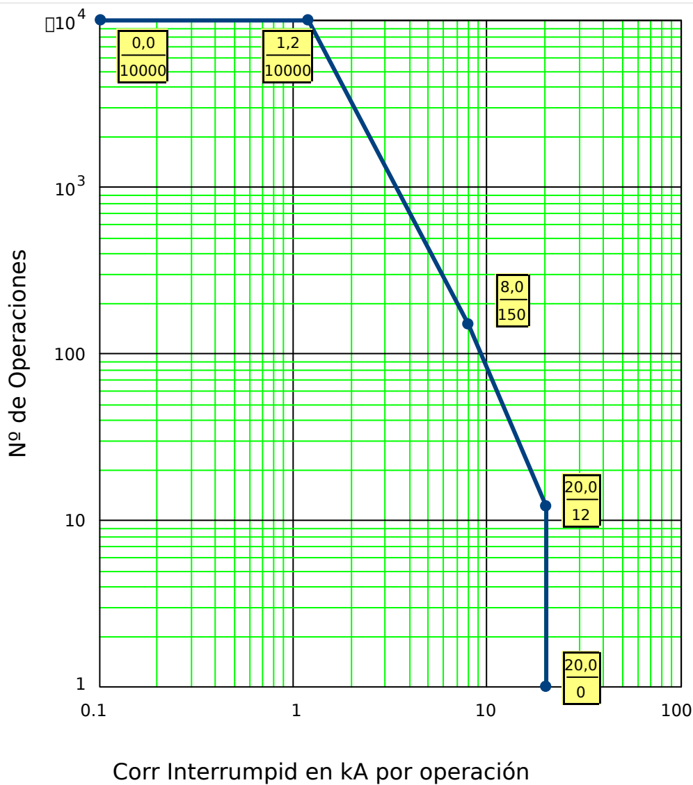
Fig. 65: Curva Mantenim Interruptor para Interrupt Circuito típico 25kV
