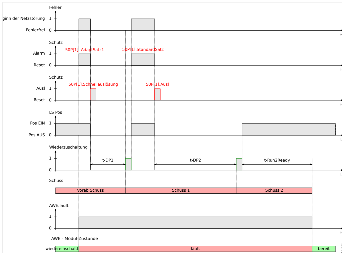
Abb. 50: Zweischüssige, erfolgreiche Wiedereinschaltung mit Schnellauslösung (Prä-Schuss).
