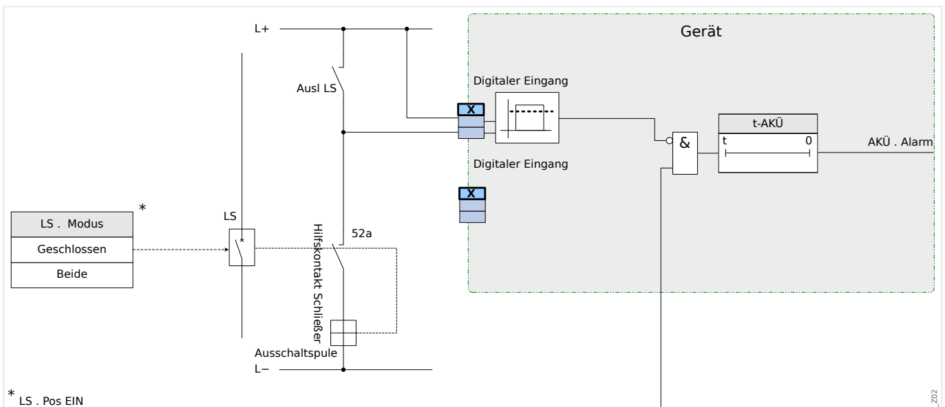
Abb. 58: Anschlussbeispiel: Auslösekreisüberwachung mit einem Hilfskontakt »Hiko EIN« (52a).
