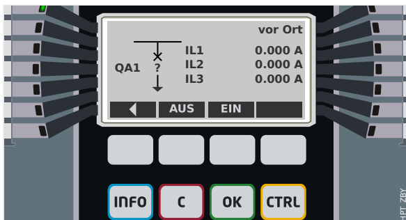
Abb. 61: Beispiel einer Steuer-Seite mit „Leistungsschalter“ in Störstellung (bzw. unplausiblem Zustand).
