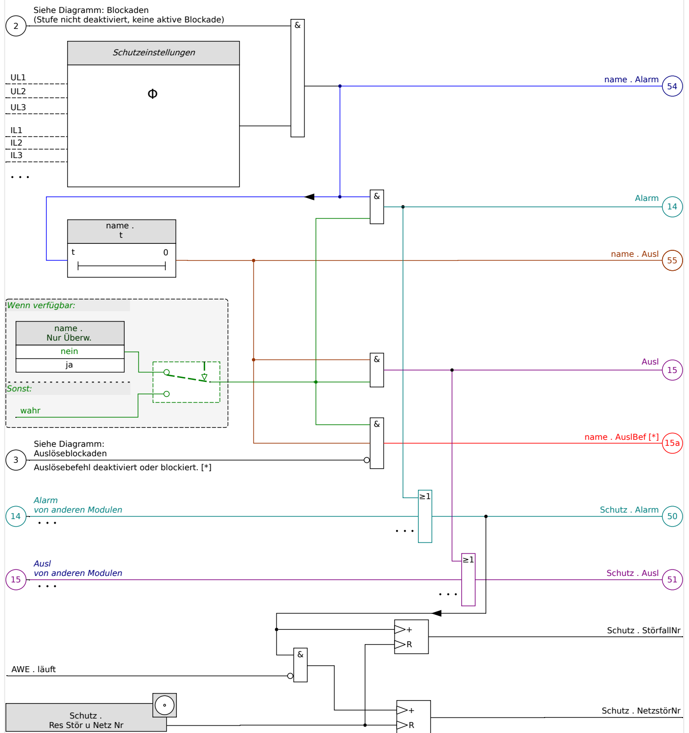
Abb. 42: Grobe Skizze der Funktionalität einer HighPROTEC-Schutzfunktion.
