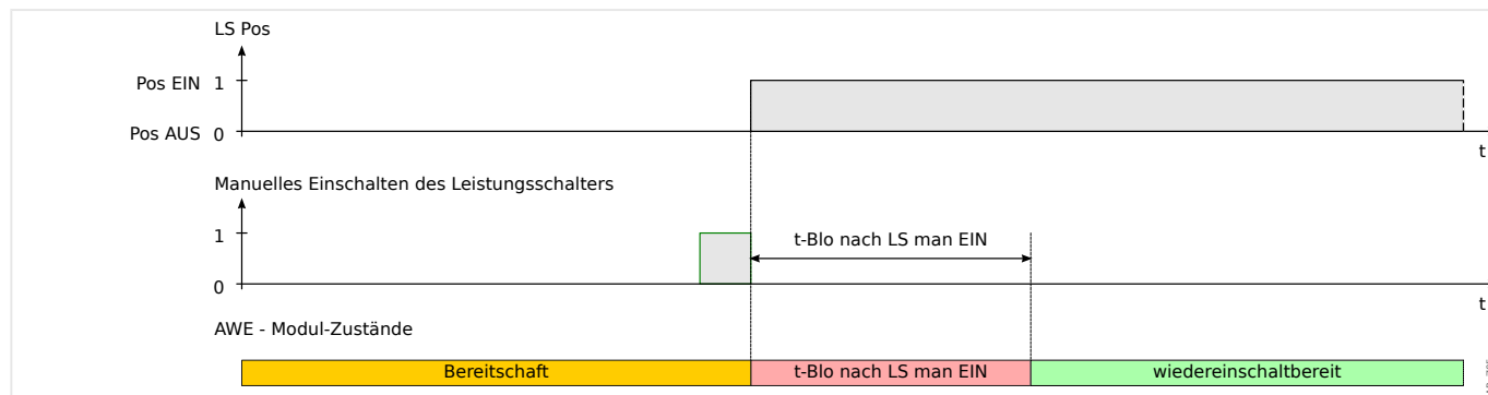
Abb. 51: AWE-Zustände beim manuellen Einschalten des Leistungsschalters.
