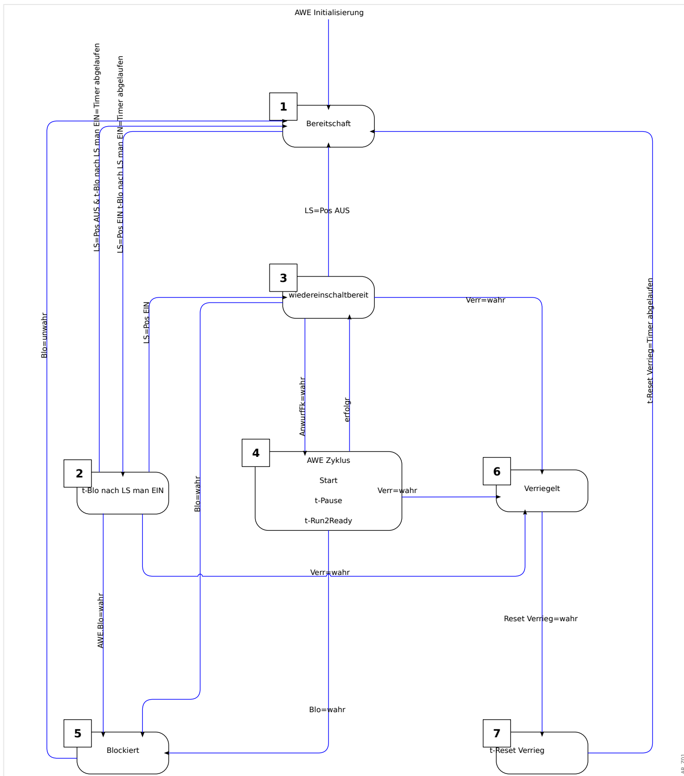
Abb. 47: Zustandsdiagramm.
