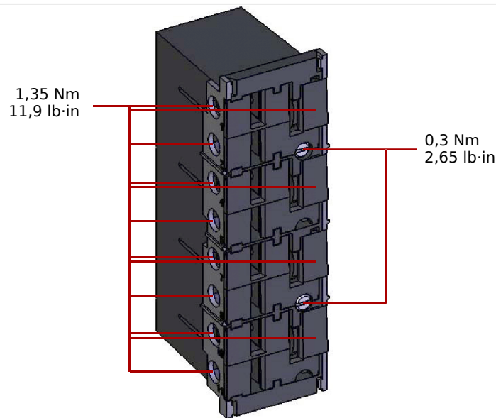
Abb. 80: Steckverbinder mit integrierten Kurzschließern (konventionelle Stromeingänge)
