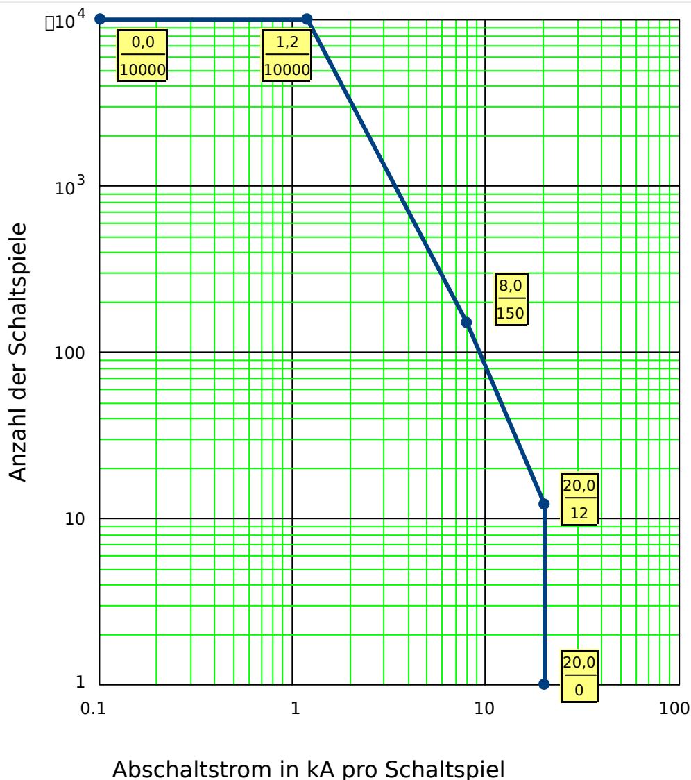
Abb. 65: Wartungskurve für einen typischen 25 kV Leistungsschalter
