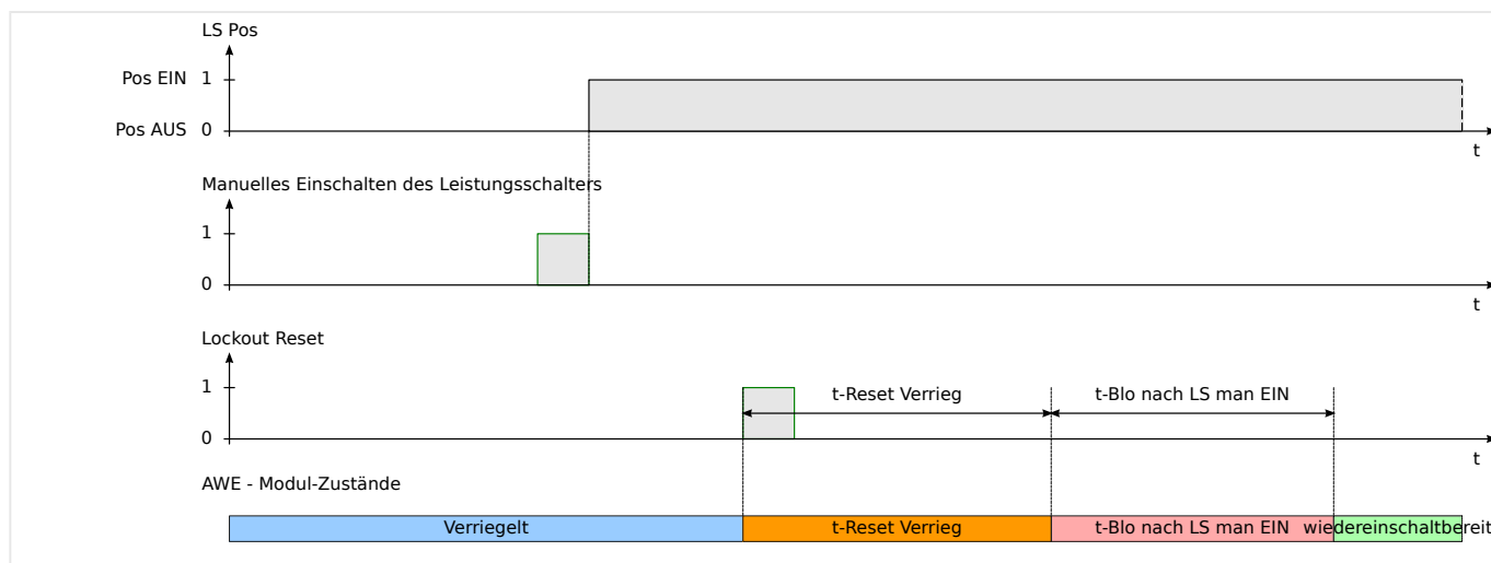
Abb. 54: AWE-Verriegelungs-Rücksetzlogik mit Rücksetzkommando nach dem manuellem Einschalten des Leistungsschalters.
