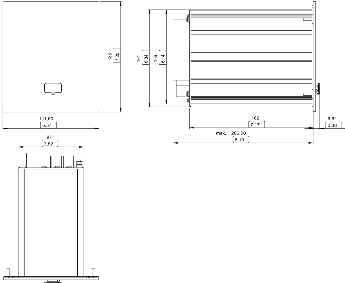
3-Seiten-Ansicht B1-Gehäuse (8-Tasten). (Alle Angaben in mm, Maße in eckigen Klammern in Zoll.)
