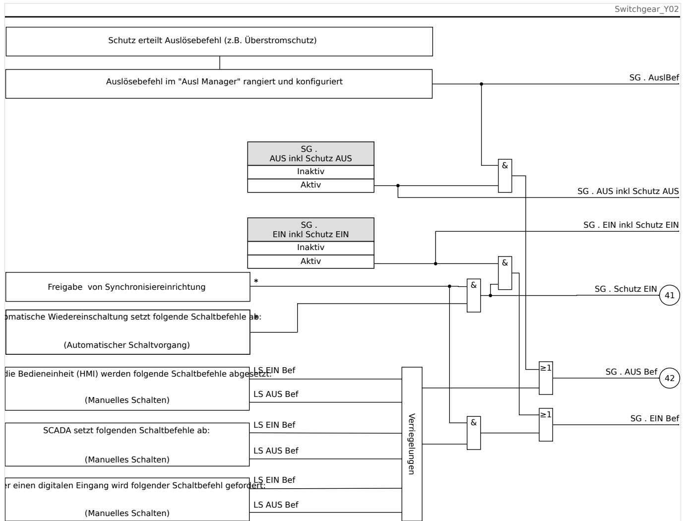
Abb. 91: Verriegelungen. (Für die mit „*“ markierten Teile gilt: Verfügbarkeit hängt von der bestellten Gerätevariante ab.)
