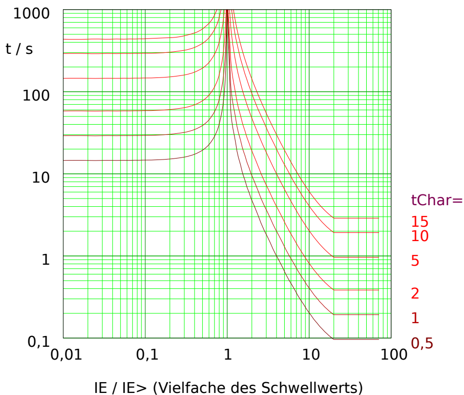
Abb. 65: EINV: Rückfallverzögerung (linke Hälfte, IE < I_{E>} ) und Auslöseverzögerung (rechte Hälfte, IE > I_{E>} ), Beispieldiagramm für I_{max} = 20 \cdot I_{E>} .
