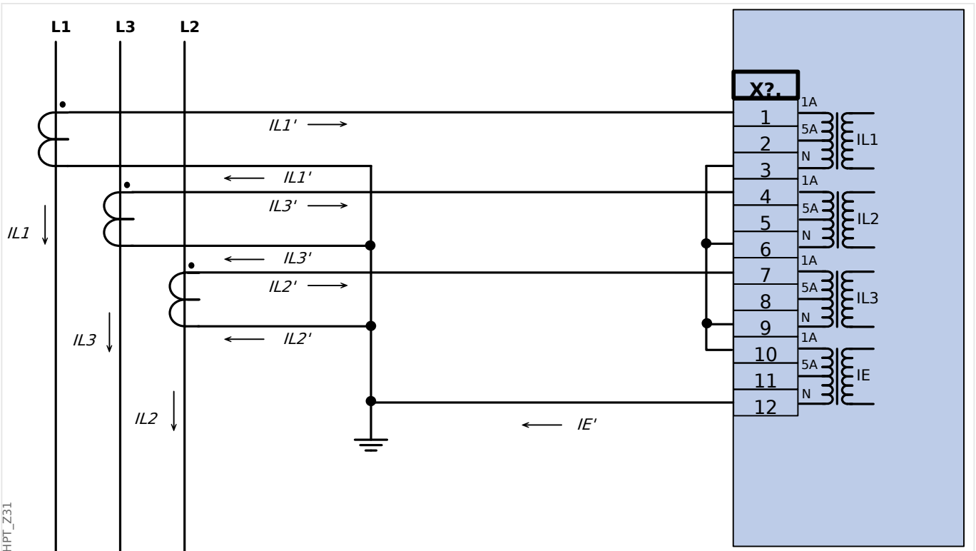
Abb. 24: Dreiphasiger Stromwandleranschluss; In sekundär = 1 A. Erdstromerfassung über Holmgrenschtaltung I_{E'n} sekundär = 1 A.
