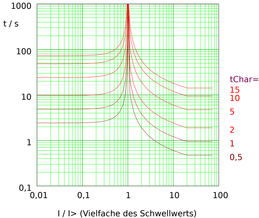
Abb. 51: MINV: Rückfallverzögerung (linke Hälfte, I < I_{>} ) und Auslöseverzögerung (rechte Hälfte, I > I_{>} ), Beispieldiagramm für I_{max} = 20 \cdot I_{>} .
