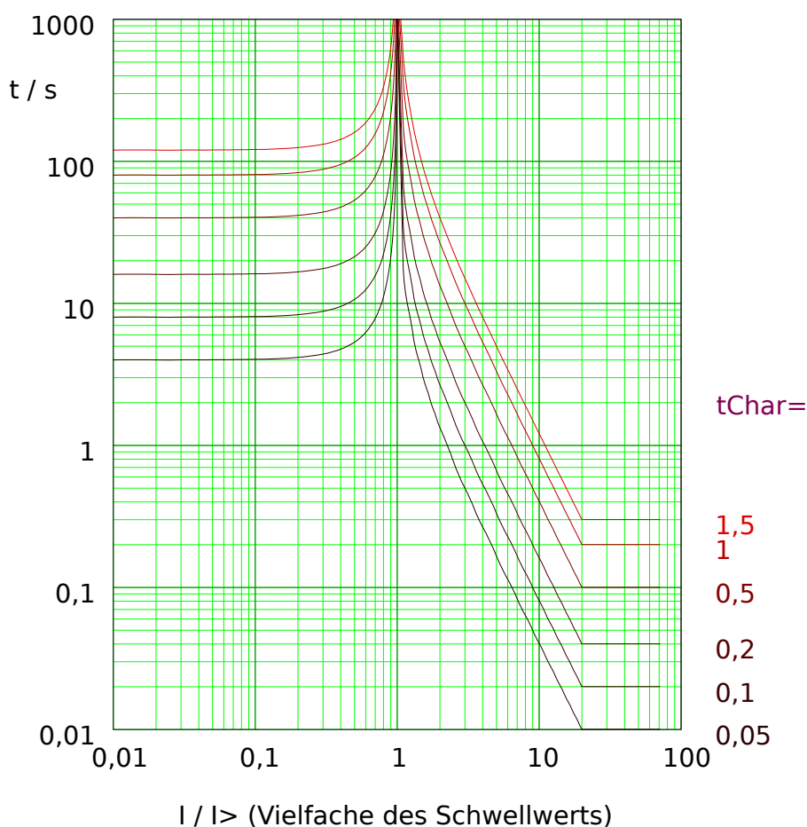
Abb. 48: EINV: Rückfallverzögerung (linke Hälfte, I < I_{>} ) und Auslöseverzögerung (rechte Hälfte, I > I_{>} ), Beispieldiagramm für I_{max} = 20 \cdot I_{>} .
