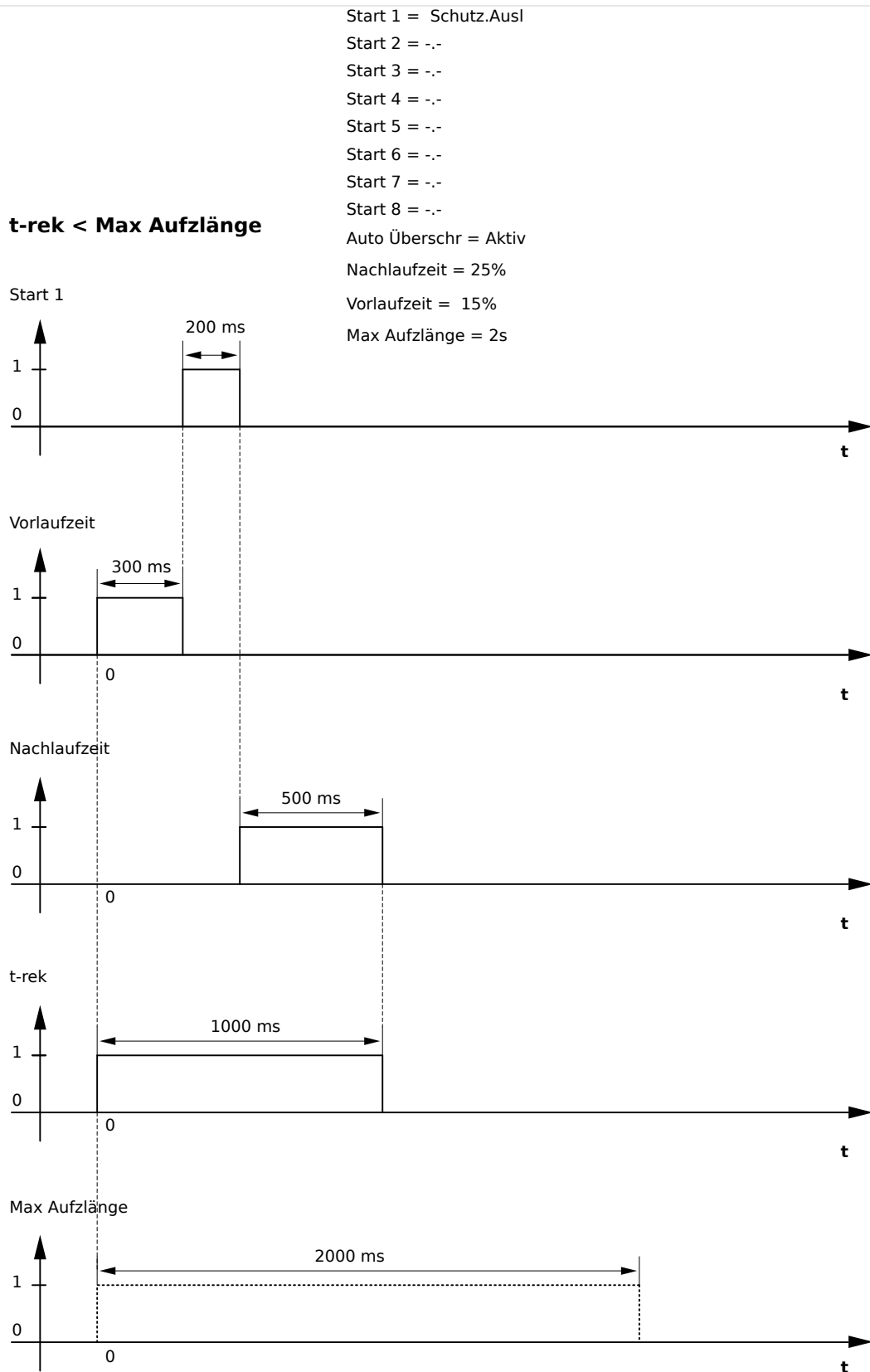
Abb. 97: Beispiel II Störschreiber-Ablaufdiagramm
