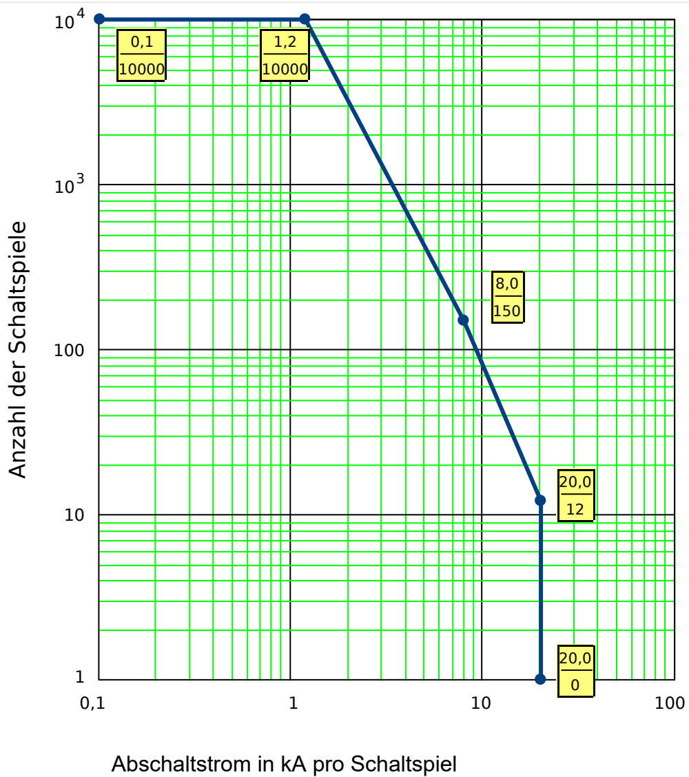
Abb. 93: Wartungskurve für einen typischen 25 kV Leistungsschalter
