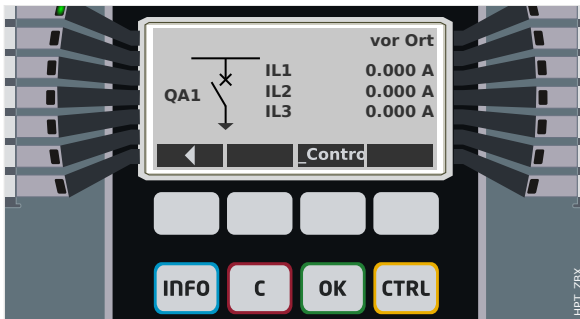
Abb. 90: Beispiel einer Steuer-Seite mit geöffnetem „Leistungsschalter“.
