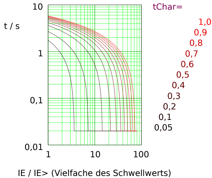
Abb. 66: RXIDG: Auslöseverzögerung, IE > IE_{>} .
