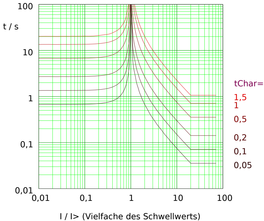
Abb. 47: VINV: Rückfallverzögerung (linke Hälfte, I < I_{>} ) und Auslöseverzögerung (rechte Hälfte, I > I_{>} ), Beispieldiagramm für I_{max} = 20 \cdot I_{>} .
