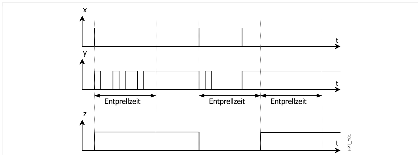
Abb. 39: Entprell-Mechanismus des MRI4.
