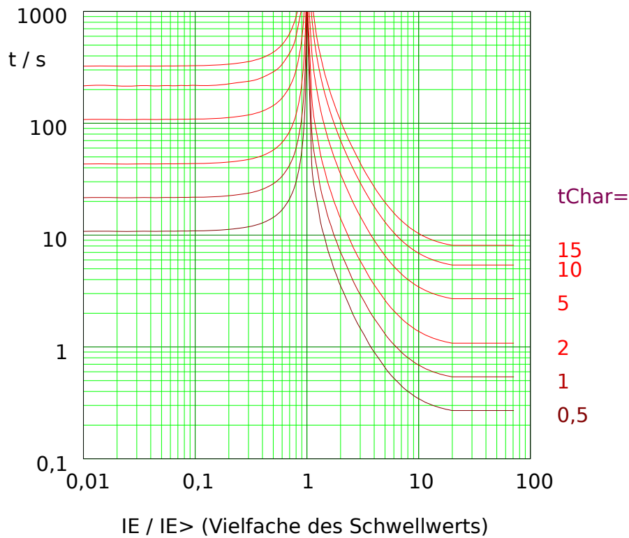
Abb. 64: VINV: Rückfallverzögerung (linke Hälfte, IE < I_{E>} ) und Auslöseverzögerung (rechte Hälfte, IE > I_{E>} ), Beispieldiagramm für I_{max} = 20 \cdot I_{E>} .
