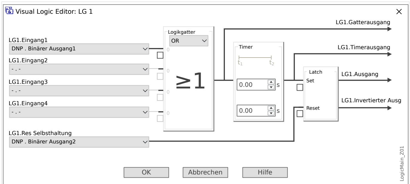
Abb. 41: Einstellbeispiel aus Smart view, um einen statischen Zustand aus einem DNP-Ausgangssignal zu erhalten.
