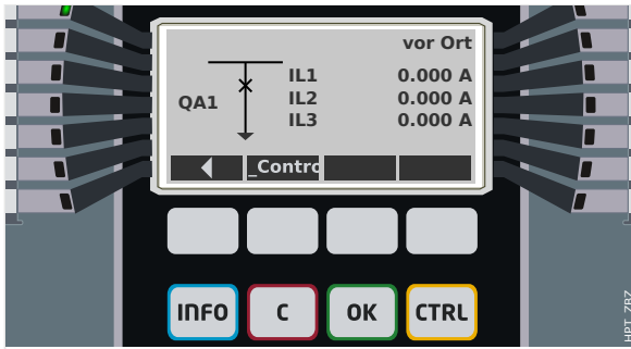
Abb. 88: Beispiel einer Steuer-Seite mit geschlossenem „Leistungsschalter“.
