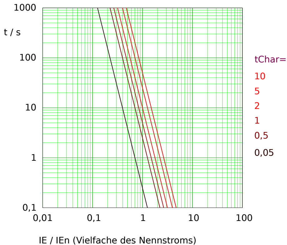
Abb. 70: Auslösekurve „I4T“, wobei nur der Bereich IE > I_{E>} jeweils anwendbar ist. Beispieldiagramm für gemessenen (nicht empfindlichen) Erdstrom.
