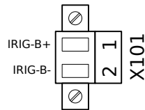
Abb. 28: IRIG-B00X - Elektromechanische Zuordnung.
