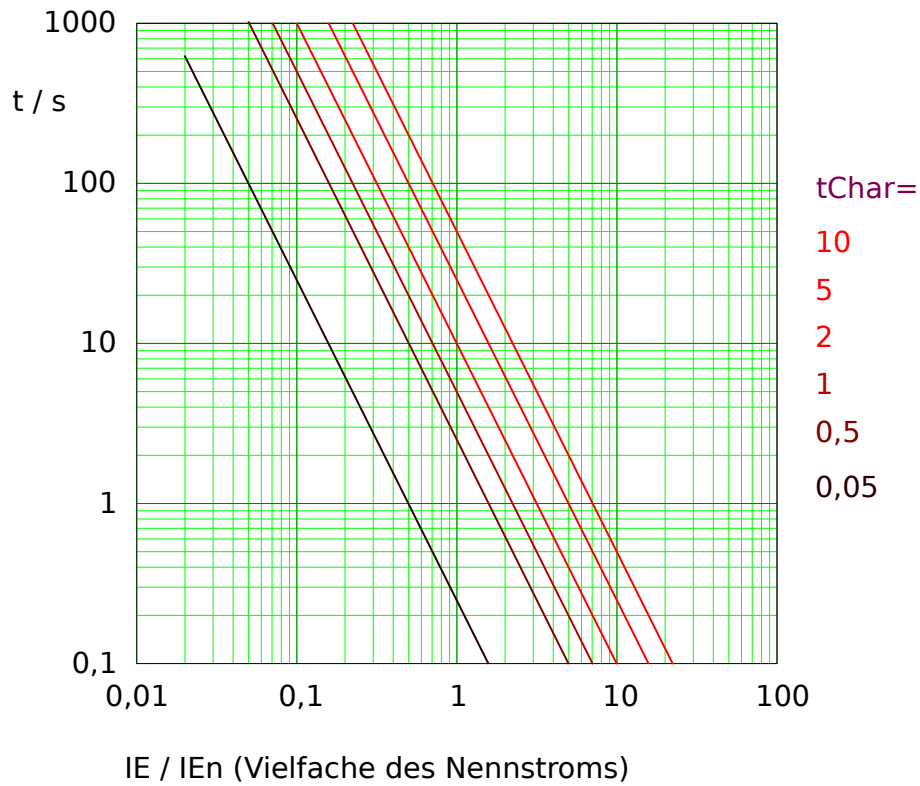
Abb. 69: Auslösekurve „I2T“, wobei nur der Bereich I_E > I_{E>} jeweils anwendbar ist. Beispieldiagramm für gemessenen (nicht empfindlichen) Erdstrom.
