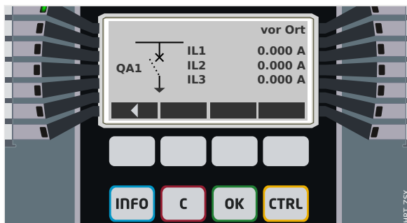
Abb. 87: Beispiel einer Steuer-Seite mit „Leistungsschalter“ in Zwischenposition).
