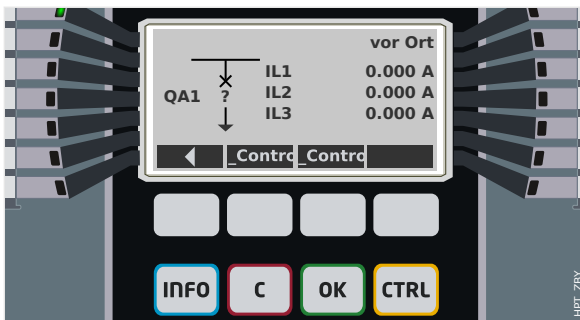
Abb. 89: Beispiel einer Steuer-Seite mit „Leistungsschalter“ in Störstellung (bzw. unplausiblem Zustand).
