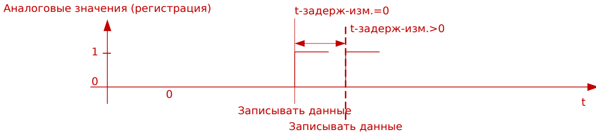
Рис. 79: Регистратор неисправностей: время и длительность.
