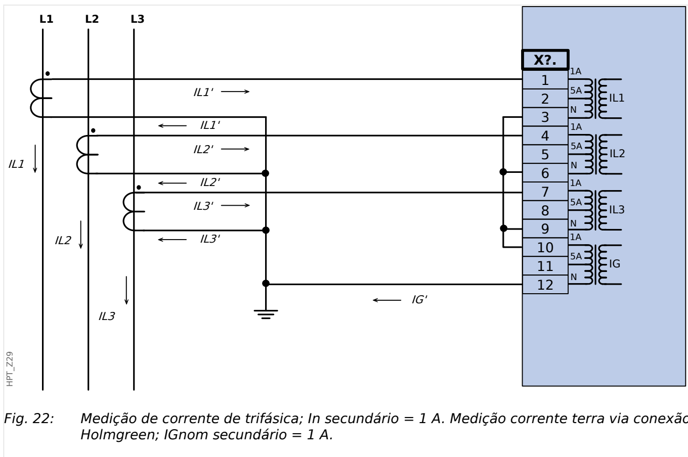
Fig. 21: Medição de corrente de trifásica; In secundário = 5 A. Medição corrente terra via conexão Holmgreen; IGnom secundário = 5 A.
