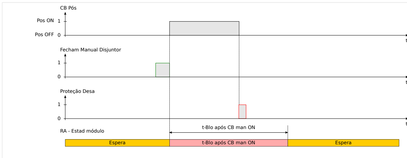
Fig. 61: Disparo de proteção enquanto o tempo de bloqueio de fechamento manual está cronometrando.
