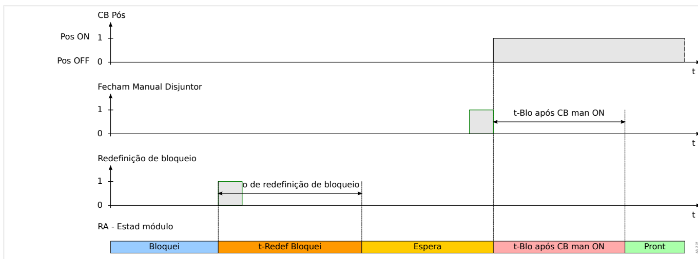
Fig. 62: A lógica de reinicialização de travamento no caso do reinício do travamento vir antes do fechamento manual do disjuntor
