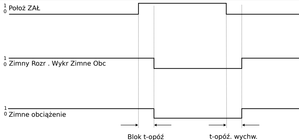
Rys. 64: Przykładowy tryb: Położenie wyłącznika.
