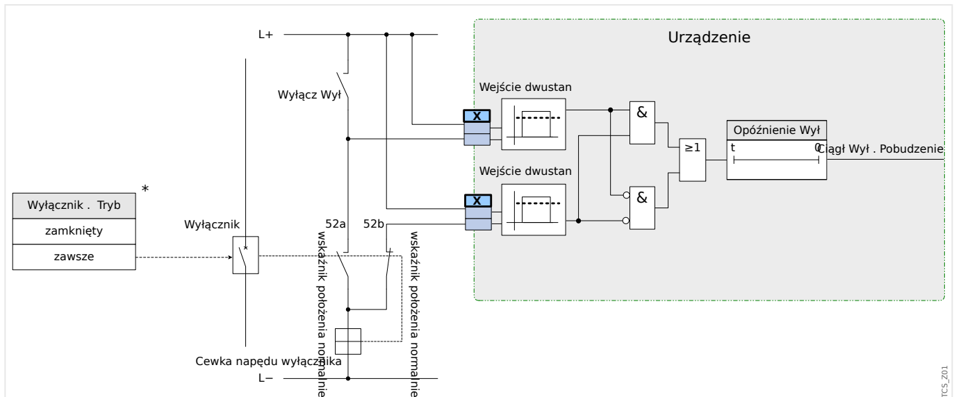
Rys. 66: Przykład okablowania: Układ kontroli ciągłości obwodów wyłącznika z dwoma stykami pomocniczymi wyłącznika „Położ ZAŁ” (52a) i „Położ WYŁ” (52b).
