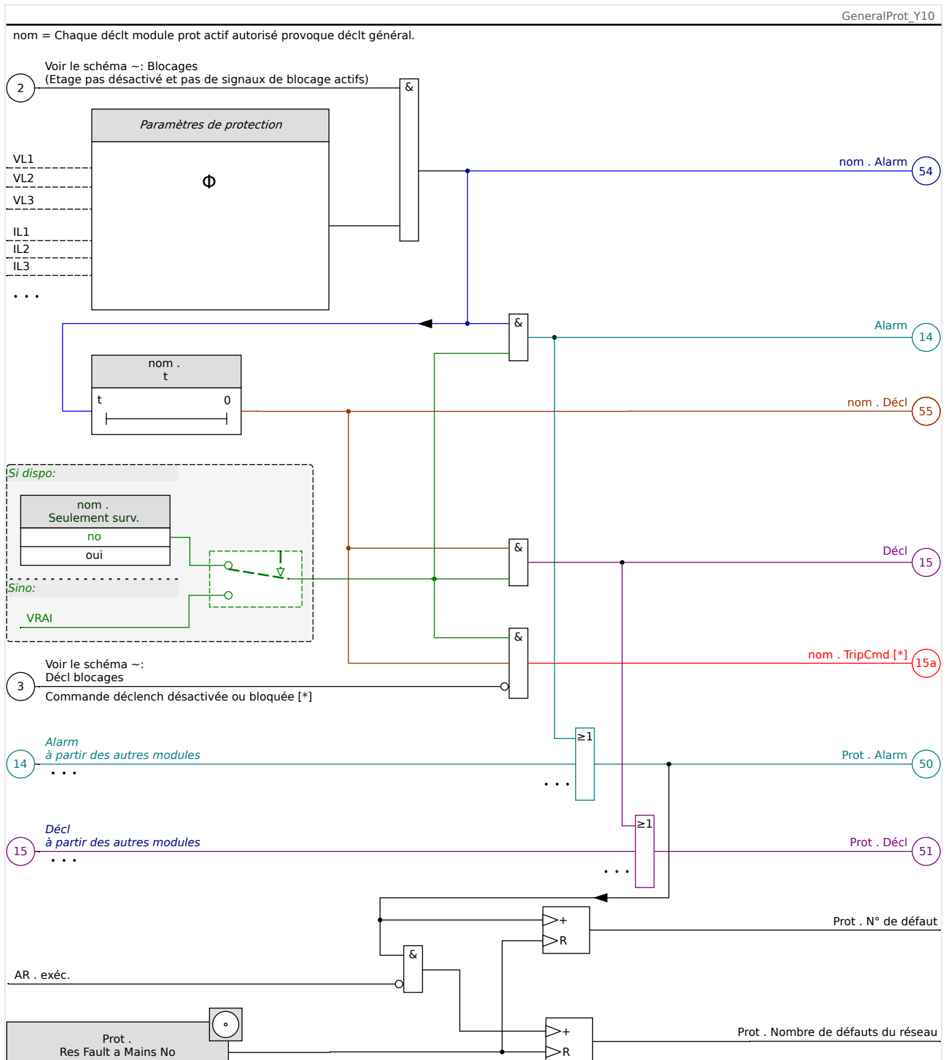
Fig. 43: Schéma de fonctionnalité des éléments de protection HighPROTEC.
