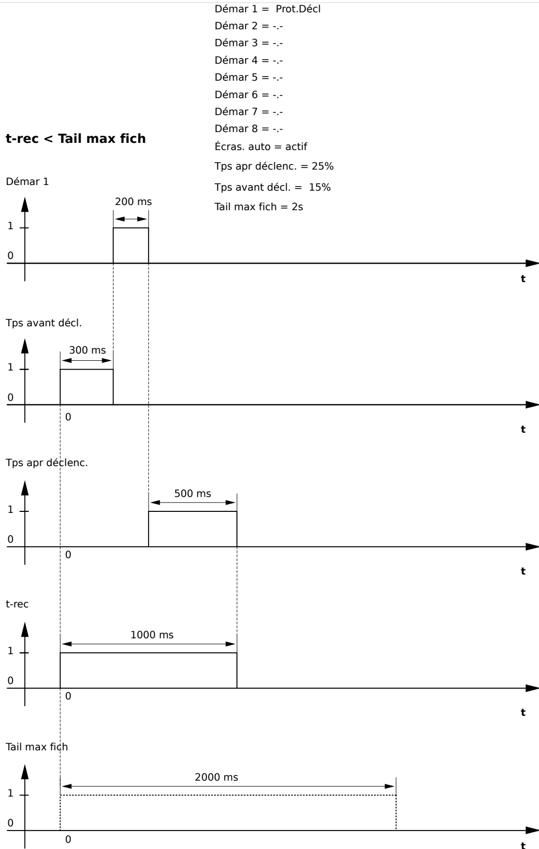
Fig. 78: Exemple de diagramme des temps de l'enregistreur de perturbations II
