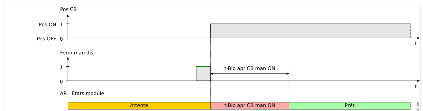
Fig. 60: États du réenclenchement automatique pendant la fermeture manuelle du disjoncteur.
