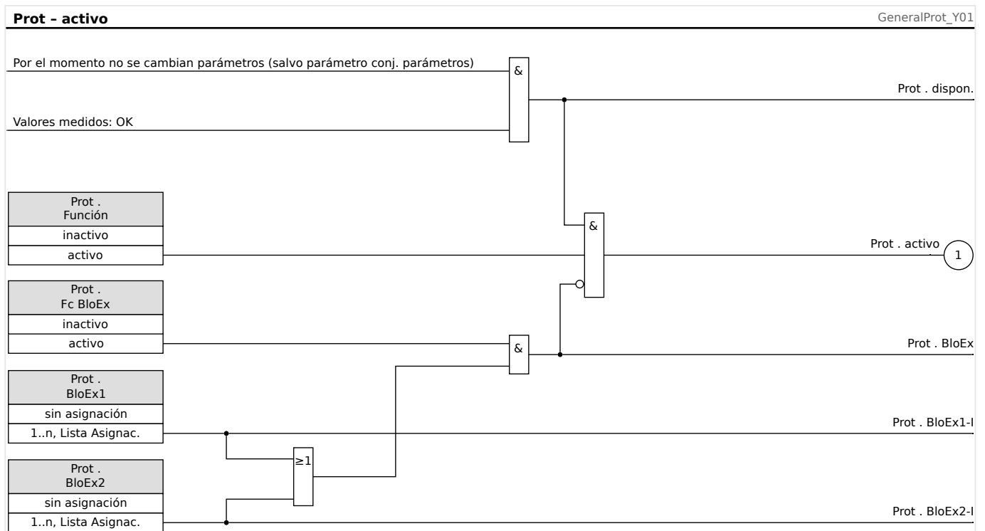
Fig. 42: Disponibilidad del módulo de protección general
