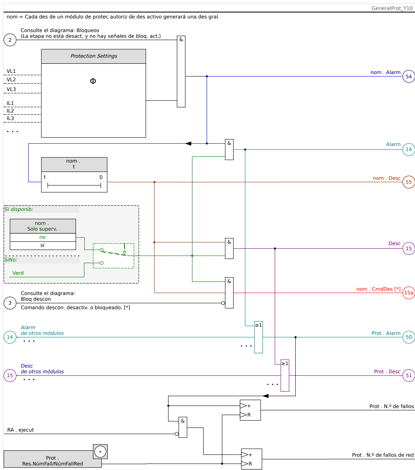
Fig. 43: Descripción a grandes rasgos de la funcionalidad de cualquier elemento de protección de HighPROTEC.
