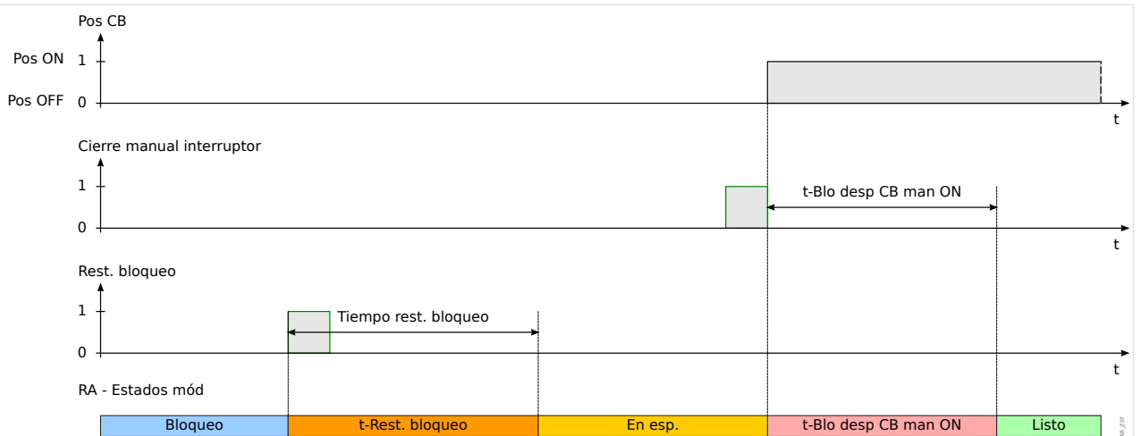
Fig. 62: Lógica de reinicio de bloqueo de AR en caso de que el reinicio de bloqueo llegue antes de que se cierre el interruptor manualmente.
