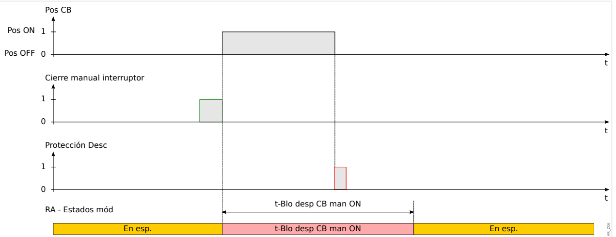
Fig. 61: Desconexión de protección mientras transcurre el tiempo de bloqueo de cierre manual.
