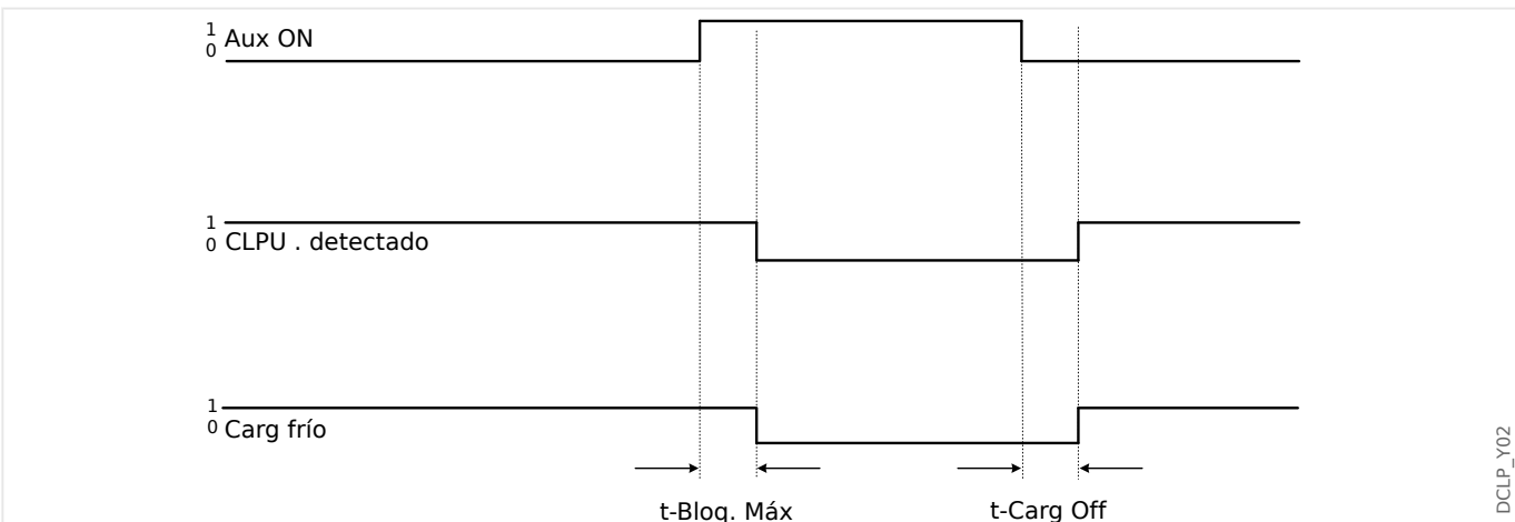
Fig. 64: Modo de ejemplo: Posición de interruptor.
