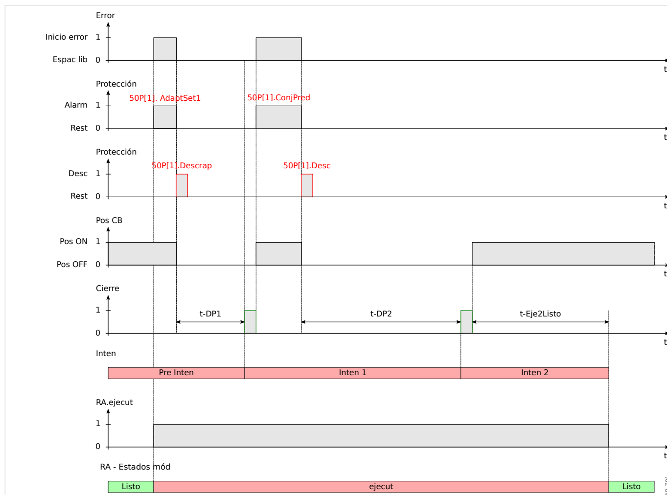
Fig. 59: Diagrama de tiempo de reconexión automática para el esquema de reconexión automática de dos intentos successful (correctos) con aceleración en un intento previo.
