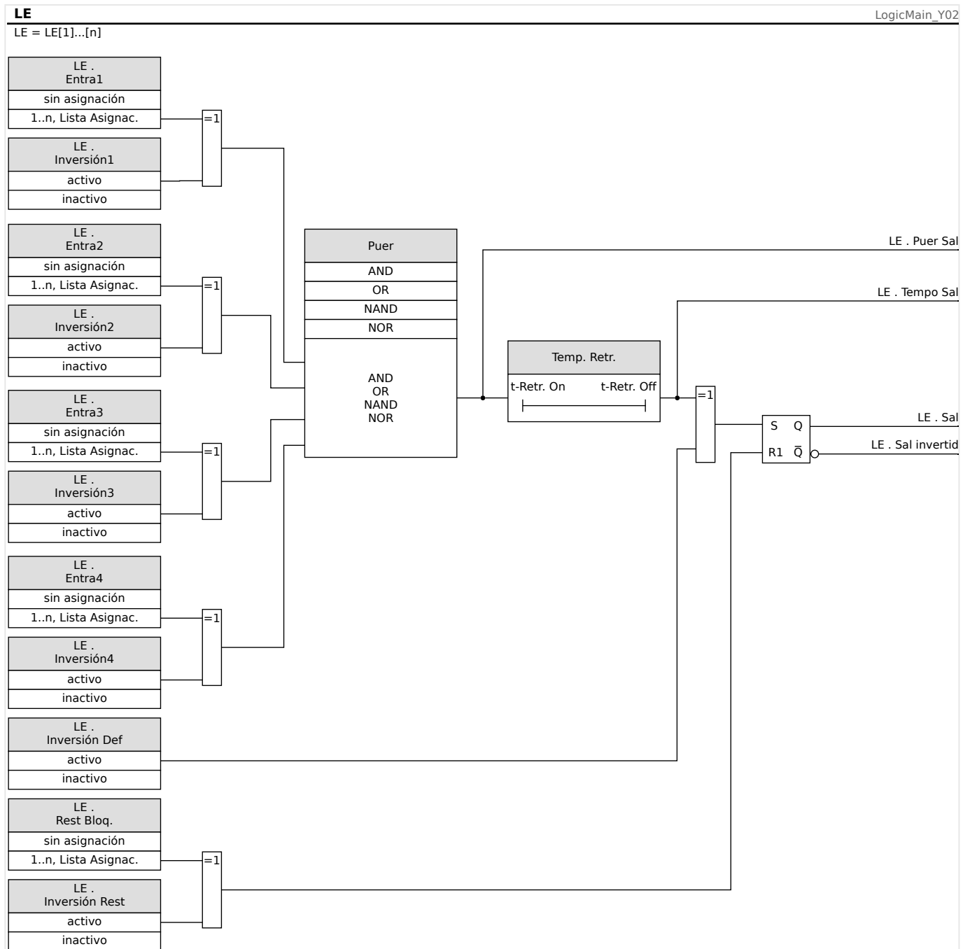
Fig. 81: Descripción detallada - Diagrama de lógica general.
