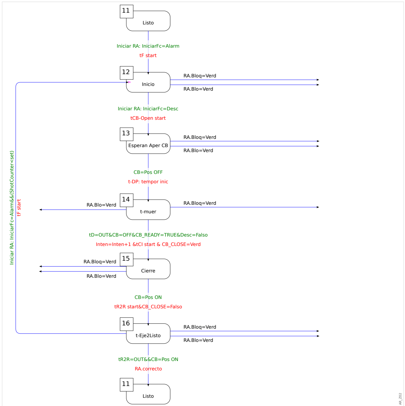
Fig. 57: Ciclo de ejecución de RA (estado 4).
