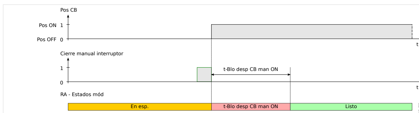
Fig. 60: Estados de reconexión automática durante el cierre manual del interruptor.
