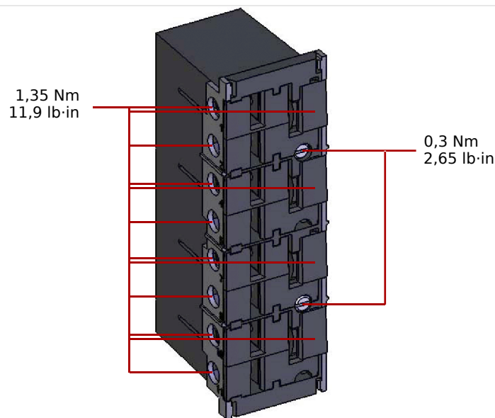
Рис. 80: Штепсельные соединения со встроенными закорачивающими перемычками (стандартные токовые входы)
