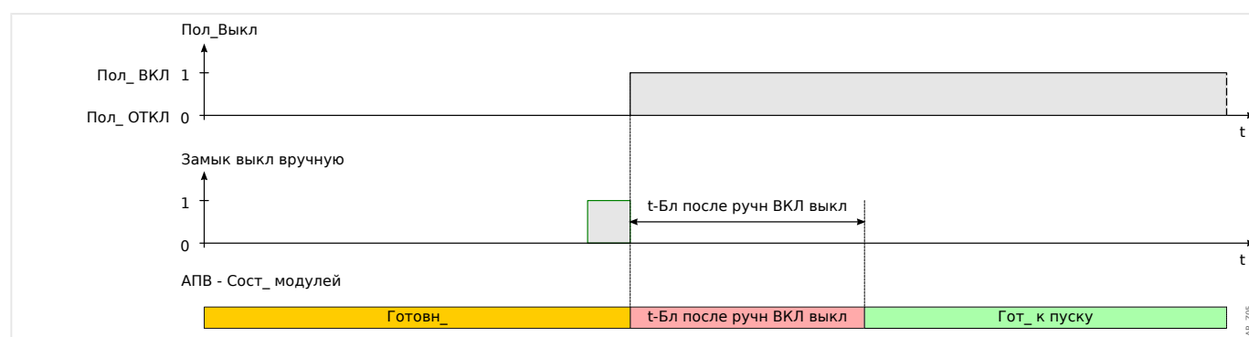
Рис. 51: Состояния автоматического повторного включения во время замыкания выключателя вручную.
