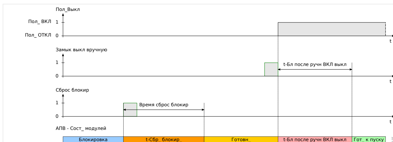
Рис. 53: Логика сброса блокировки АПВ при получении команды сброса блокировки перед замыканием выключателя вручную.
