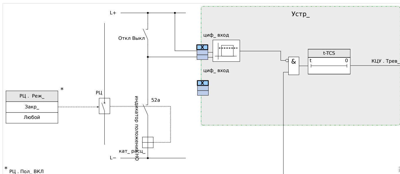
Рис. 58: Пример соединения: контроль цепи отключения только с одним вспомогательным контактом выключателя «Всп Вкл» (52a).
