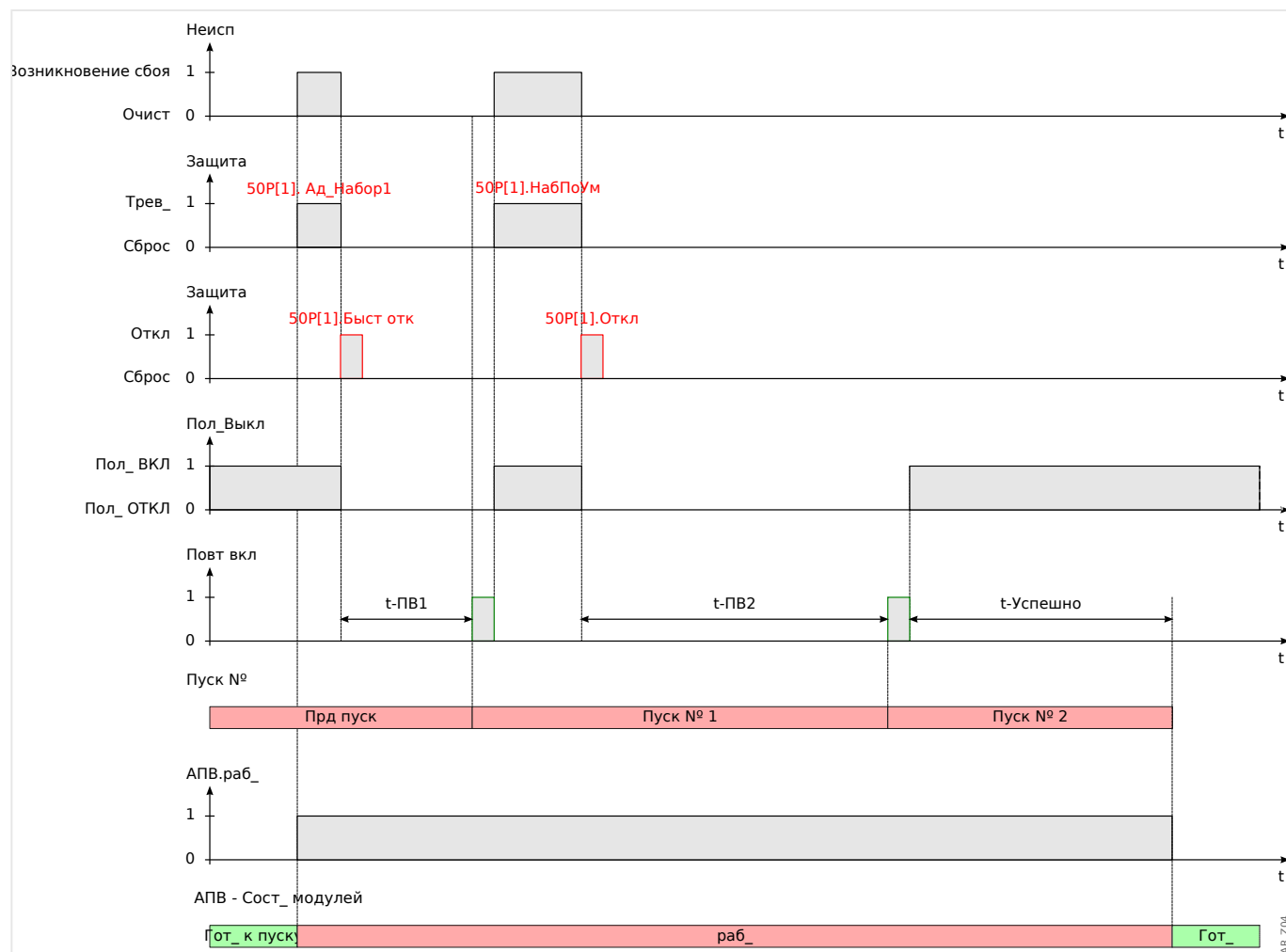
Рис. 50: Диаграмма синхронизации автоматического повторного включения для схемы с 2 удачными попытками автоматического повторного включения и ускорением перед импульсом.
