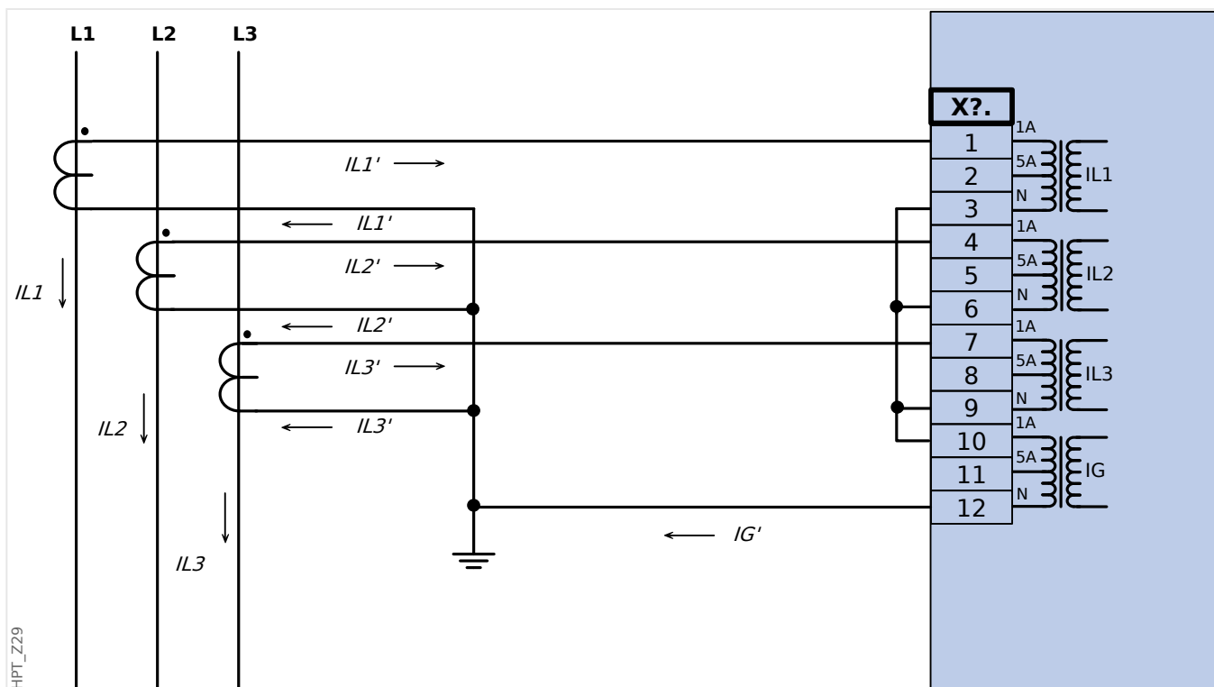
Fig. 22: Medição de corrente de trifásica; I_n secundário = 1 A. Medição corrente terra via conexão Holmgreen; I_{Gnom} secundário = 1 A.
