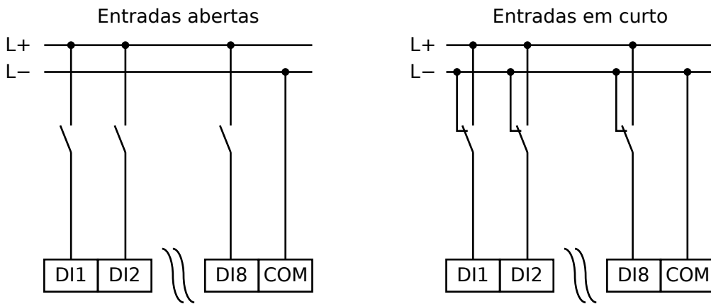
Fig. 81: Estado seguro das entradas digitais
