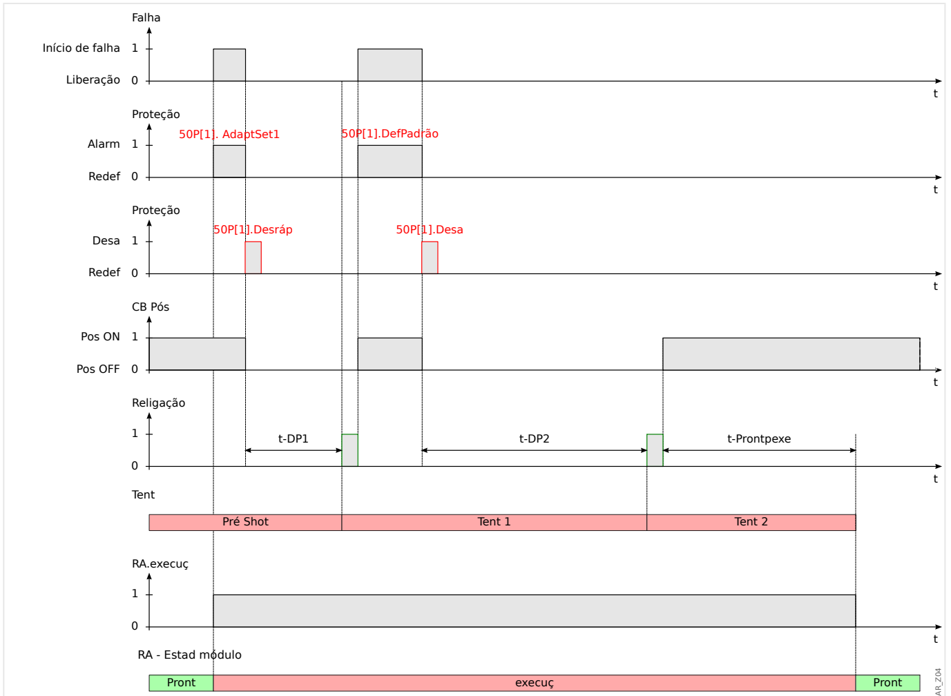
Fig. 50: Diagrama de temporização de religamento automático para esquema de religamento de 2 tentativas bem-sucedidas com aceleração na pré tentativa
