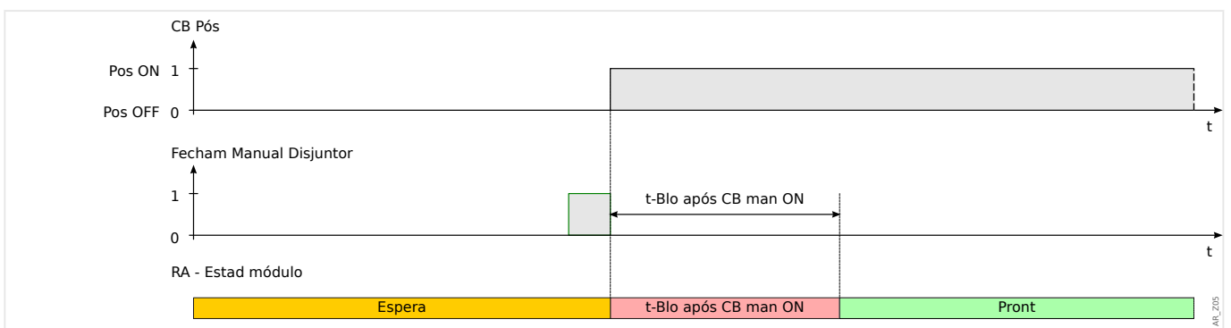
Fig. 51: Estados de religamento automático durante fechamento manual do disjuntor
