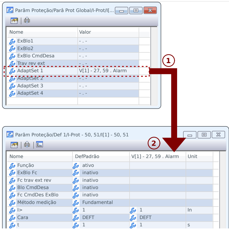
Fig. 2: Uma atribuição a um conjunto de parâmetros adaptativos adiciona valores alternativos aos parâmetros de configuração de grupo.
