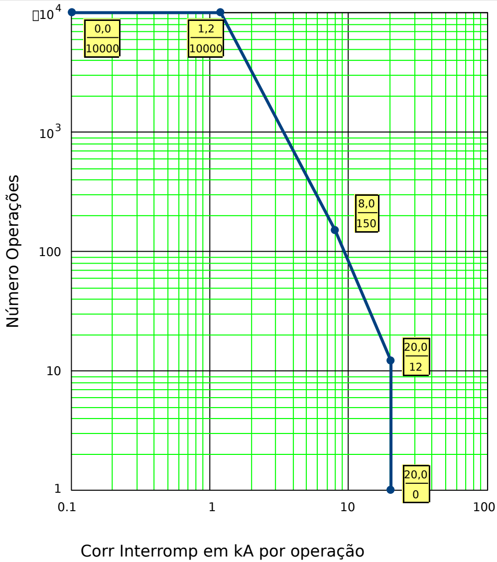
Fig. 65: Curva Manutenção de Disjuntor para Disjuntor normal 25kV
