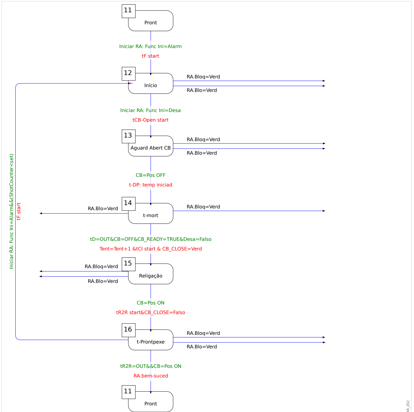
Fig. 48: Ciclo de execução de RA (estado 4).
