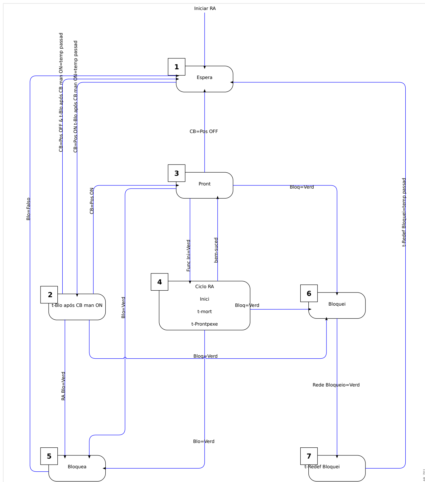
Fig. 47: Diagrama de estado de transição
