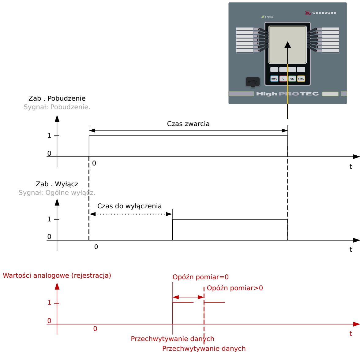
Rys. 70: Rejestrator zwarć: czasy (trwania).
