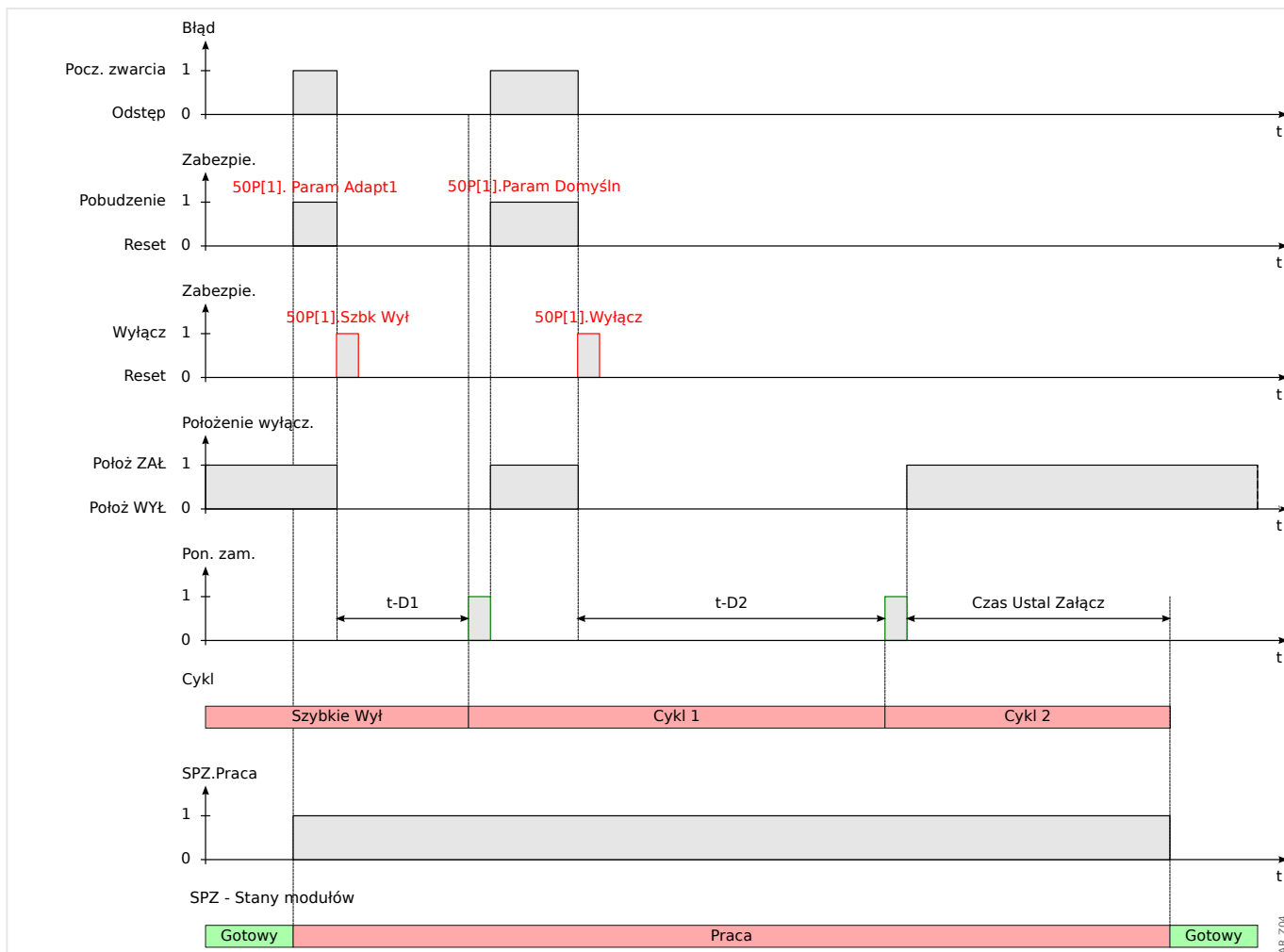
Rys. 50: Schemat czasów SPZ w przypadku udanego planu SPZ z 2 próbami i przyspieszeniem przy próbie wstępnej
