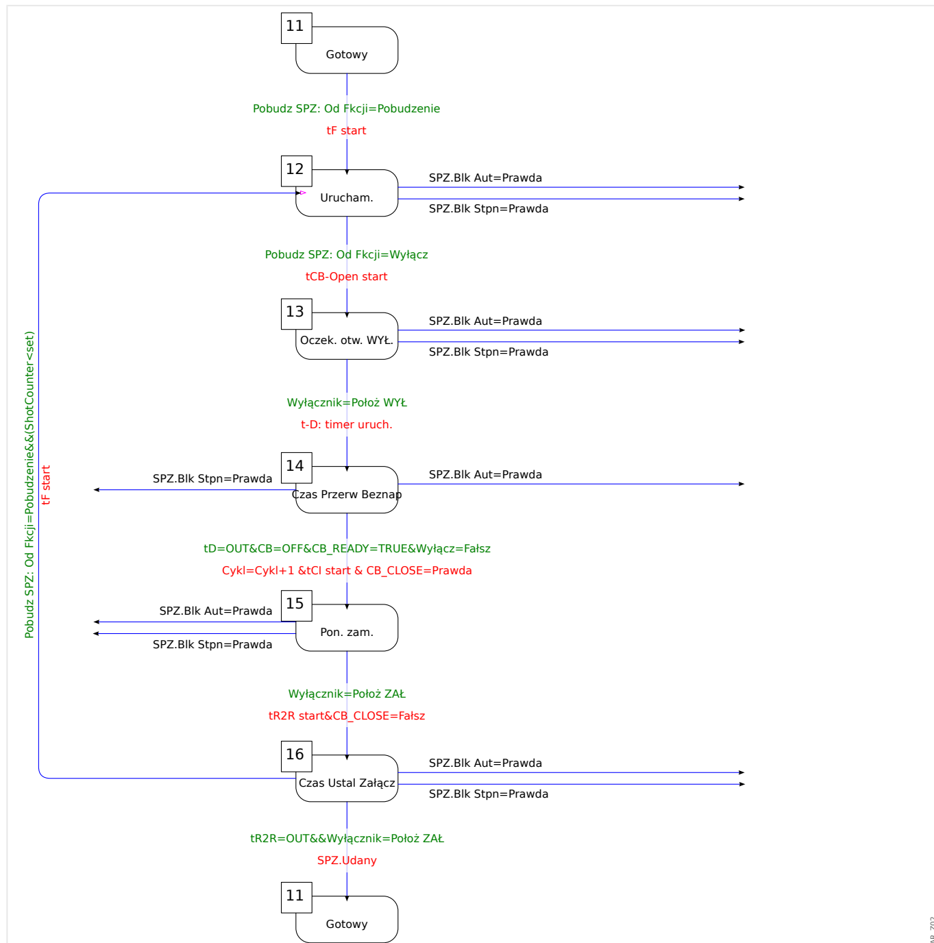
Rys. 48: Cykl pracy SPZ (stan 4).
