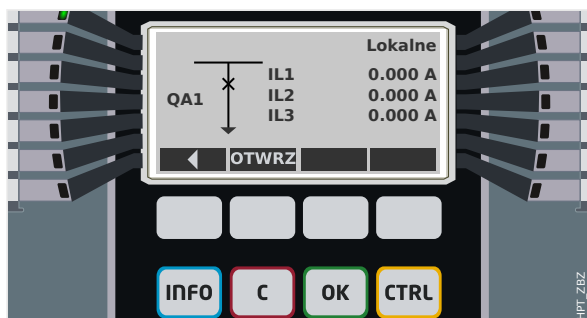
Rys. 60: Przykład strony sterowania z wyłącznikiem w pozycji zamkniętej.
