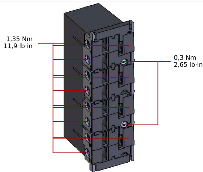
Rys. 80: Łącznik wtykowy ze zintegrowanym elementem zwarciovym (konwencjonalne wejścia prądowe)
