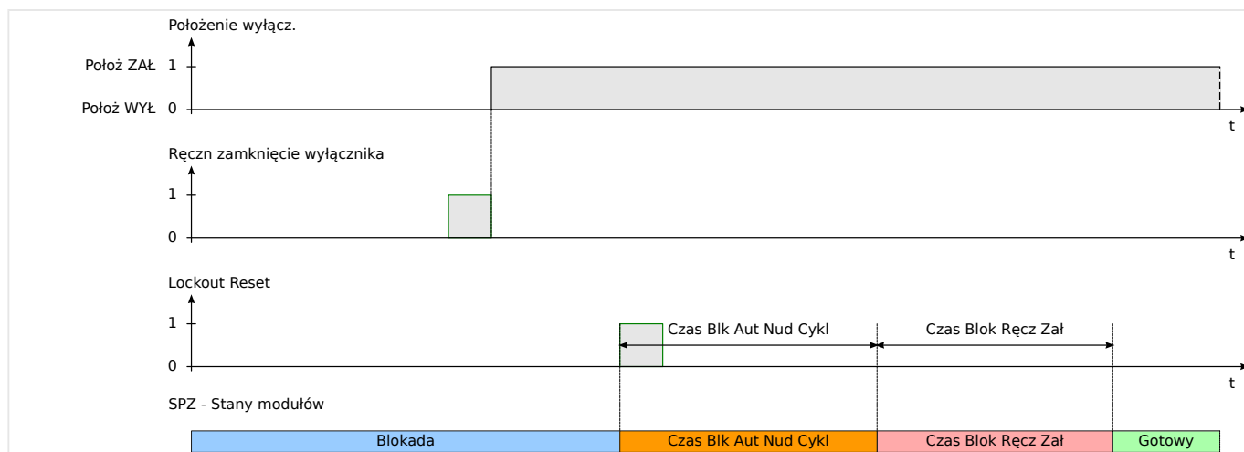
Rys. 54: Logika resetowania blokady automatyki SPZ w przypadku odebrania sygnału resetowania blokady po ręcznym zamknięciu wyłącznika.
