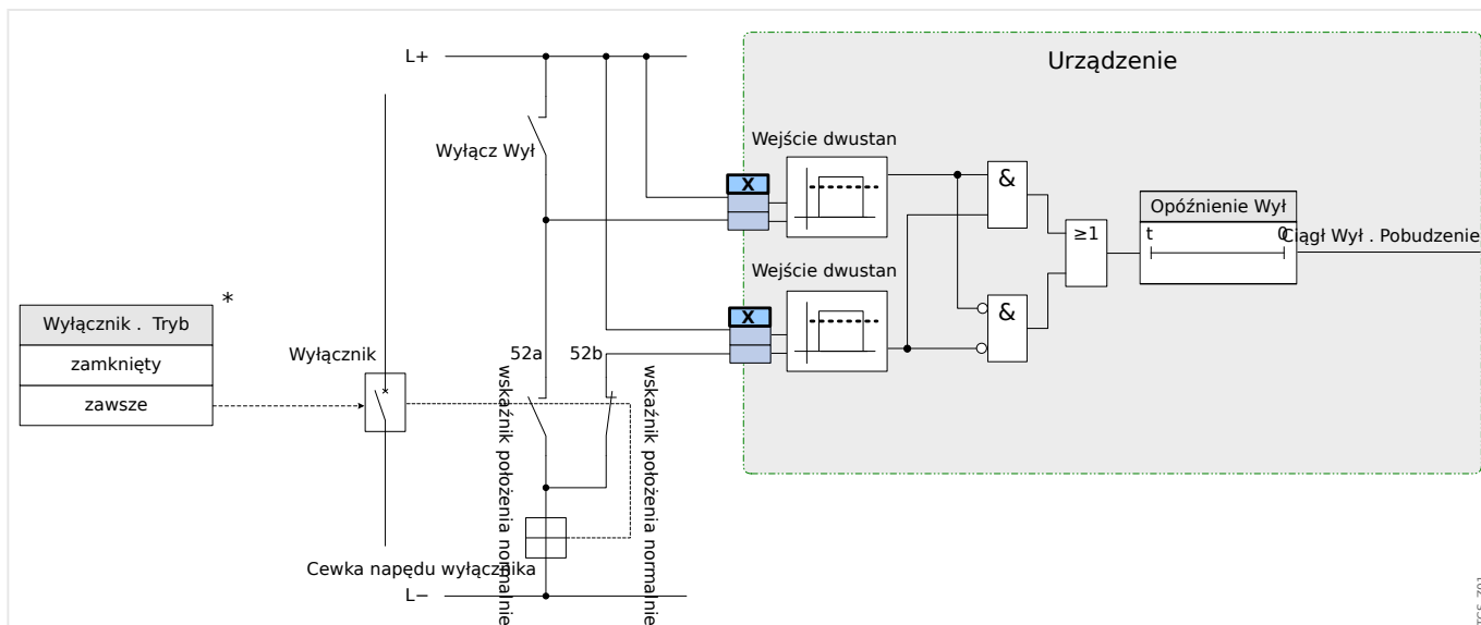
Rys. 57: Przykład okablowania: Układ kontroli ciągłości obwodów wyłącznika z dwoma stykami pomocniczymi wyłącznika „Położ ZAŁ” (52a) i „Położ WYŁ” (52b).
