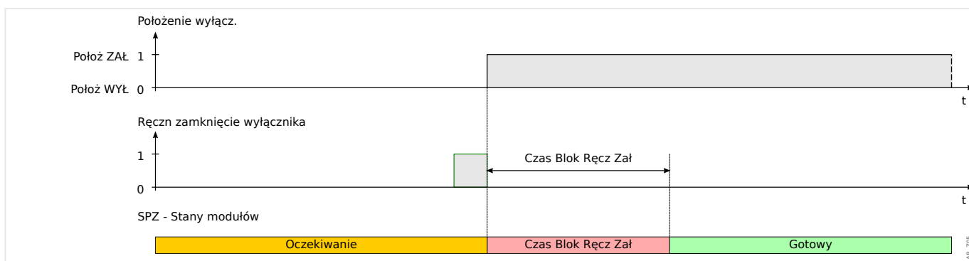
Rys. 51: Stany SPZ podczas ręcznego zamykania wyłącznika.
