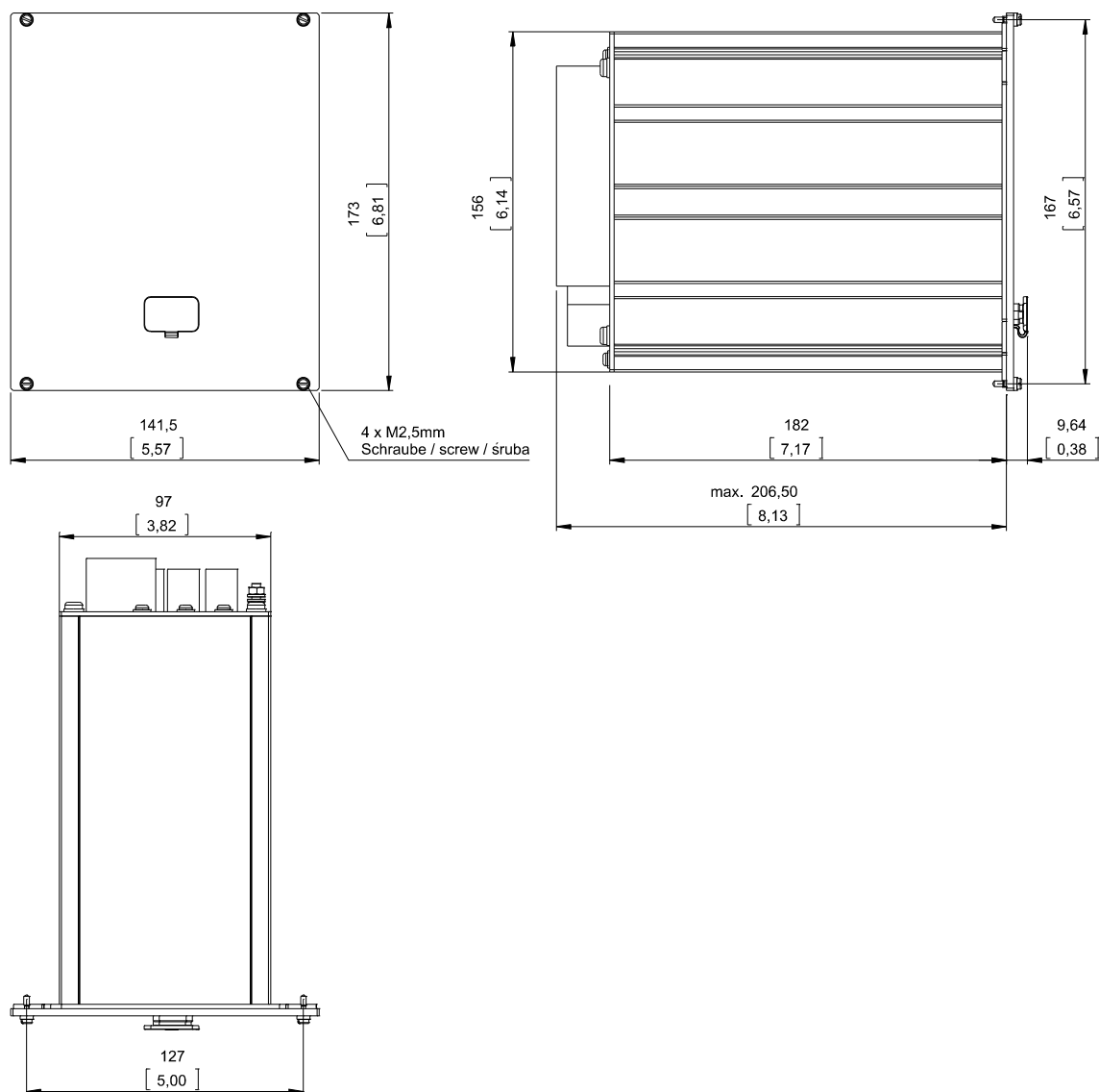
Корпус В1: вид с трех сторон (устройства 19 дюймов)
