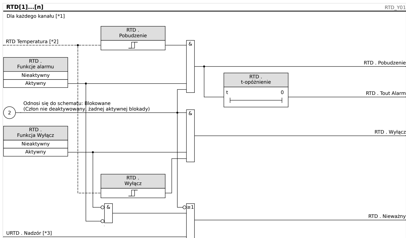
Rys. 57: Ogólna zasada działania (alarm z opóźnieniem, wyzwolenie bezzwłoczne).
