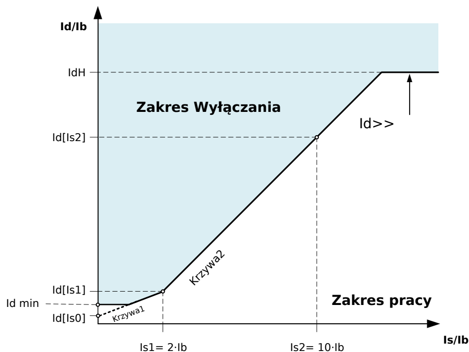
Rys. 49: Stopień nieograniczonego wysokoprądowego zabezpieczenia różnicowego I_{dH}
