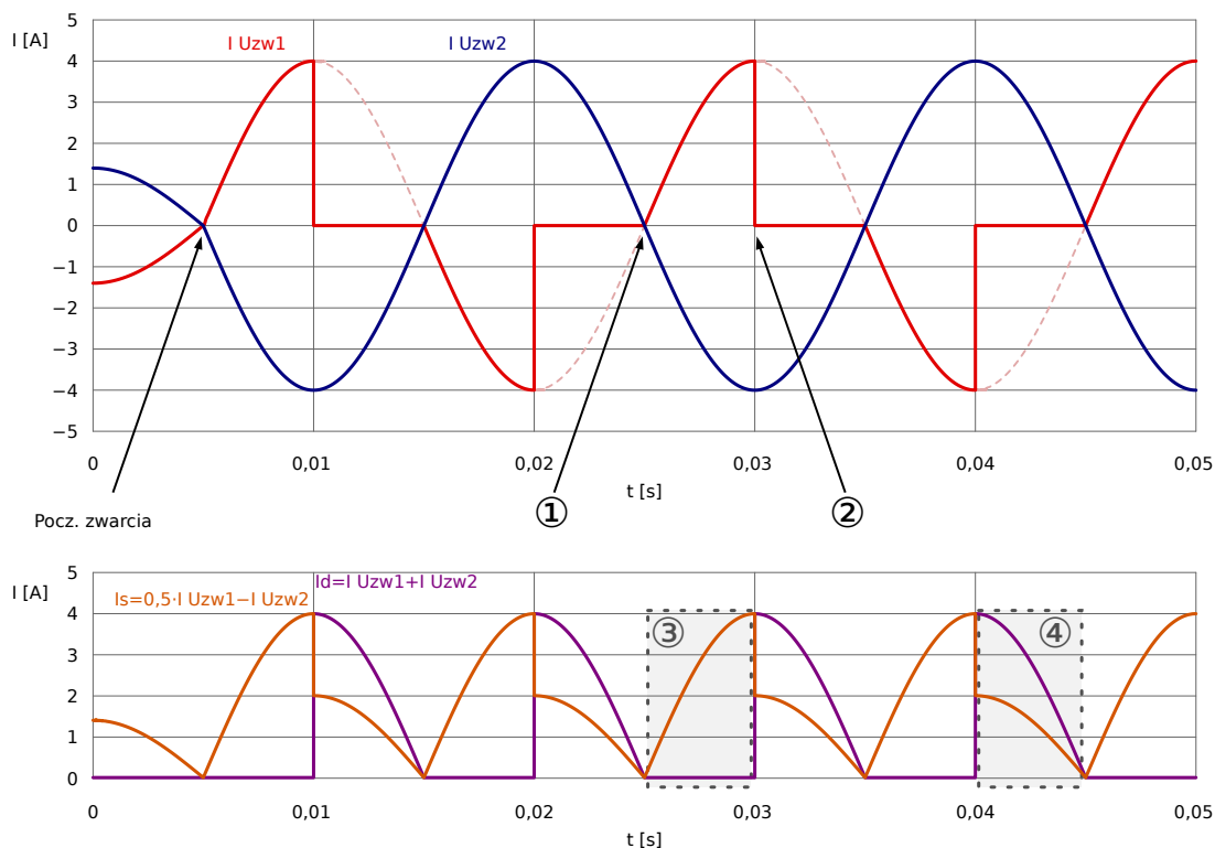
Rys. 48: Charakterystyka I_d i I_s z nasyceniem po stronie W1 przekładnika prądowego w przypadku zwarcia zewnętrznego.
