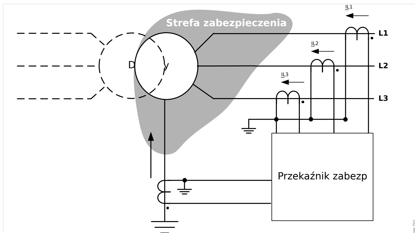
Rys. 50: Zasada działania zabezpieczenia różnicowego ziemnozwarciowego w uzwojeniach transformatorów połączonych w gwiazdę.
