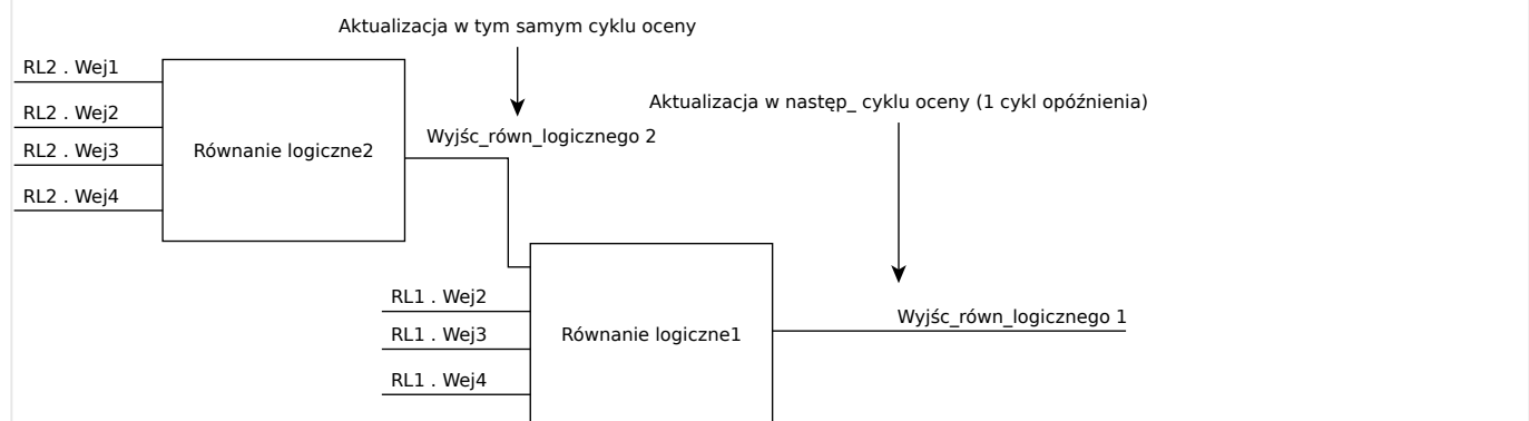
Rys. 77: Ukł. kaskadowy w porządku malejącym
