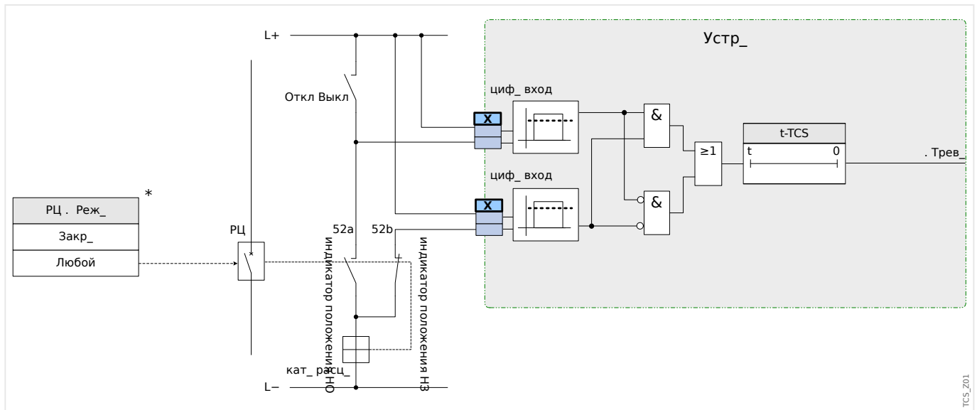
Рис. 68: Пример соединения: контроль цепи отключения с двумя вспомогательными контактами выключателя «Всп Вкл» (52a) и «Всп Выкл» (52b).
