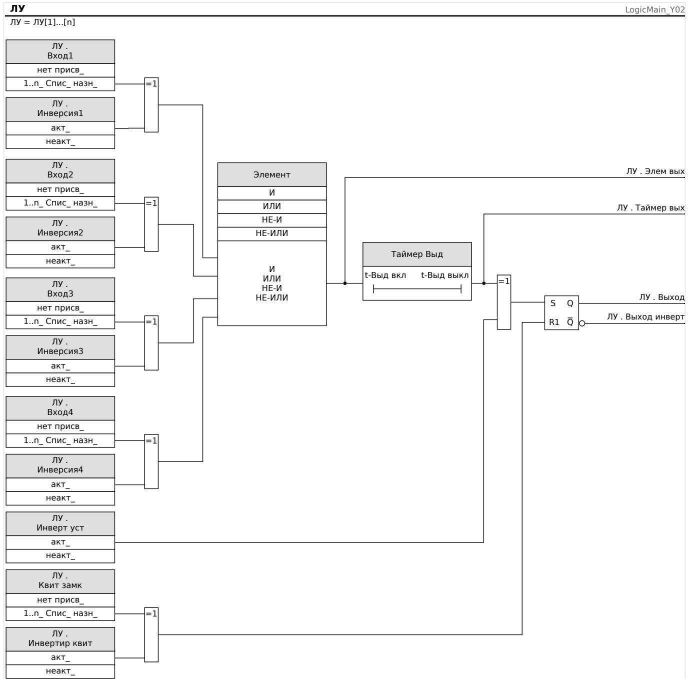
Рис. 83: Подробный обзор — общая логическая схема.
