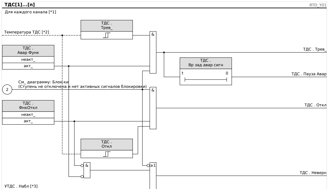
Рис. 67: Общий принцип работы (аварийный сигнал с задержкой, отключение без задержки).
