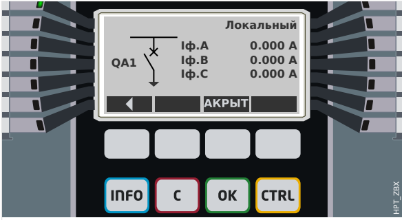
Рис. 73: Пример страницы управления, выключатель в разомкнутом положении.
