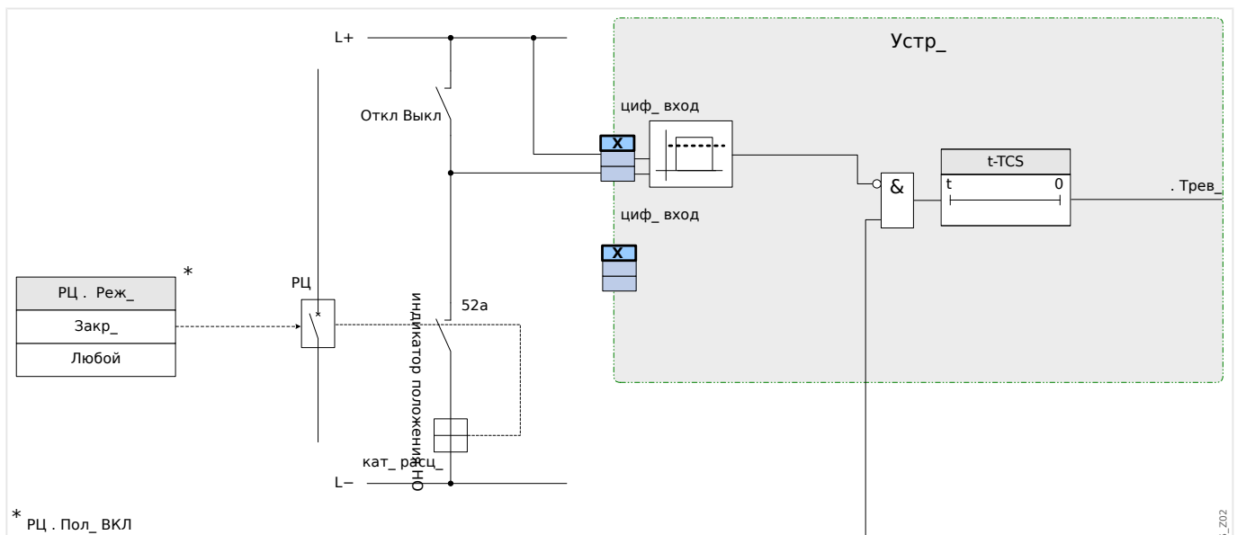
Рис. 69: Пример соединения: контроль цепи отключения только с одним вспомогательным контактом выключателя «Всп Вкл» (52a).
