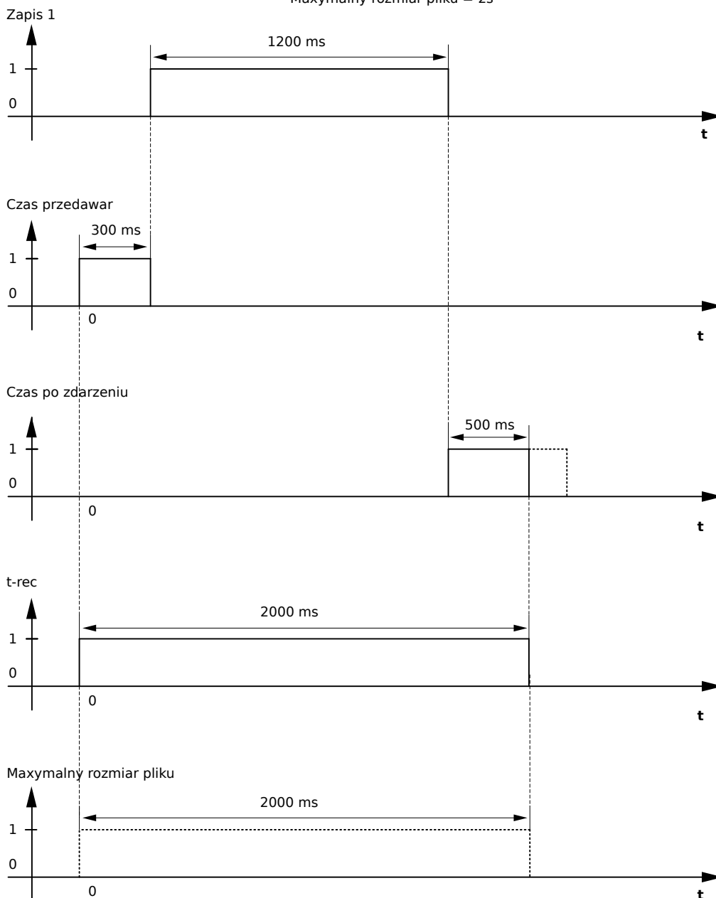
Rys. 79: Przykładowy wykres czasów pracy rejestratora zakłóceń I
