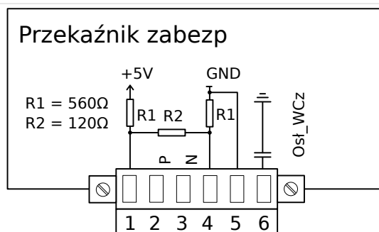
Rys. 30: Przypisanie elektromechaniczne
