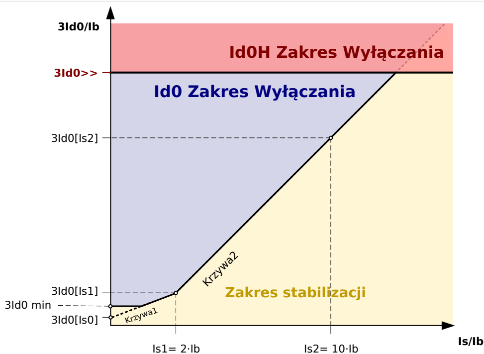
Rys. 53: Wartość pobudzenia „3Id0>>” prądu różnicowego doziemnego w oparciu o prąd znamionowy „lb” obiektu zabezpieczanego.
