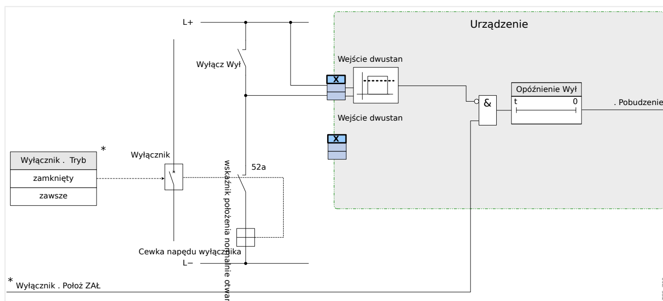
Rys. 69: Przykład okablowania: Układ kontroli ciągłości obwodów wyłącznika z tylko jednym stykiem pomocniczym wyłącznika „Położ ZAŁ” (52a).
