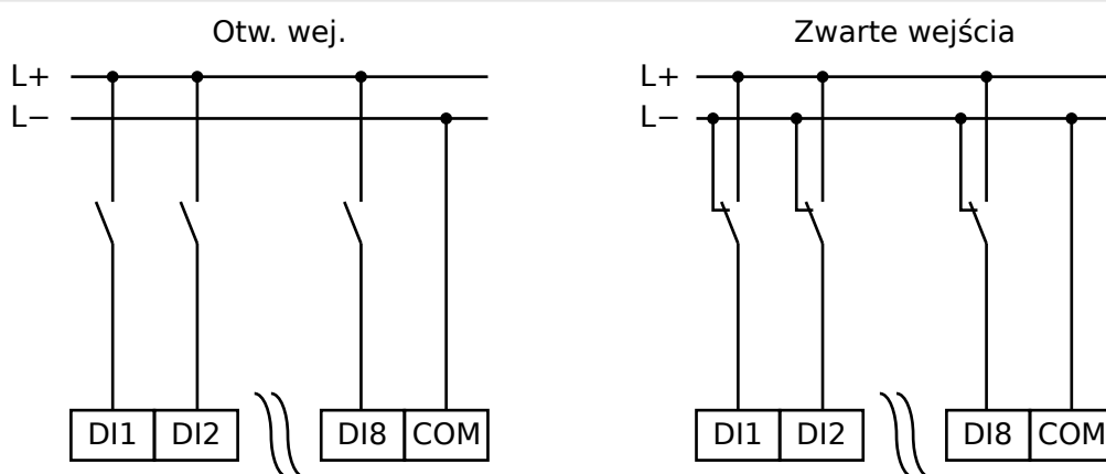
Rys. 90: Stan bezpieczny wejść dwustanowych
