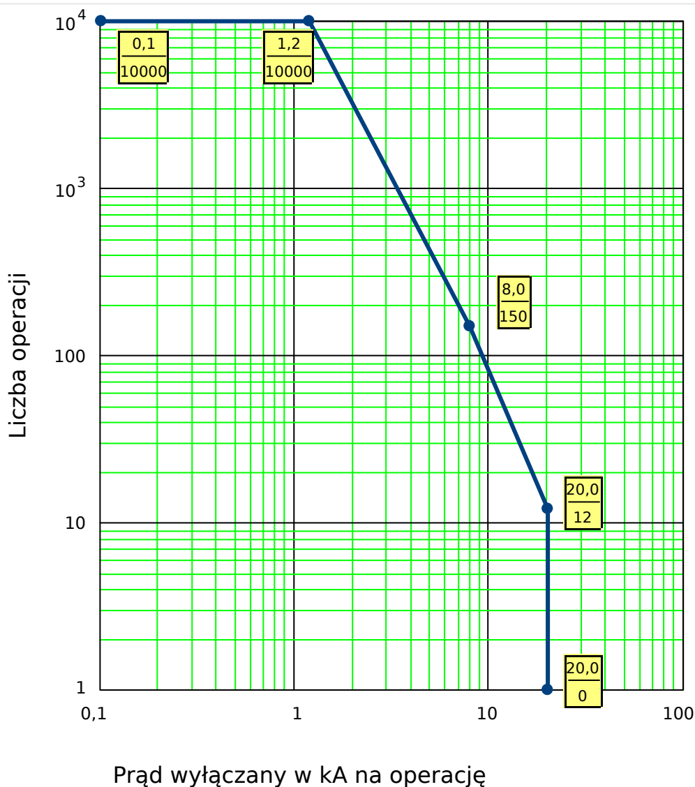
Rys. 76: Krzywa konserwacji wyłącznika typowego wyłącznika 25 kV
