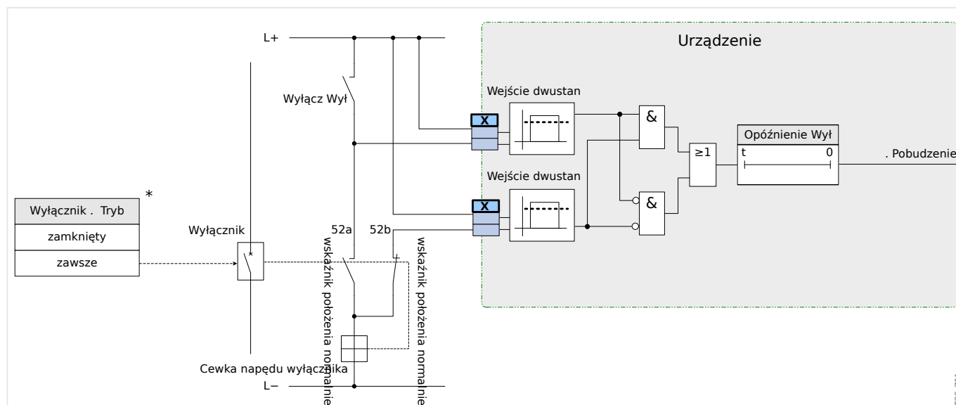
Rys. 68: Przykład okablowania: Układ kontroli ciągłości obwodów wyłącznika z dwoma stykami pomocniczymi wyłącznika „Położ ZAŁ” (52a) i „Położ WYŁ” (52b).
