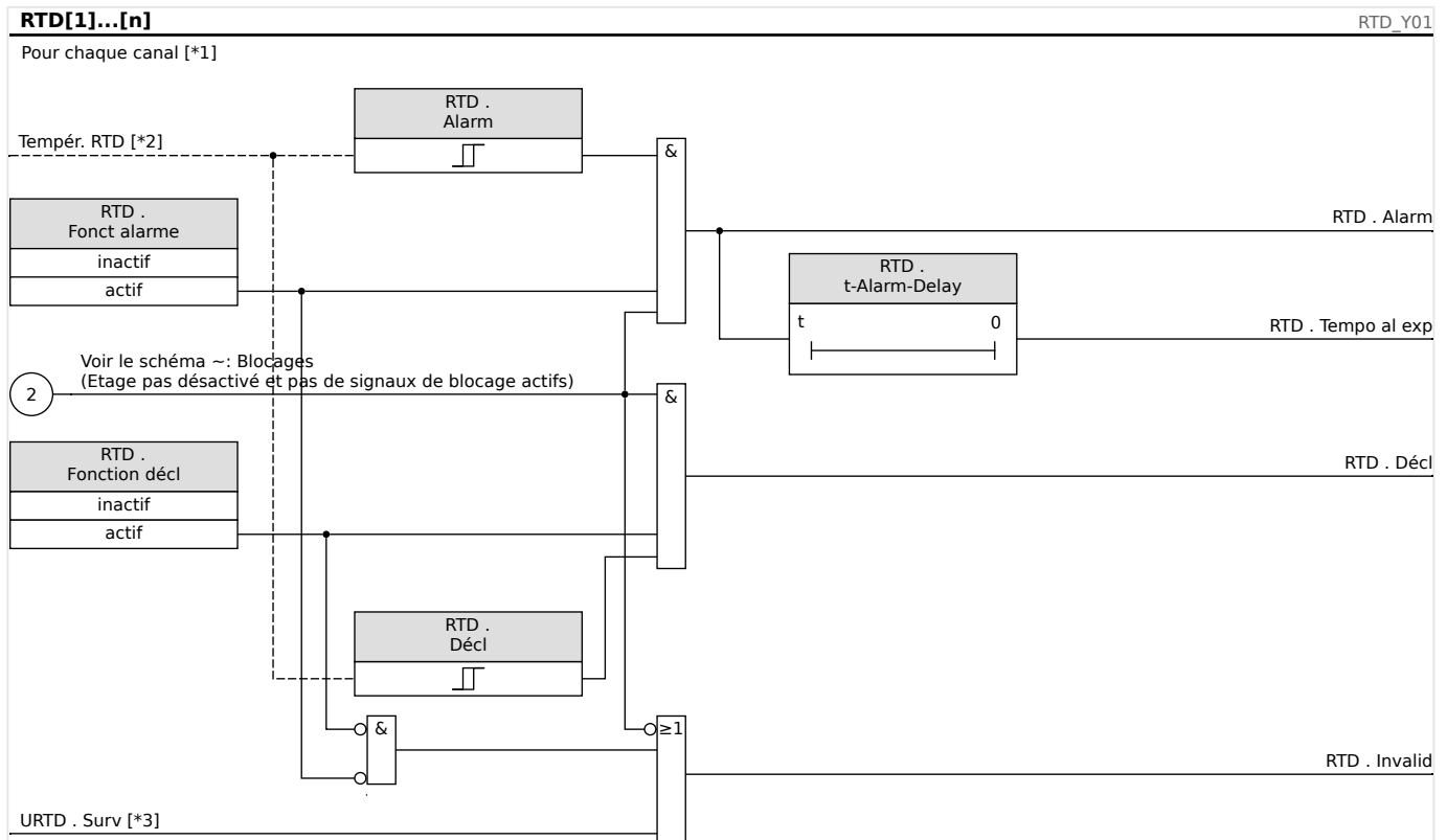
Fig. 67: Principe de fonctionnement général (alarme retardée, déclenchement non retardé).
