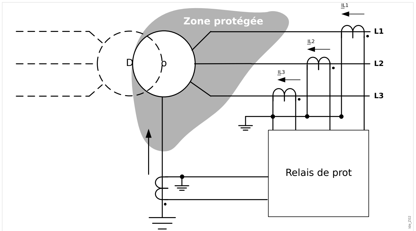
Fig. 52: Principe de protection différentielle du courant à la terre connecté à la partie en étoile de l'enroulement d'un transformateur
