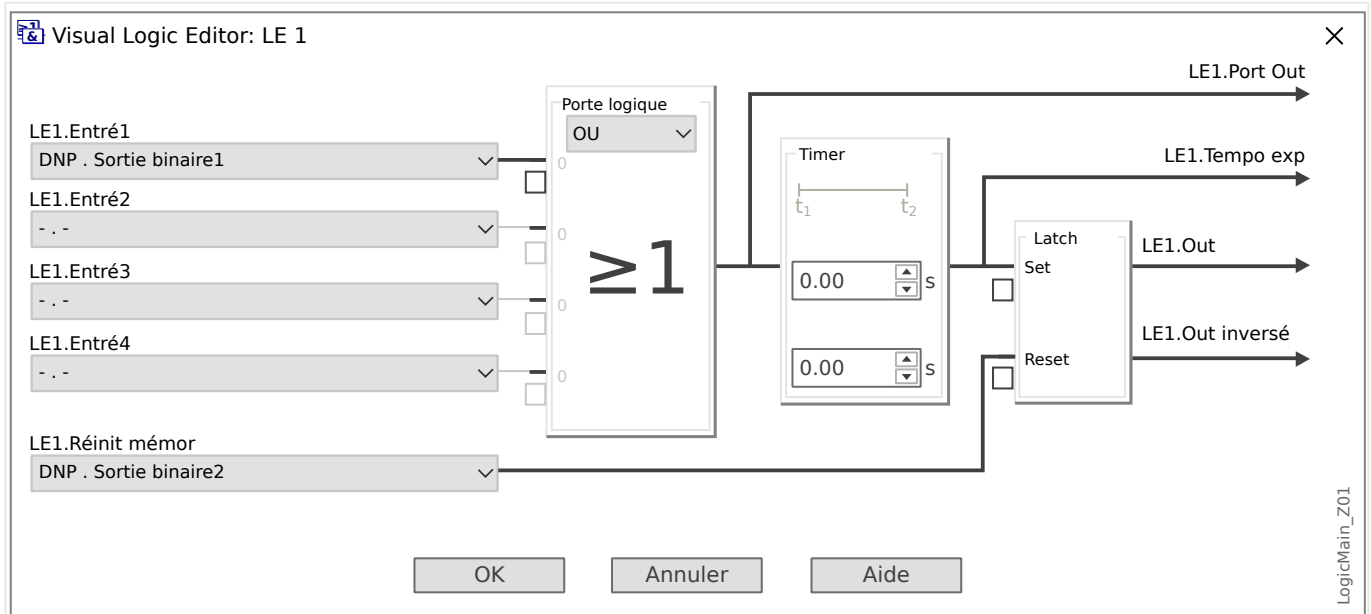
Fig. 42: Exemple (Smart view) : Créer des états stables des signaux d'impulsion du DNP.
