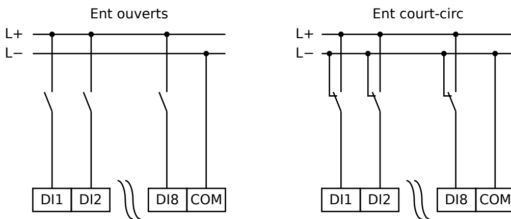
Fig. 90: État sécuritaire des entrées numériques
