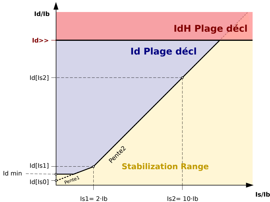
Fig. 51: Valeur IdH d'étape de niveau supérieur et non limitée de protection différentielle
