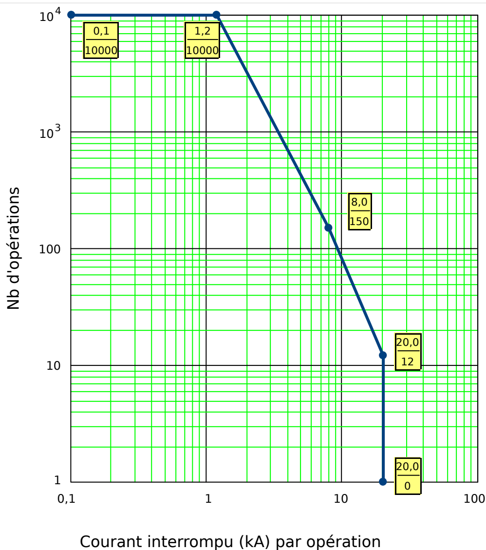
Fig. 76: Courbe de maintenance du disj pour un disj 25 ~kV typique
