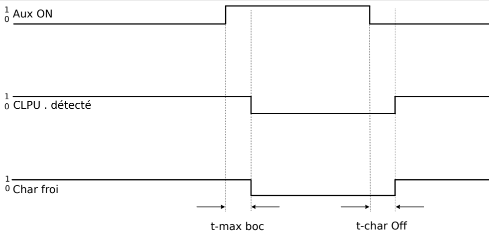
Fig. 65: Exemple de mode : Position du disjoncteur.
