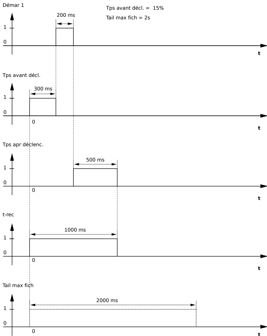
Fig. 80: Exemple de diagramme des temps de l'enregistreur de perturbations II
