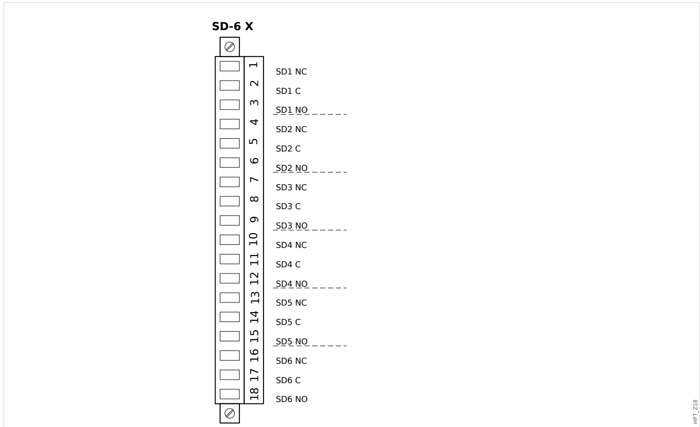
Fig. 13: Asignación electromecánica
