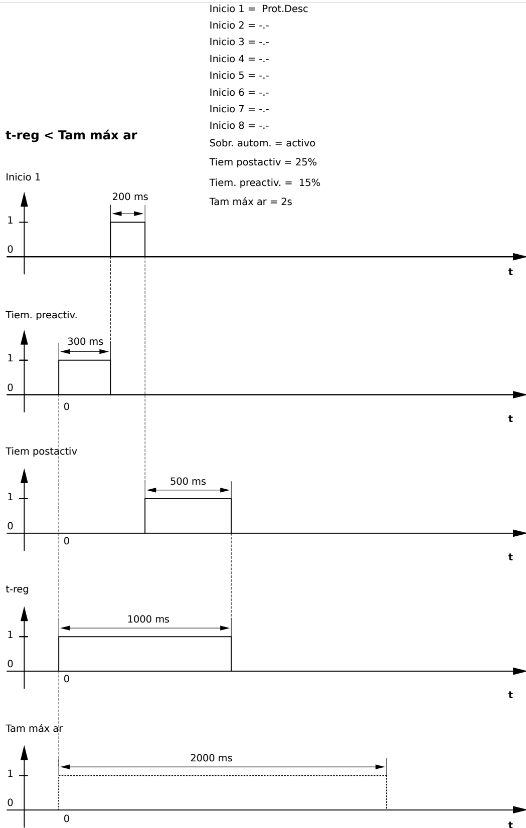
Fig. 80: Ejemplo 2: cuadro de intervalos del registrador de perturbaciones
