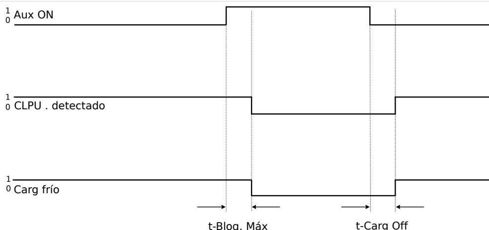
Fig. 65: Modo de ejemplo: Posición de interruptor.
