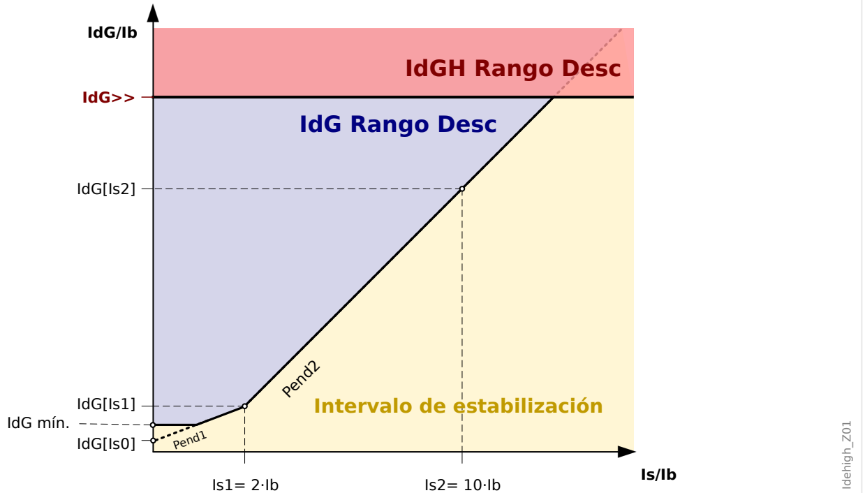
Fig. 53: Valor de selección »IdG>>« de la corriente de diferencial de tierra basada en la corriente nominal »lb« del objeto de protección relacionado.
