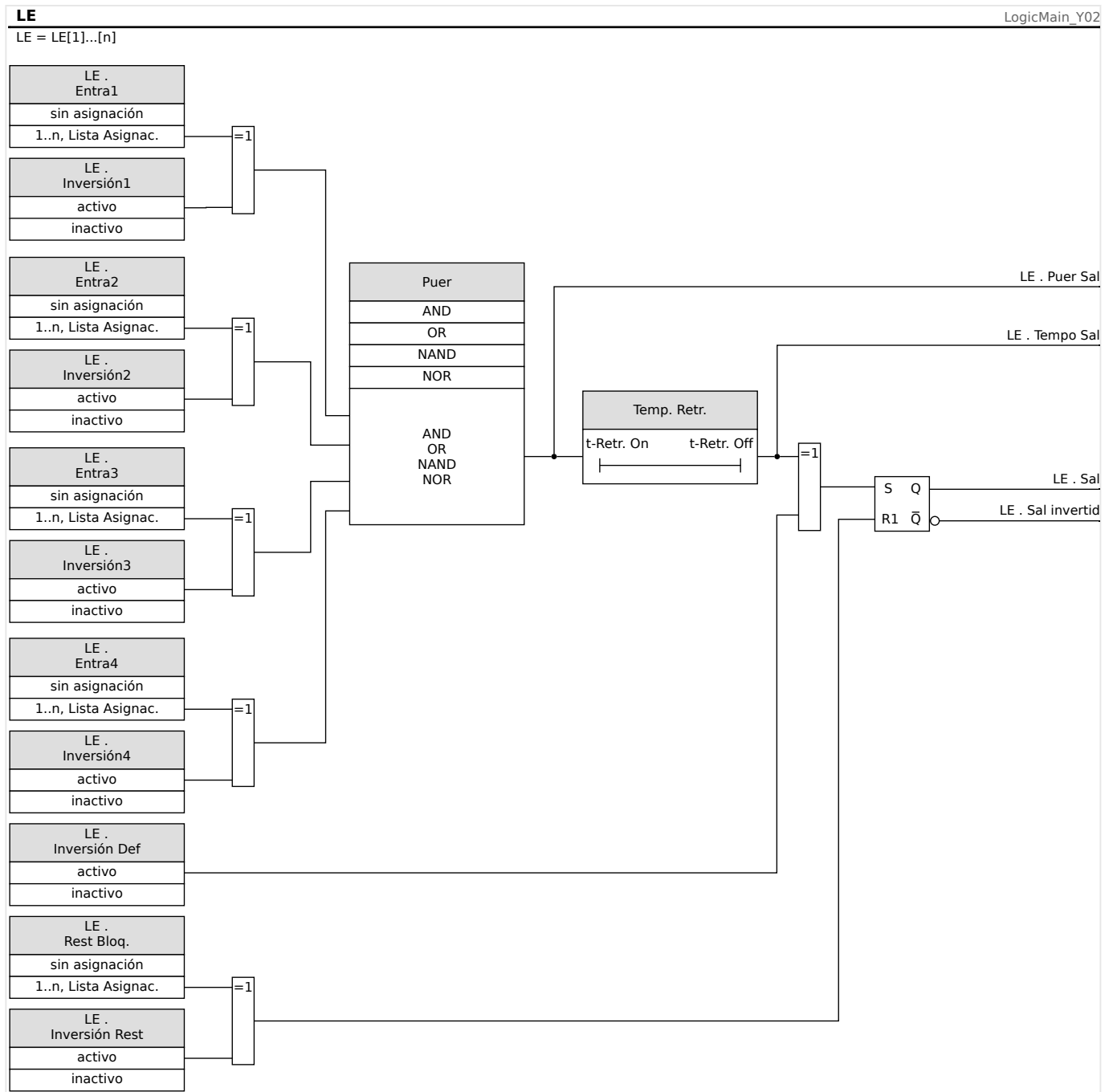
Fig. 83: Descripción detallada - Diagrama de lógica general.
