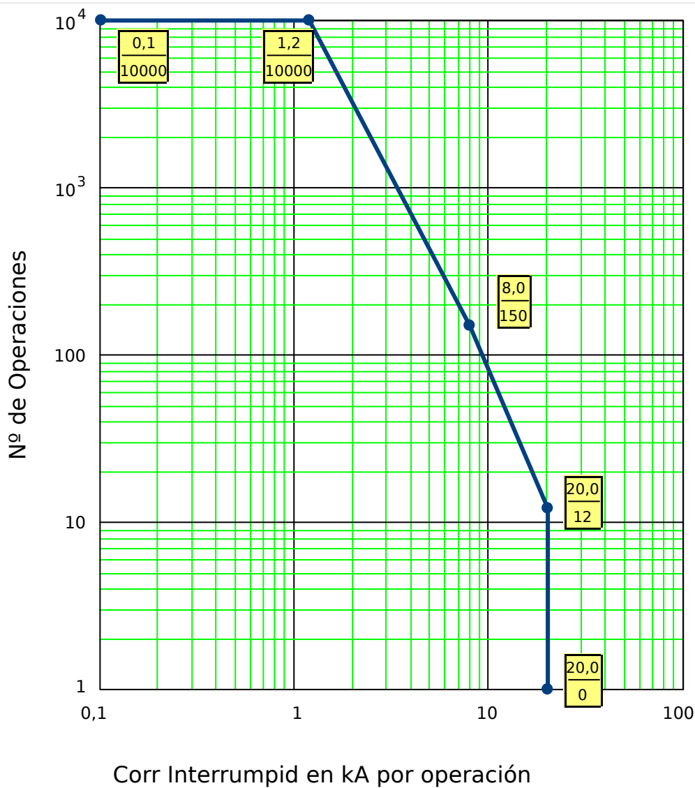
Fig. 76: Curva Mantenim Interruptor para Interrupt Circuito típico 25kV
