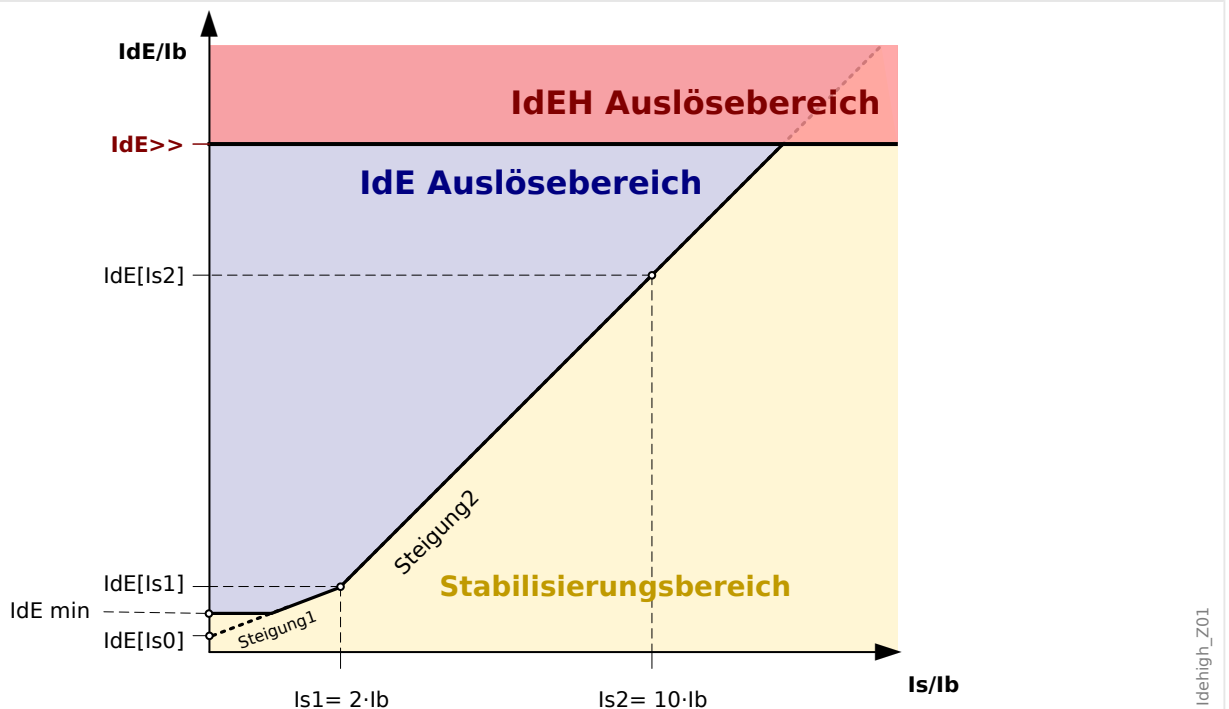
Abb. 55: Ansprechwert »IdE>>« des Erddifferenzialstromes bezogen auf den Nennstrom »lb« des entsprechenden Schutzobjektes.
