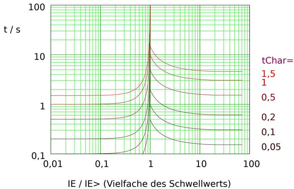
Abb. 72: RINV: Rückfallverzögerung (linke Hälfte, IE < I_{E>} ) und Auslöseverzögerung (rechte Hälfte, IE > I_{E>} ), Beispieldiagramm für I_{max} = 20 \cdot I_{E>} .
