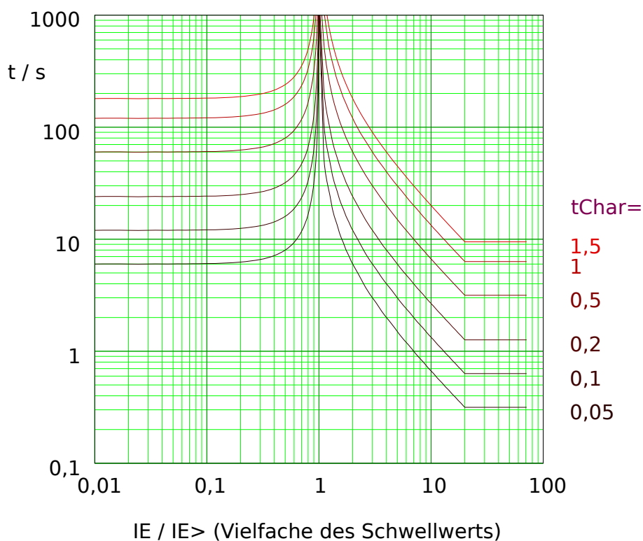
Abb. 71: LINV: Rückfallverzögerung (linke Hälfte, IE < I_{E>} ) und Auslöseverzögerung (rechte Hälfte, IE > I_{E>} ), Beispieldiagramm für I_{max} = 20 \cdot I_{E>} .
