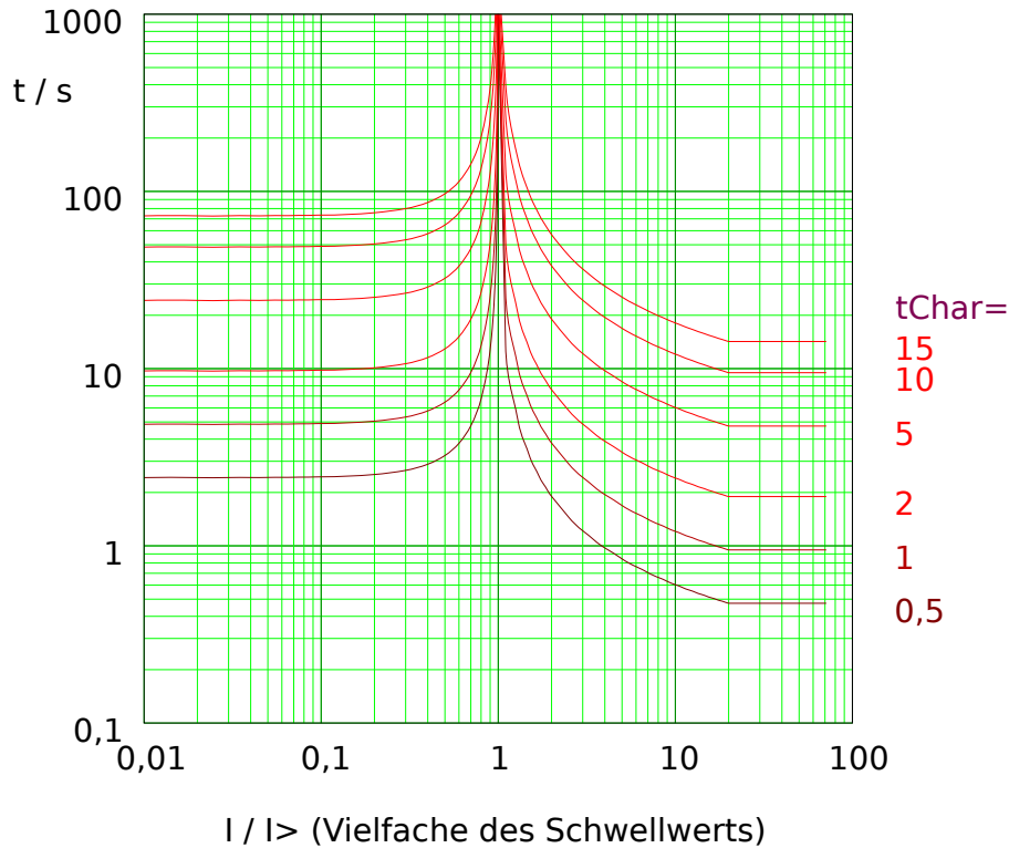
Abb. 61: MINV: Rückfallverzögerung (linke Hälfte, I < I_{>} ) und Auslöseverzögerung (rechte Hälfte, I > I_{>} ), Beispieldiagramm für I_{max} = 20 \cdot I_{>} .
