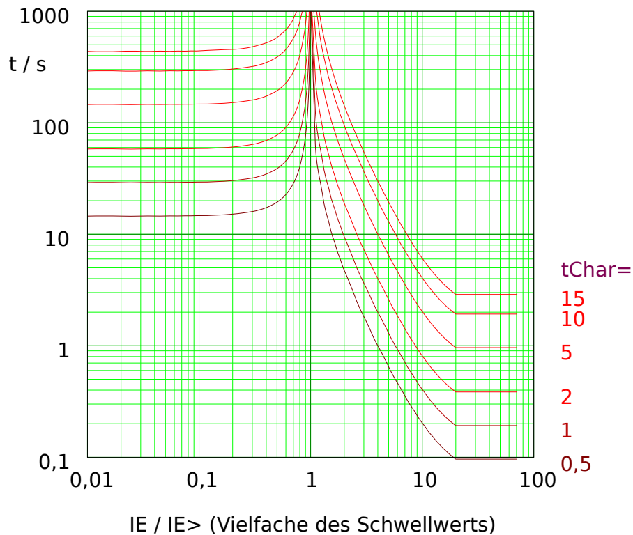
Abb. 75: EINV: Rückfallverzögerung (linke Hälfte, IE < I_{E>} ) und Auslöseverzögerung (rechte Hälfte, IE > I_{E>} ), Beispieldiagramm für I_{max} = 20 \cdot I_{E>} .
