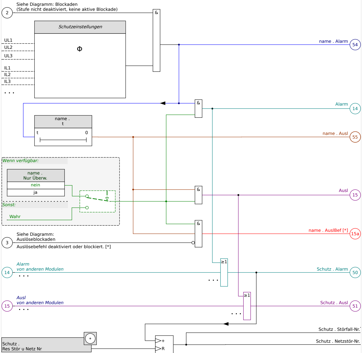
Abb. 47: Grobe Skizze der Funktionalität einer HighPROTEC-Schutzfunktion.
