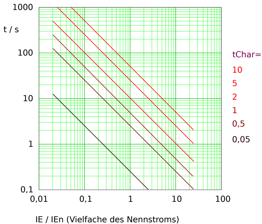
Abb. 78: Auslösekurve „IT“, wobei nur der Bereich IE > I_{E>} jeweils anwendbar ist. Beispieldiagramm für gemessenen (nicht empfindlichen) Erdstrom.
