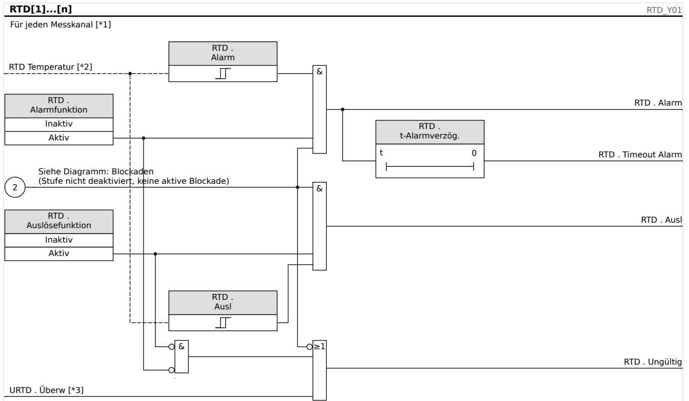
Abb. 86: Generelles RTD-Funktionsprinzip.
