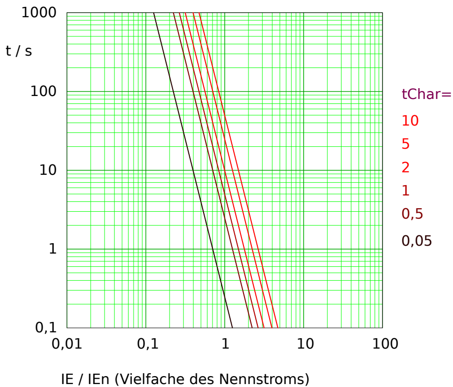
Abb. 80: Auslösekurve „I4T“, wobei nur der Bereich IE > I_{E>} jeweils anwendbar ist. Beispieldiagramm für gemessenen (nicht empfindlichen) Erdstrom.
