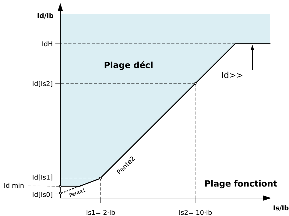
Fig. 49: Valeur IdH d'étape de niveau supérieur et non limitée de protection différentielle
