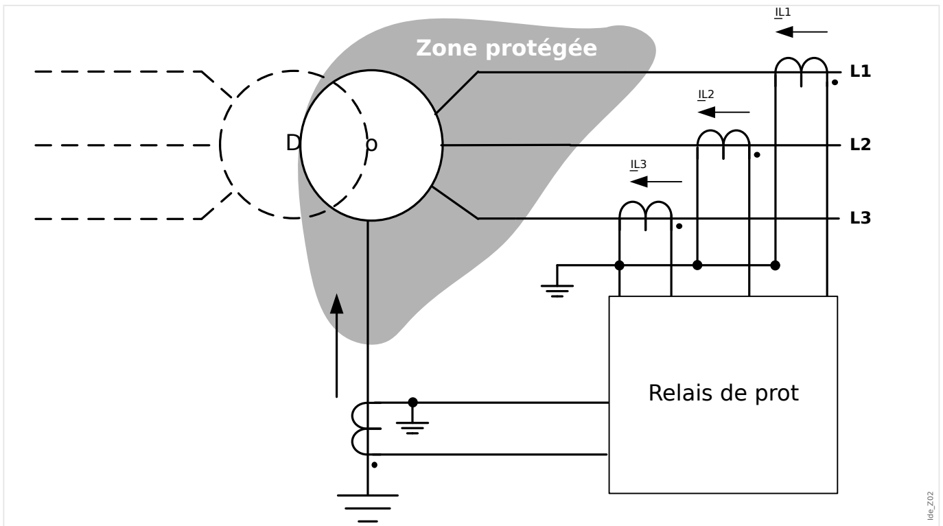
Fig. 50: Principe de protection différentielle du courant à la terre connecté à la partie en étoile de l'enroulement d'un transformateur
