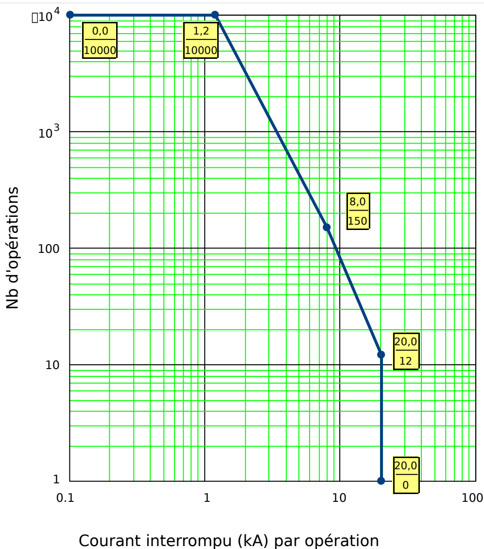
Fig. 66: Courbe de maintenance du disj pour un disj 25 ~kV typique
