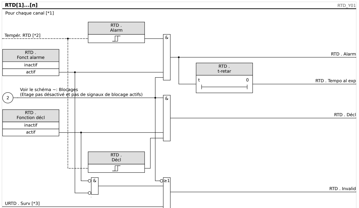
Fig. 57: Principe de fonctionnement général (alarme retardée, déclenchement non retardé).
