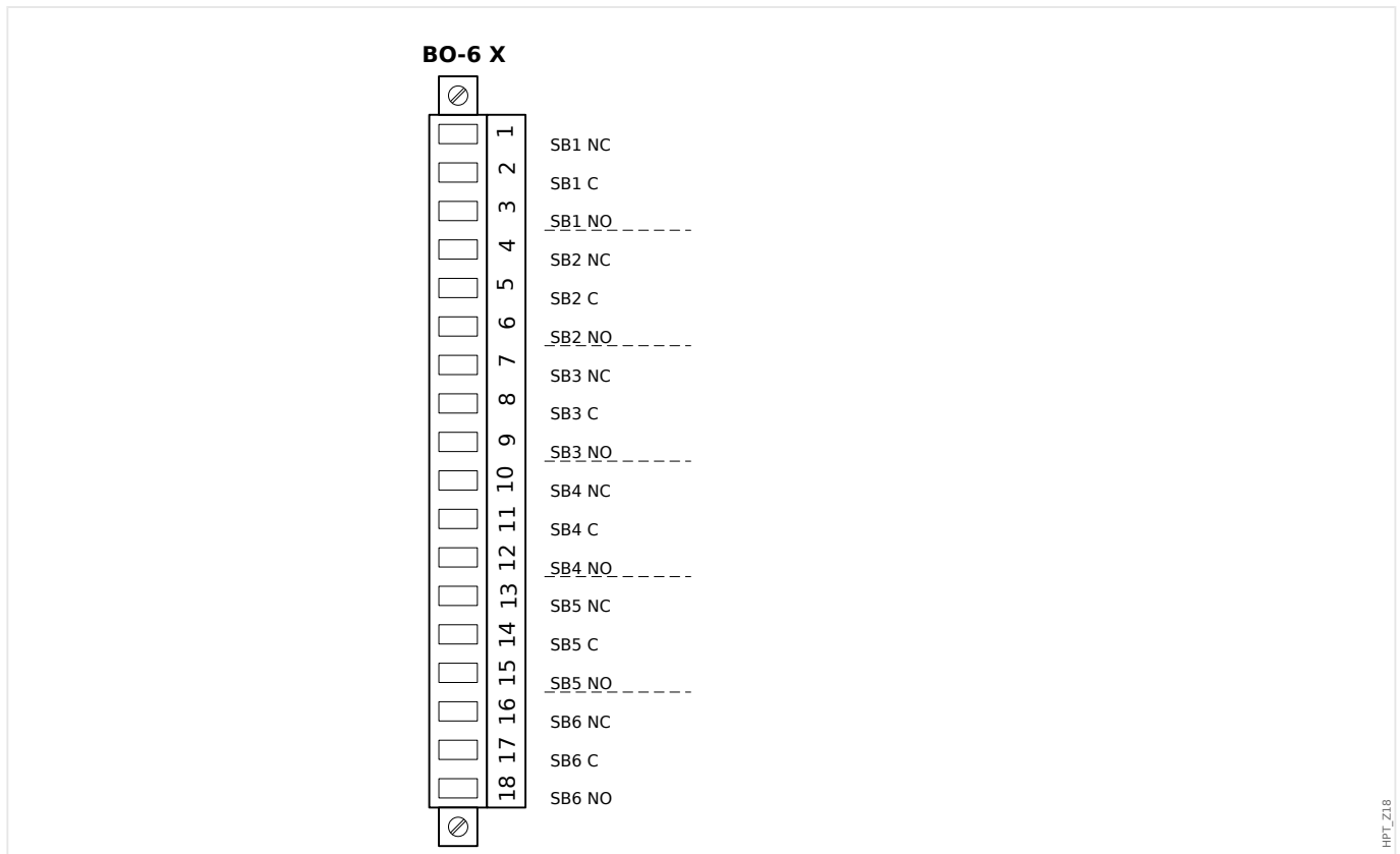
Fig. 13: Affectation électromécanique
