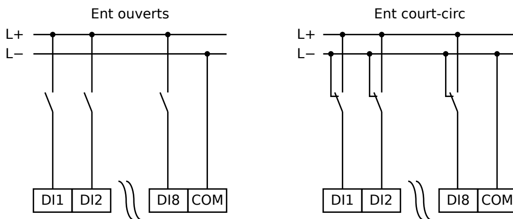
Fig. 82: État sécuritaire des entrées numériques
