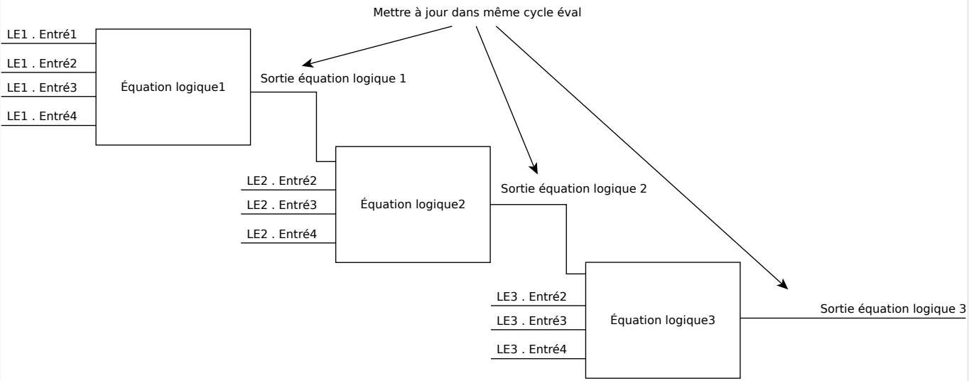
Fig. 76: En cascade ordre croissant
