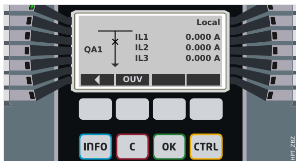
Fig. 61: Exemple de page de contrôle, avec le « disjoncteur » en position fermée.
