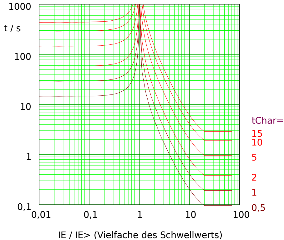
Abb. 78: EINV: Rückfallverzögerung (linke Hälfte, IE < I_{E>} ) und Auslöseverzögerung (rechte Hälfte, IE > I_{E>} ), Beispieldiagramm für I_{max} = 20 \cdot I_{E>} .
