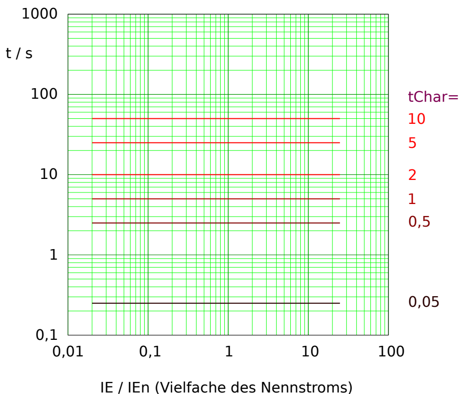
Abb. 80: Auslösekurve „Therm Flat“, wobei nur der Bereich IE > I_{E>} jeweils anwendbar ist. Beispieldiagramm für gemessenen (nicht empfindlichen) Erdstrom.
