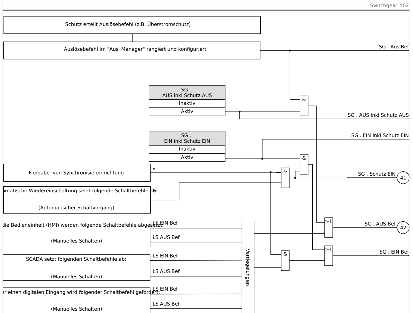
Abb. 97: Verriegelungen. (Für die mit „*“ markierten Teile gilt: Verfügbarkeit hängt von der bestellten Gerätevariante ab.)
