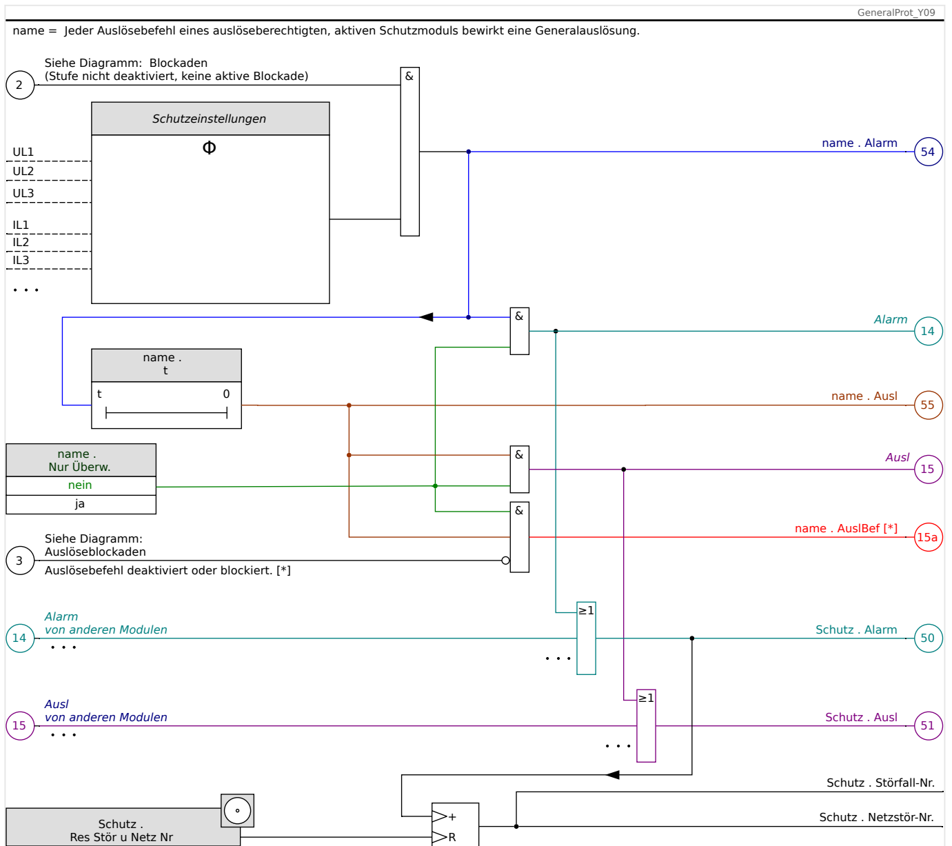
Abb. 47: Grobe Skizze der Funktionalität einer HighPROTEC-Schutzfunktion.
