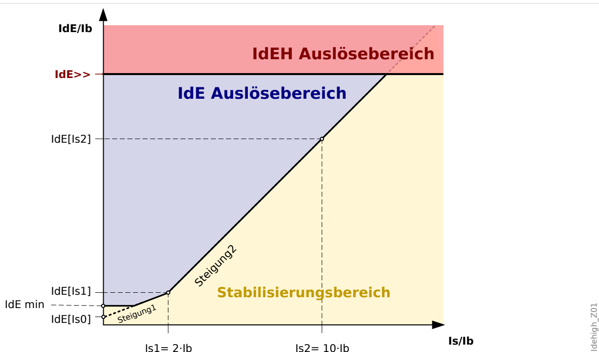
Abb. 58: Ansprechwert »IdE>>« des Erddifferentialstromes bezogen auf den Nennstrom »lb« des entsprechenden Schutzobjektes.
