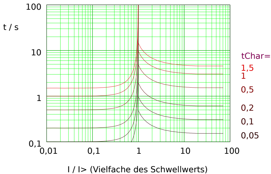
Abb. 63: RINV: Rückfallverzögerung (linke Hälfte, I < I_{>} ) und Auslöseverzögerung (rechte Hälfte, I > I_{>} ), Beispieldiagramm für I_{max} = 20 \cdot I_{>} .
