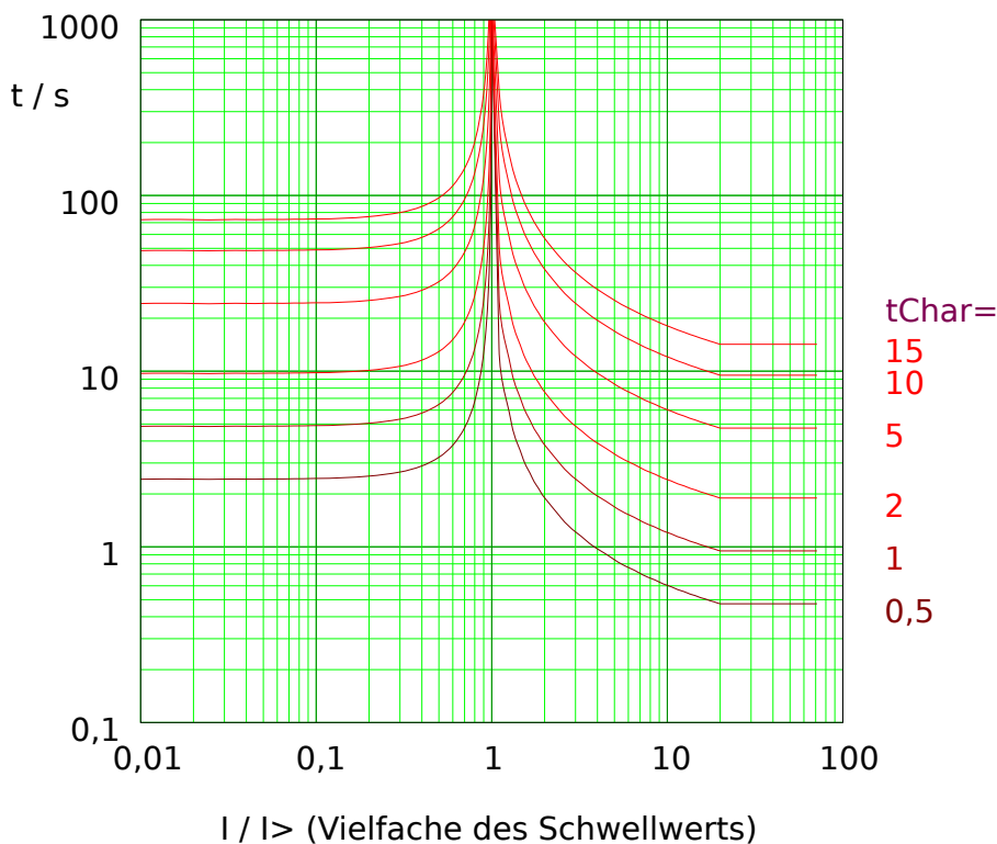
Abb. 64: MINV: Rückfallverzögerung (linke Hälfte, I < I_{>} ) und Auslöseverzögerung (rechte Hälfte, I > I_{>} ), Beispieldiagramm für I_{max} = 20 \cdot I_{>} .
