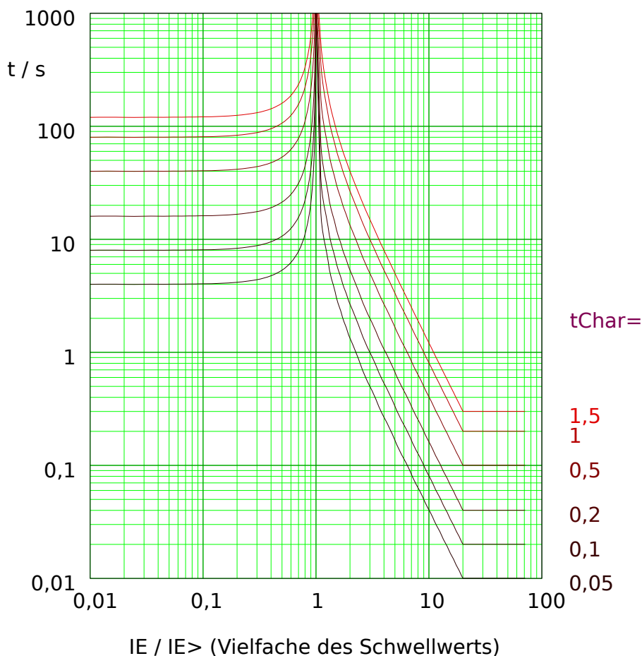
Abb. 73: EINV: Rückfallverzögerung (linke Hälfte, IE < I_{E>} ) und Auslöseverzögerung (rechte Hälfte, IE > I_{E>} ), Beispieldiagramm für I_{max} = 20 \cdot I_{E>} .
