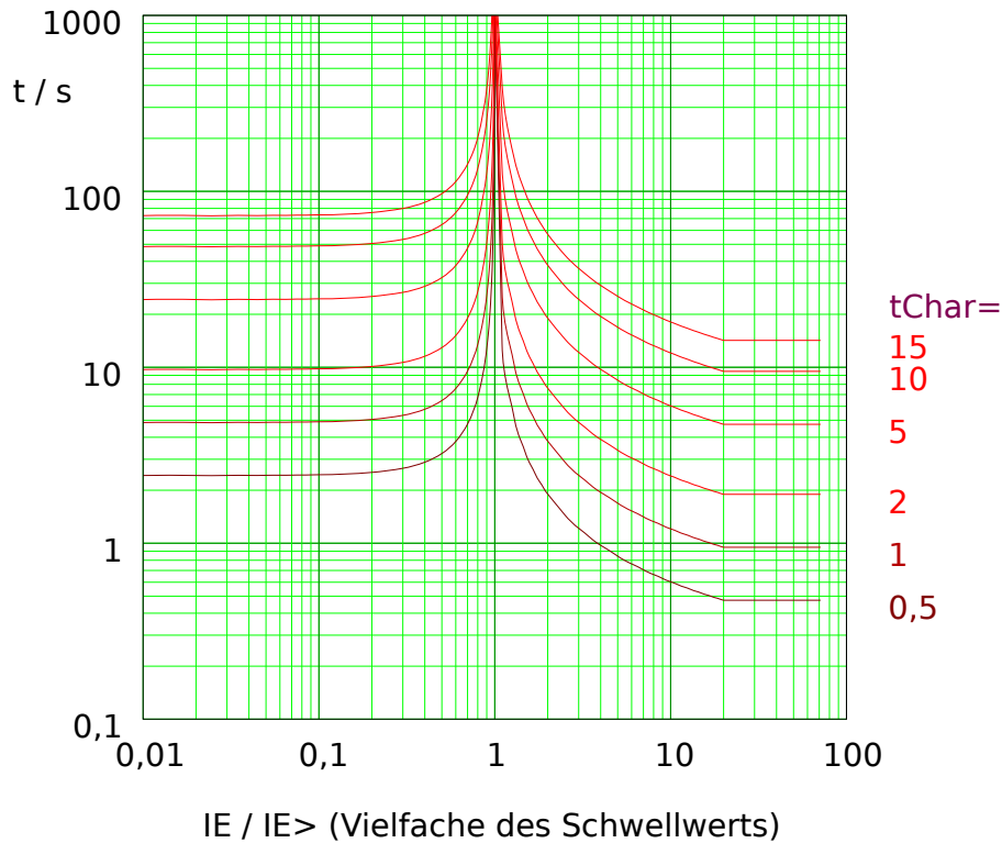
Abb. 76: MINV: Rückfallverzögerung (linke Hälfte, IE < I_{E>} ) und Auslöseverzögerung (rechte Hälfte, IE > I_{E>} ), Beispieldiagramm für I_{max} = 20 \cdot I_{E>} .
