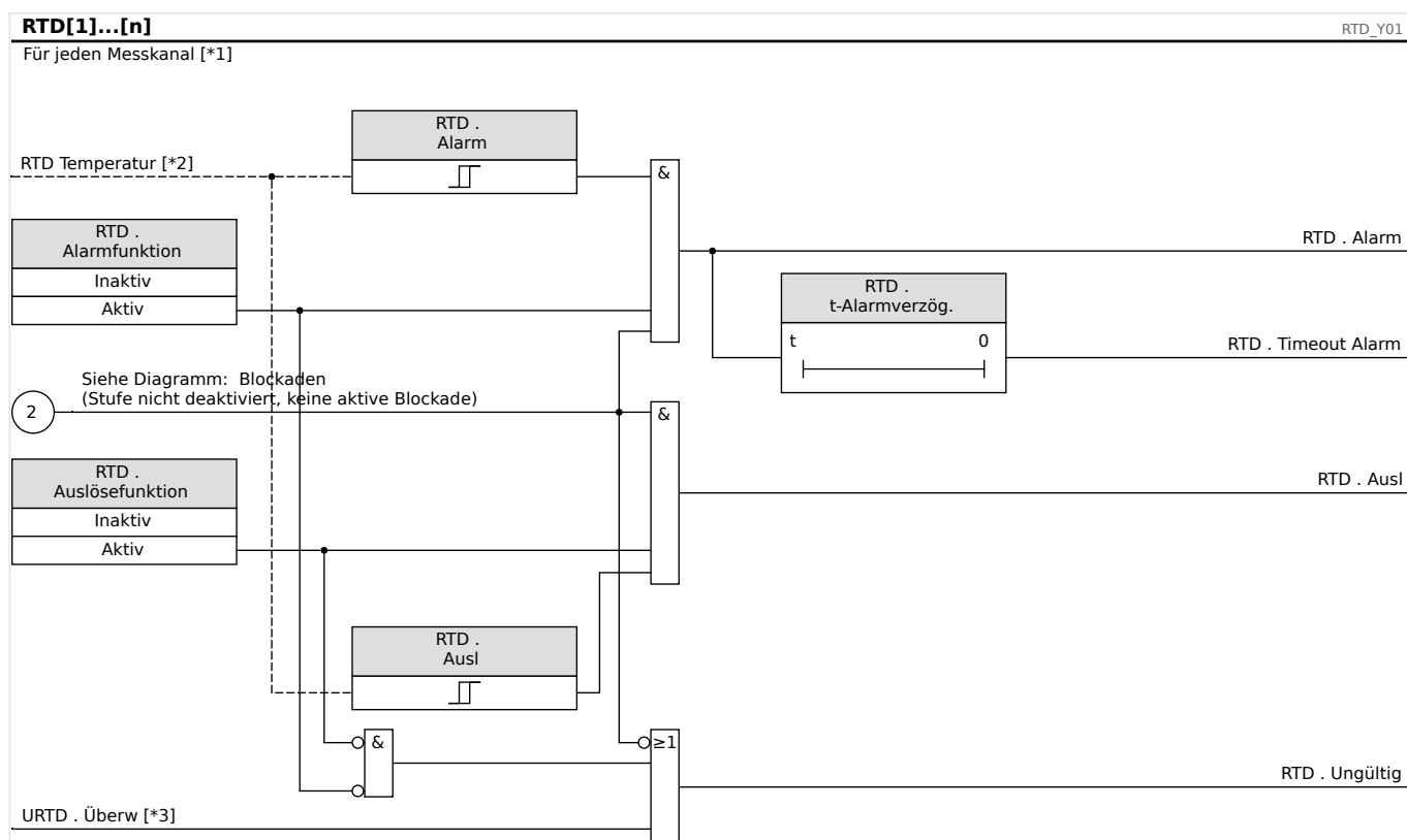
Abb. 89: Generelles RTD-Funktionsprinzip.
