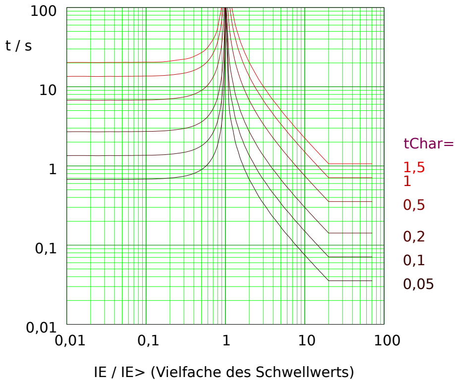
Abb. 72: VINV: Rückfallverzögerung (linke Hälfte, IE < I_{E>} ) und Auslöseverzögerung (rechte Hälfte, IE > I_{E>} ), Beispieldiagramm für I_{max} = 20 \cdot I_{E>} .
