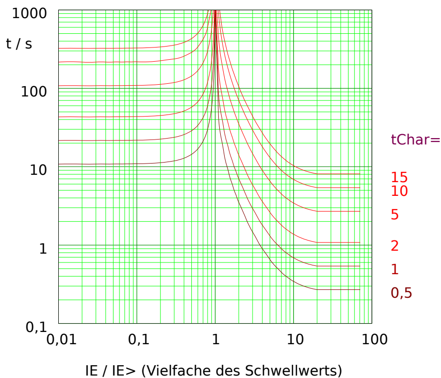
Abb. 77: VINV: Rückfallverzögerung (linke Hälfte, IE < I_{E>} ) und Auslöseverzögerung (rechte Hälfte, IE > I_{E>} ), Beispieldiagramm für I_{max} = 20 \cdot I_{E>} .
