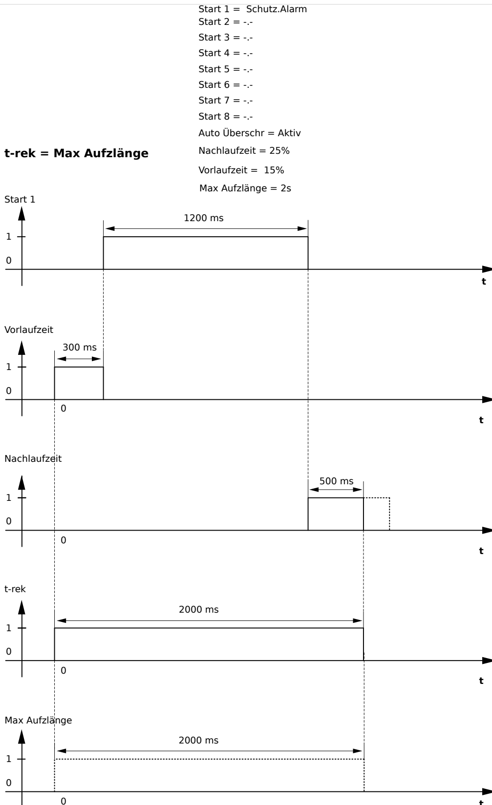
Abb. 102: Beispiel I Störschreiber-Ablaufdiagramm
