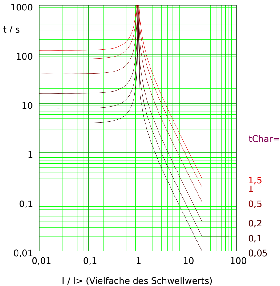
Abb. 61: EINV: Rückfallverzögerung (linke Hälfte, I < I_{>} ) und Auslöseverzögerung (rechte Hälfte, I > I_{>} ), Beispieldiagramm für I_{max} = 20 \cdot I_{>} .
