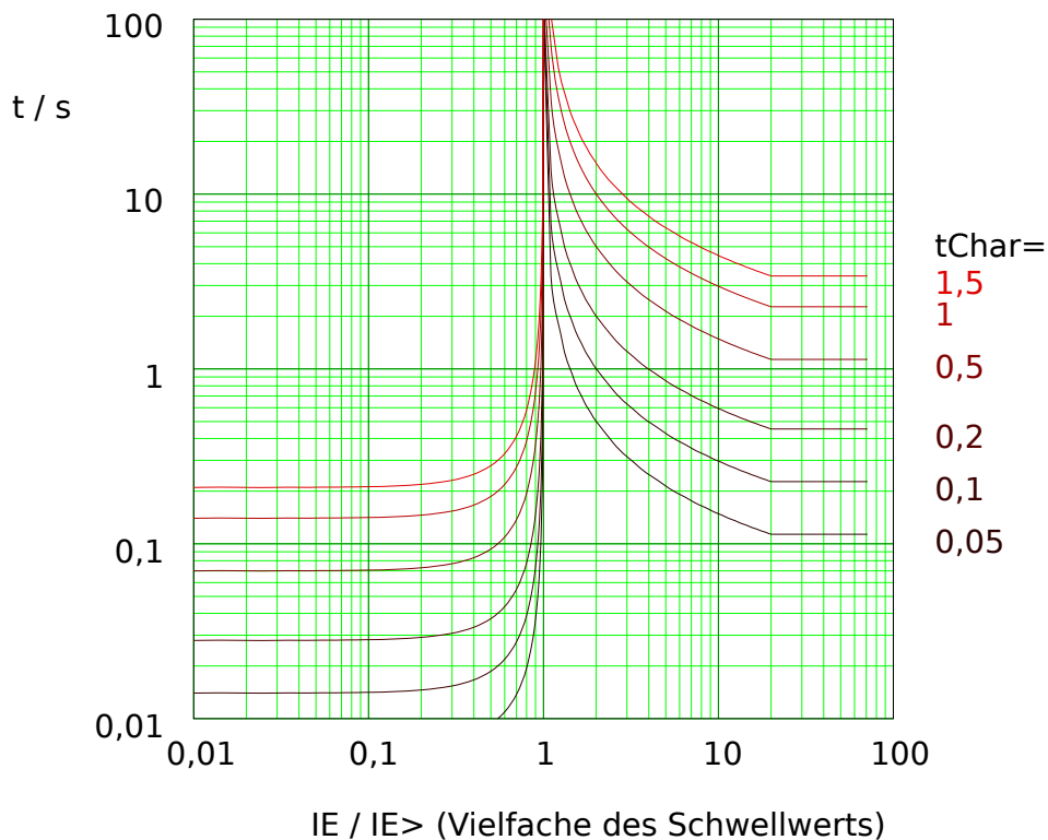
Abb. 71: NINV: Rückfallverzögerung (linke Hälfte, IE < IE> ) und Auslöseverzögerung (rechte Hälfte, IE > IE> ), Beispieldiagramm für I_{max} = 20 \cdot IE> .
