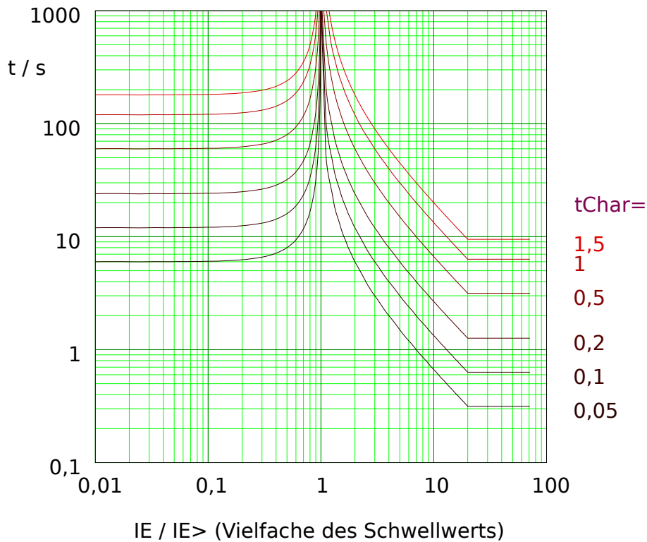
Abb. 74: LINV: Rückfallverzögerung (linke Hälfte, IE < I_{E>} ) und Auslöseverzögerung (rechte Hälfte, IE > I_{E>} ), Beispieldiagramm für I_{max} = 20 \cdot I_{E>} .
