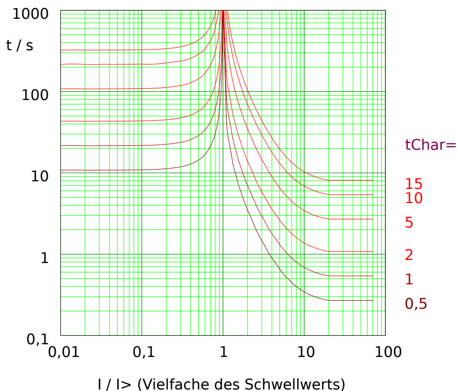
Abb. 71: VINV: Rückfallverzögerung (linke Hälfte, I < I_{>} ) und Auslöseverzögerung (rechte Hälfte, I > I_{>} ), Beispieldiagramm für I_{max} = 20 \cdot I_{>} .
