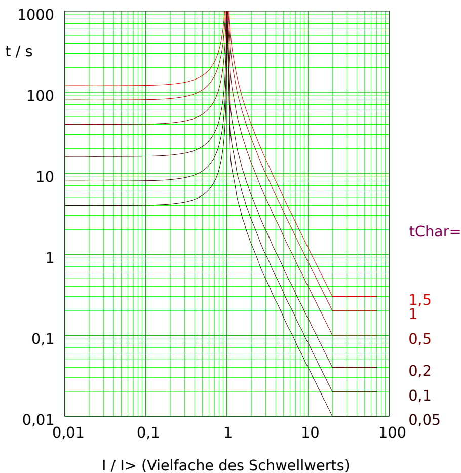
Abb. 67: EINV: Rückfallverzögerung (linke Hälfte, I < I_{>} ) und Auslöseverzögerung (rechte Hälfte, I > I_{>} ), Beispieldiagramm für I_{max} = 20 \cdot I_{>} .
