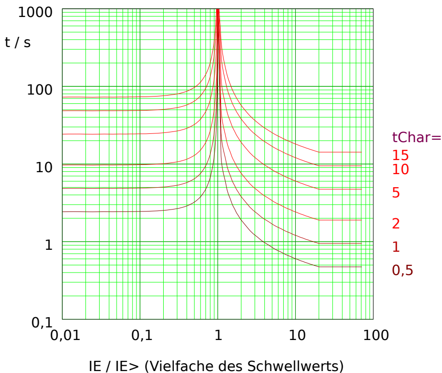
Abb. 82: MINV: Rückfallverzögerung (linke Hälfte, IE < I_{E>} ) und Auslöseverzögerung (rechte Hälfte, IE > I_{E>} ), Beispieldiagramm für I_{max} = 20 \cdot I_{E>} .
