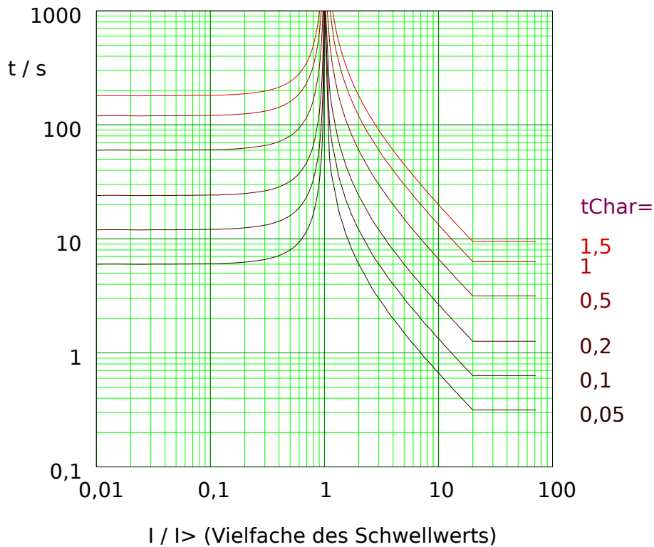
Abb. 68: LINV: Rückfallverzögerung (linke Hälfte, I < I_{>} ) und Auslöseverzögerung (rechte Hälfte, I > I_{>} ), Beispieldiagramm für I_{max} = 20 \cdot I_{>} .
