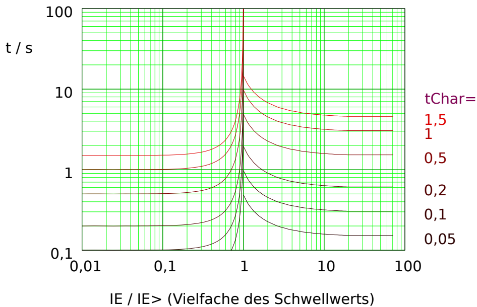
Abb. 81: RINV: Rückfallverzögerung (linke Hälfte, IE < I_{E>} ) und Auslöseverzögerung (rechte Hälfte, IE > I_{E>} ), Beispieldiagramm für I_{max} = 20 \cdot I_{E>} .
