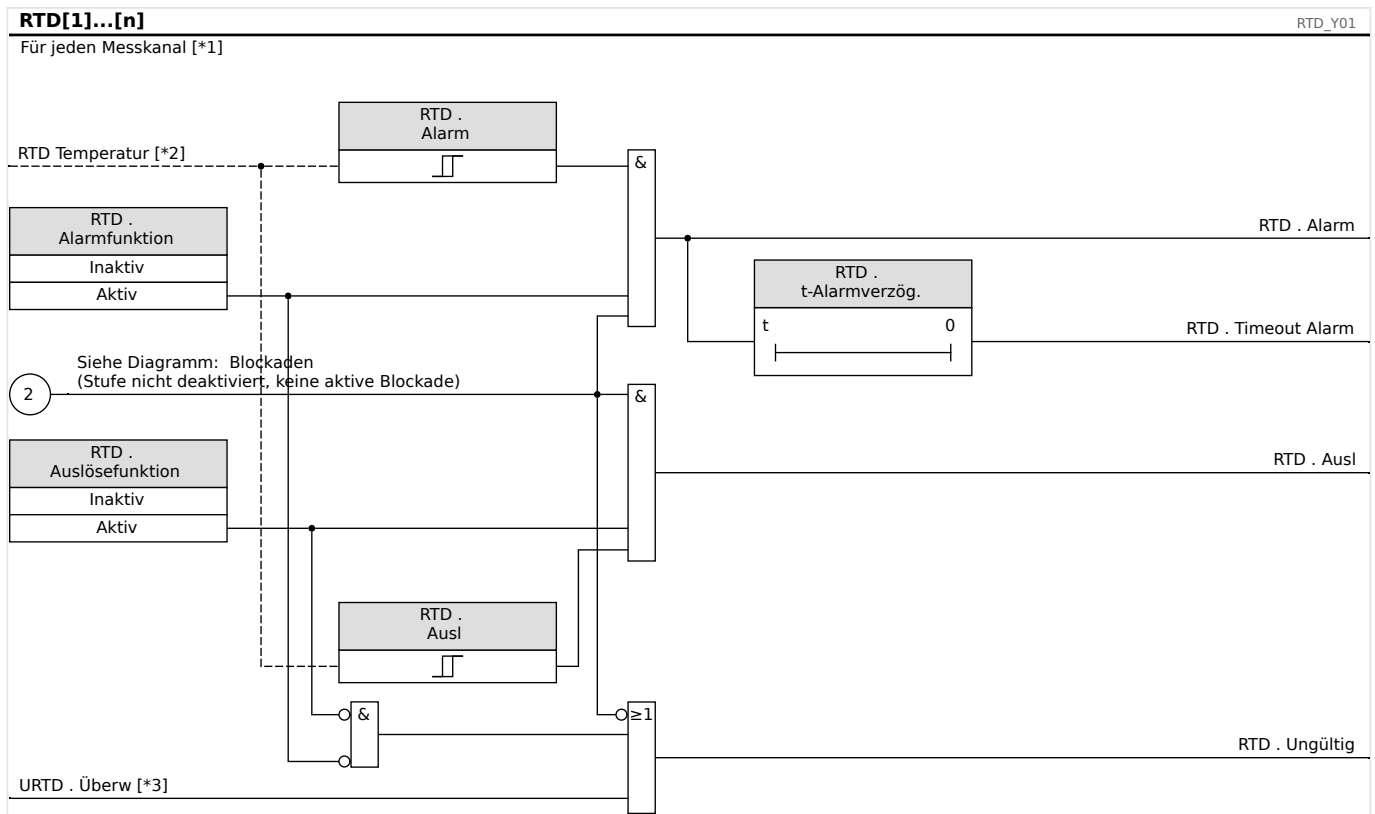
Abb. 95: Generelles RTD-Funktionsprinzip.
