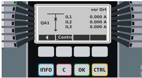
Abb. 100: Beispiel einer Steuer-Seite mit geschlossenem „Leistungsschalter“.
