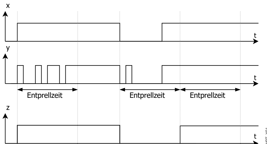
Abb. 45: Entprell-Mechanismus des MRDT4.
