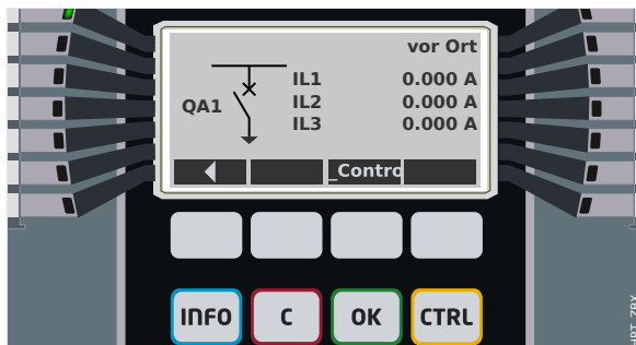
Abb. 102: Beispiel einer Steuer-Seite mit geöffnetem „Leistungsschalter“.
