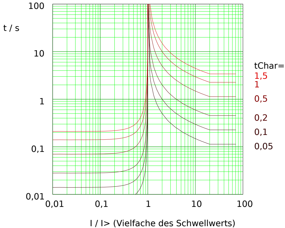
Abb. 65: NINV: Rückfallverzögerung (linke Hälfte, I < I_{>} ) und Auslöseverzögerung (rechte Hälfte, I > I_{>} ), Beispieldiagramm für I_{max} = 20 \cdot I_{>} .
