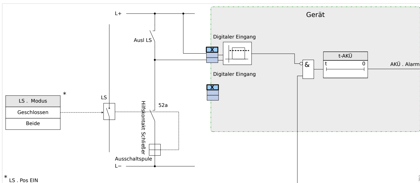
Abb. 97: Anschlussbeispiel: Auslösekreisüberwachung mit einem Hilfskontakt »Hiko EIN« (52a).
