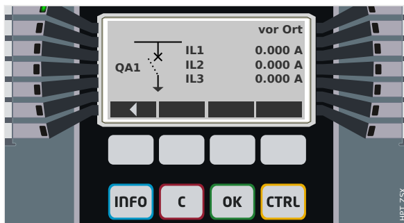
Abb. 99: Beispiel einer Steuer-Seite mit „Leistungsschalter“ in Zwischenposition).
