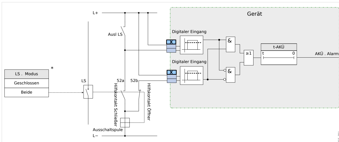
Abb. 96: Anschlussbeispiel (Empfehlung): Auslösekreisüberwachung mit zwei Hilfskontakten »Hiko EIN« (52a) und »Hiko AUS« (52b).
