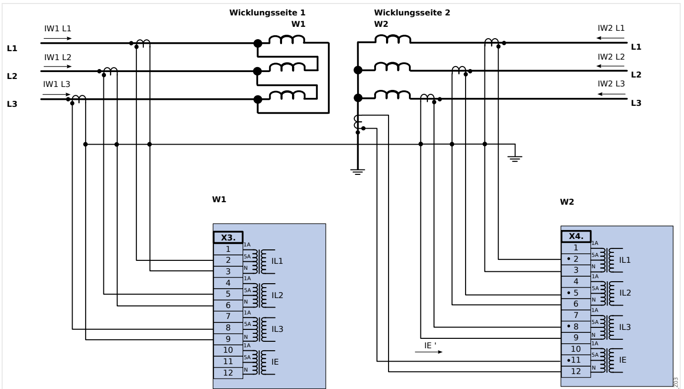
Dreiphasiger Stromwandleranschluss; In sekundär = 5 A.
