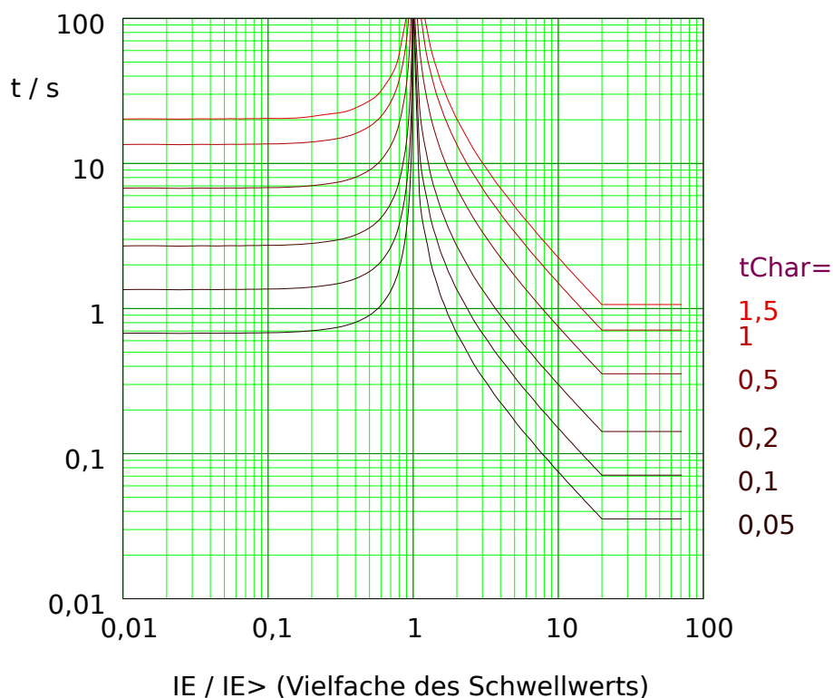
Abb. 78: VINV: Rückfallverzögerung (linke Hälfte, IE < IE_{>} ) und Auslöseverzögerung (rechte Hälfte, IE > IE_{>} ), Beispieldiagramm für I_{max} = 20 \cdot IE_{>} .
