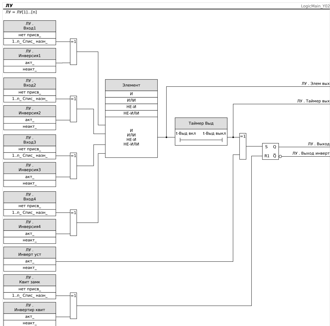
Рис. 83: Подробный обзор — общая логическая схема.
