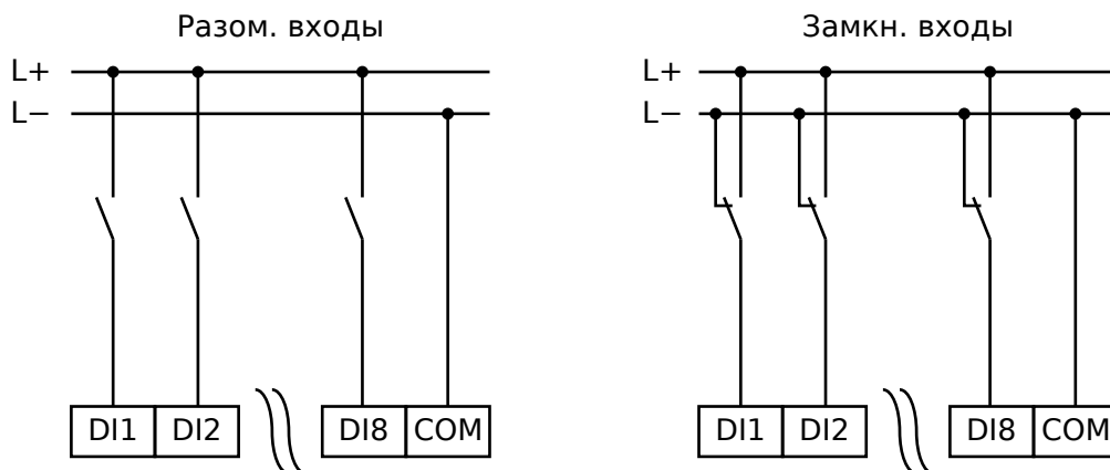
Рис. 90: Безопасное состояние цифровых входов
