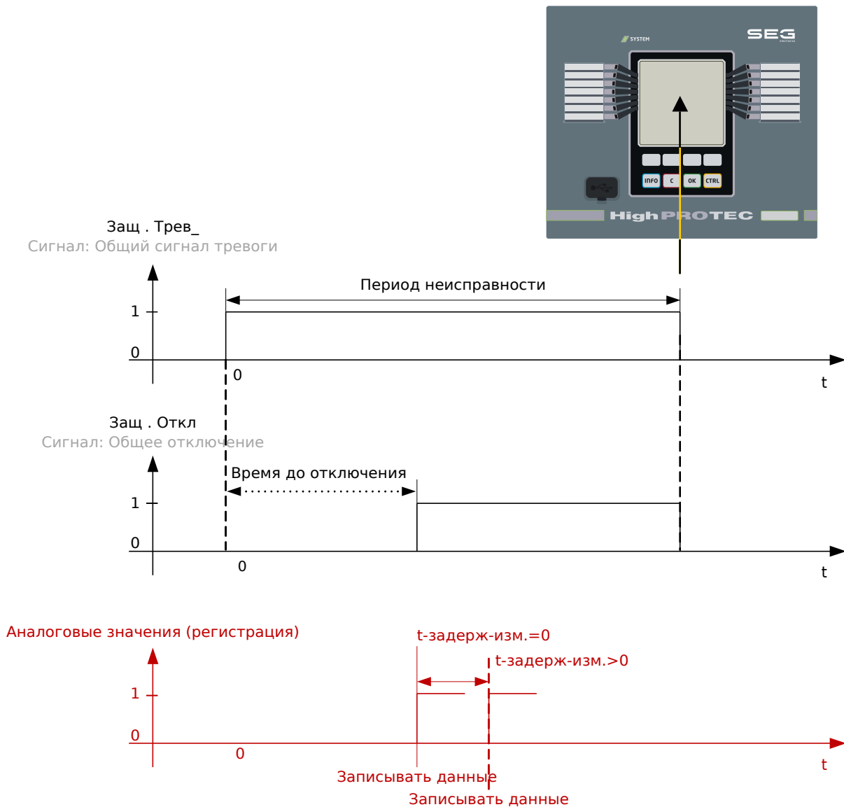
Рис. 81: Регистратор неисправностей: время и длительность.
