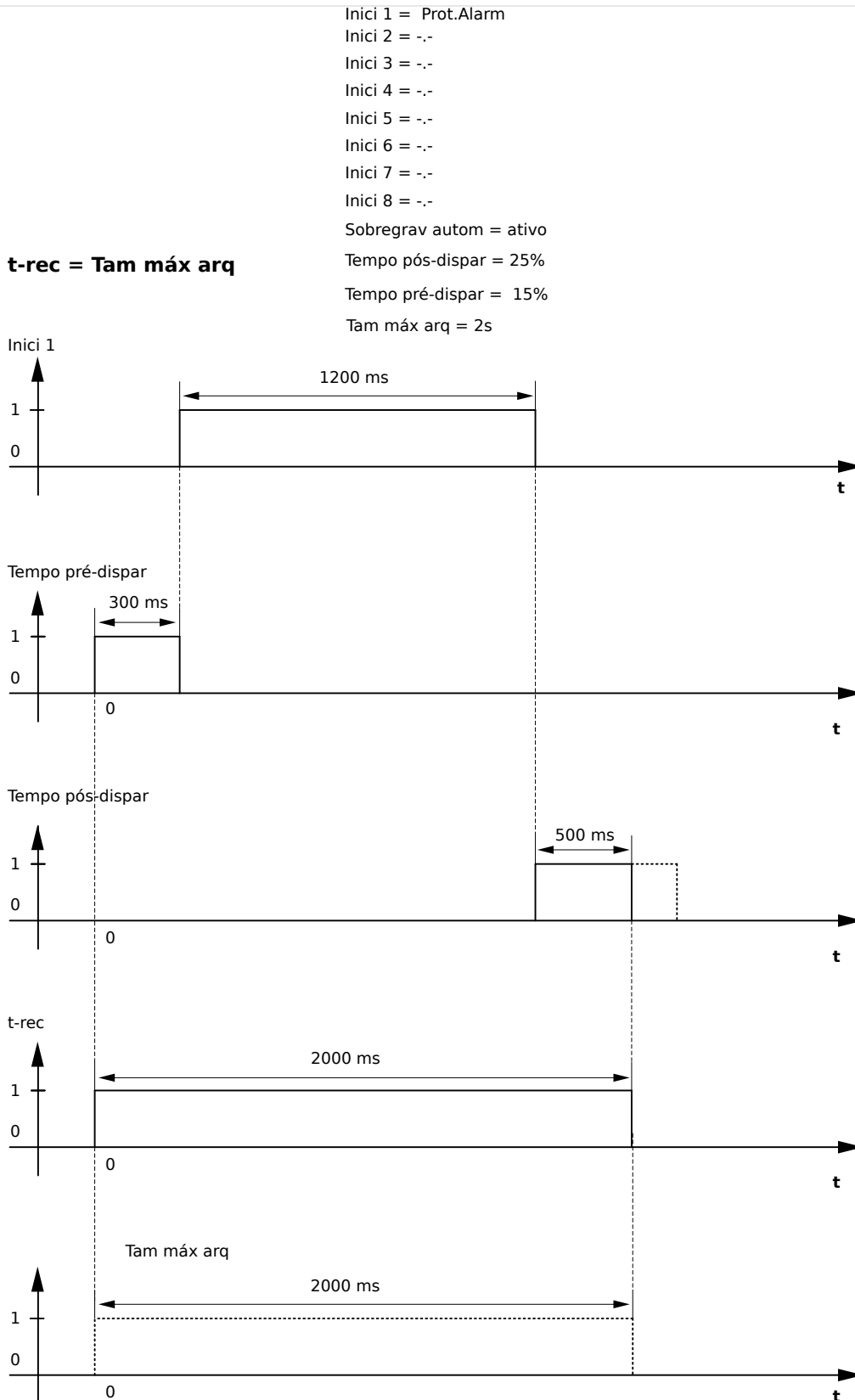
Fig. 79: Exemplo de Gráfico de Prazo do Gravador de Perturbação I
