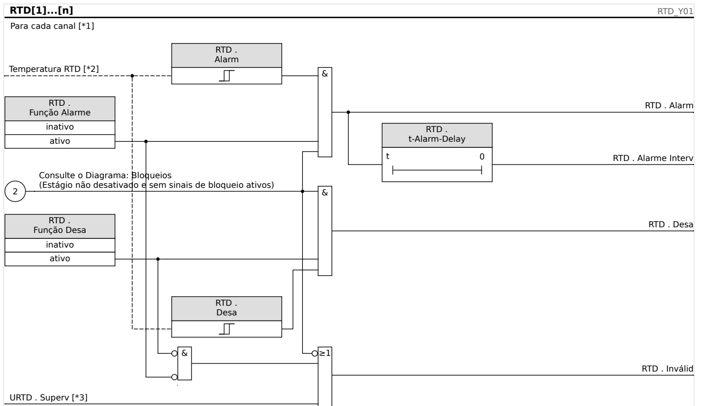
Fig. 67: O princípio geral de funcionamento (alarme atrasado, disparo sem atraso).
