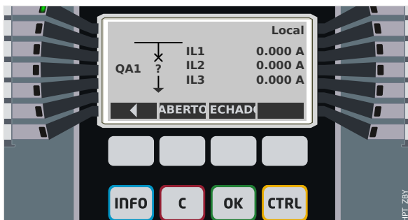
Fig. 72: Exemplo de página de controle, com o "Disjuntor" na posição de falha (ou implausível).
