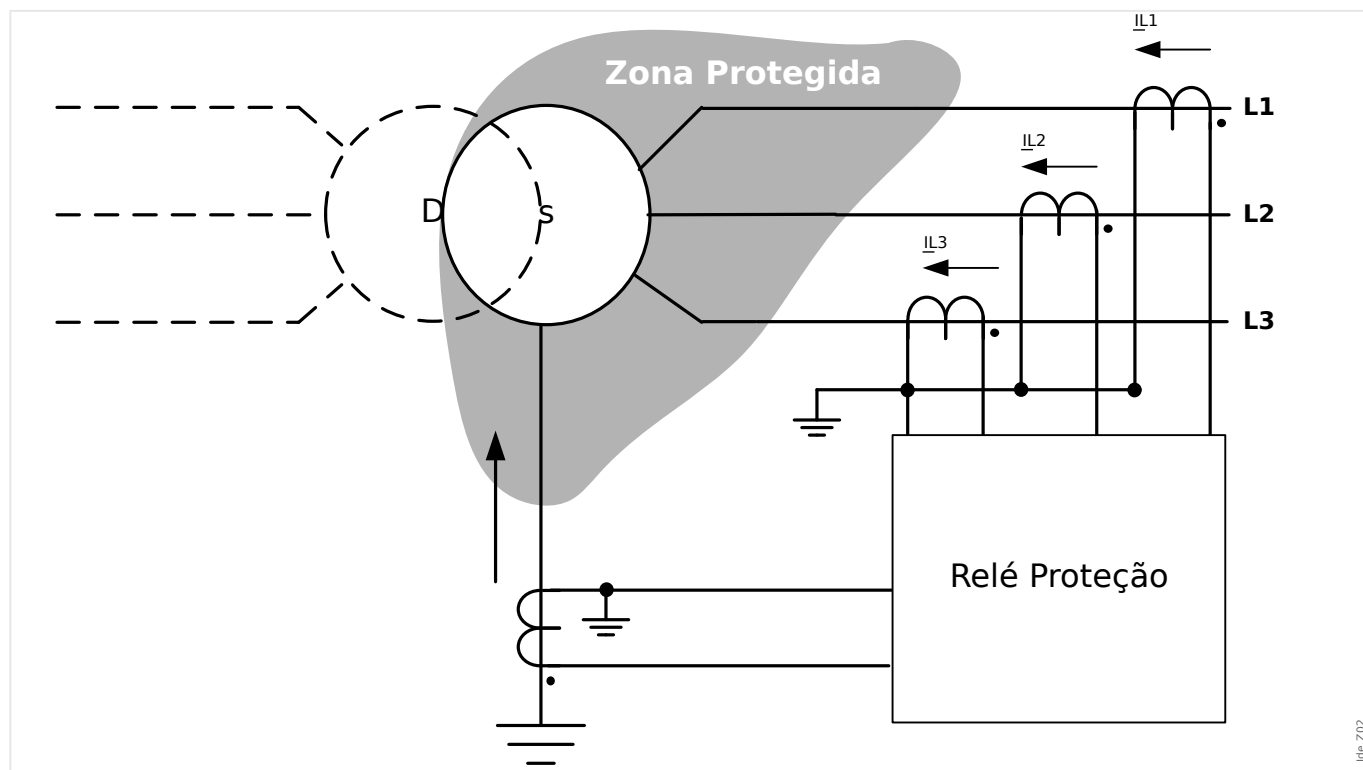
Fig. 52: Princípio de Proteção da Proteção Diferencial de Corrente de Aterramento no enrolamento lateral wye do transformador.
