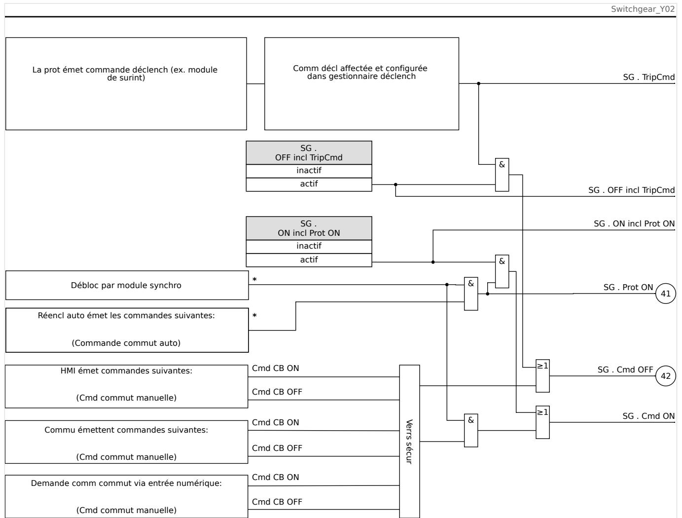
Fig. 74: Verrouillages (Parties identifiées par « * » : la disponibilité dépend du type de dispositif commandé.)
