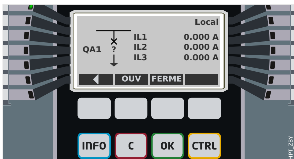
Fig. 72: Exemple de page de contrôle, avec le « disjoncteur » en position de dysfonctionnement (ou invraisemblable).
