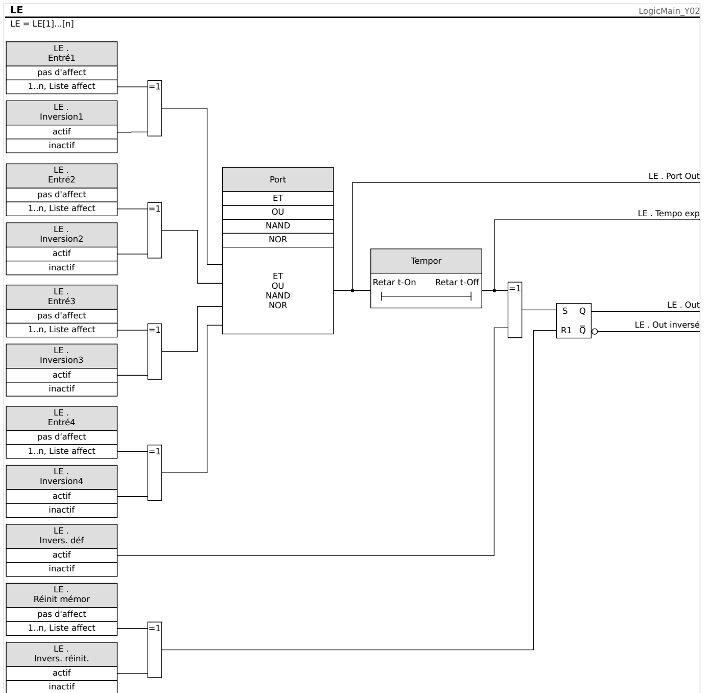
Fig. 83: Présentation détaillée - Diagramme logique global.
