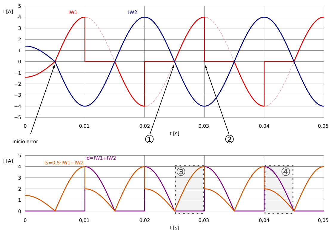
Fig. 50: Característica de I_d e I_s con saturación en el lado W1 del CT en caso de fallo externo.
