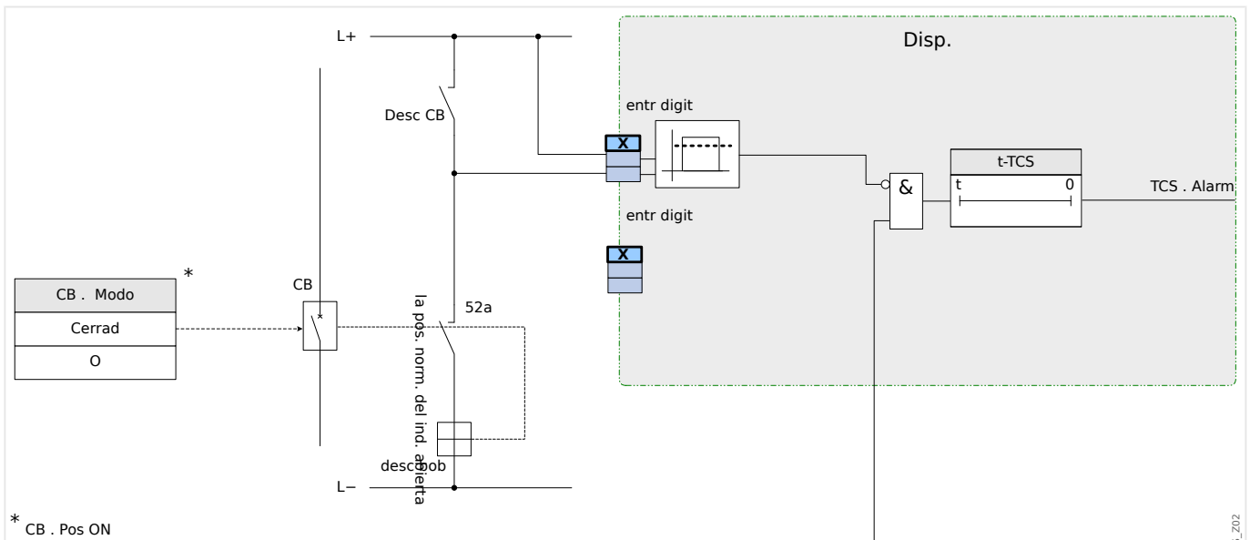
Fig. 69: Ejemplo de conexión: Supervisión del circuito de desconexión solo con un contacto auxiliar CB »Aux ON« (52a).
