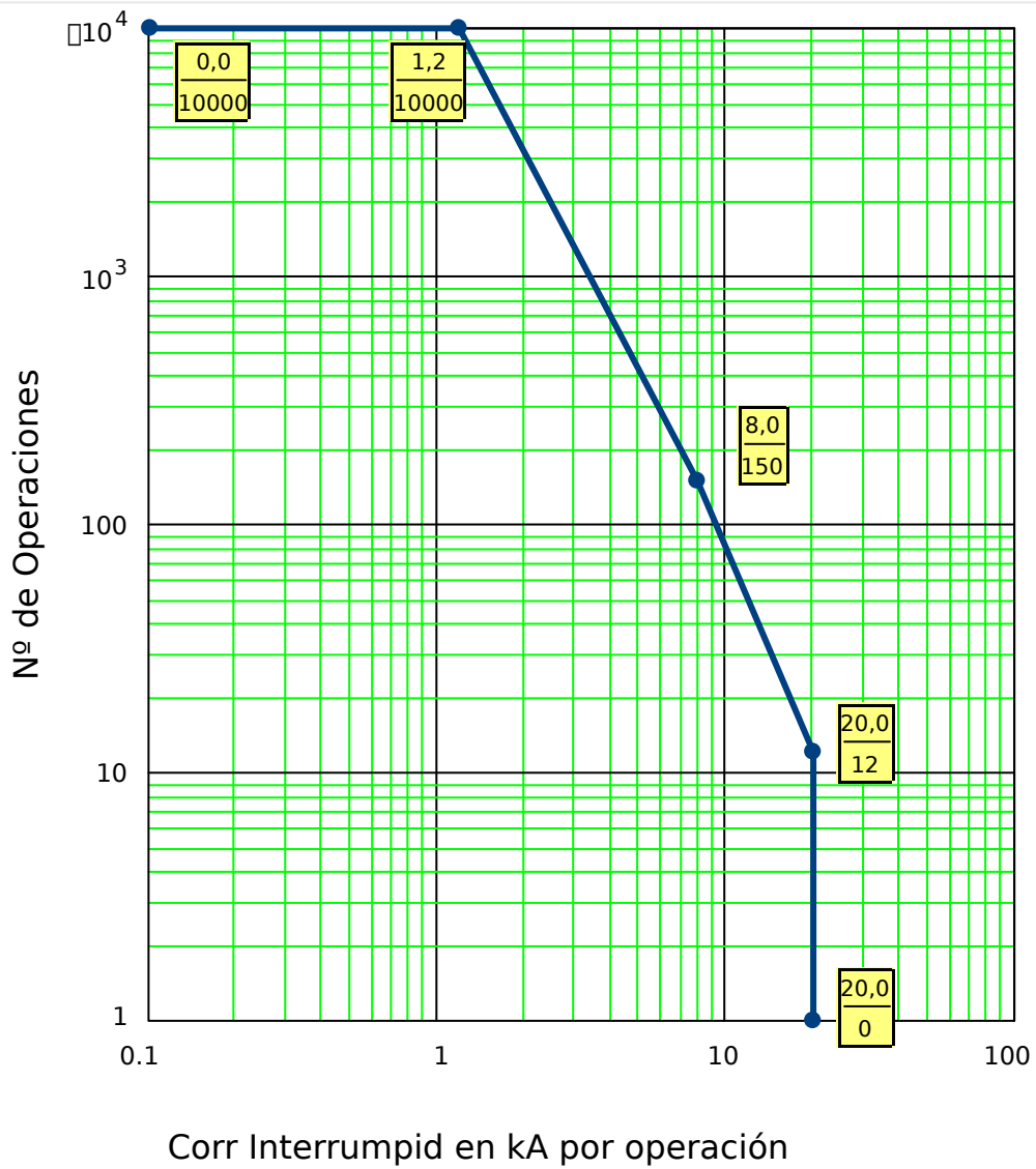
Fig. 76: Curva Mantenim Interruptor para Interrupt Circuito típico 25kV
