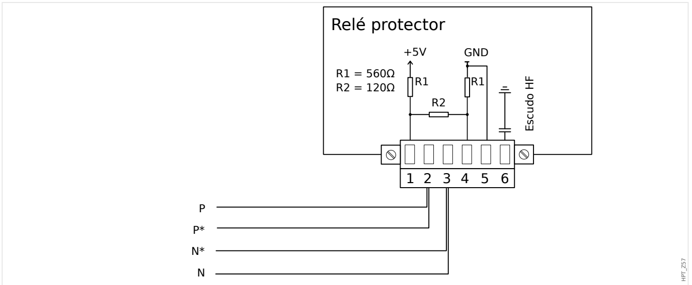
Fig. 31: Ejemplo de cableado, dispositivo en el medio de BUS
