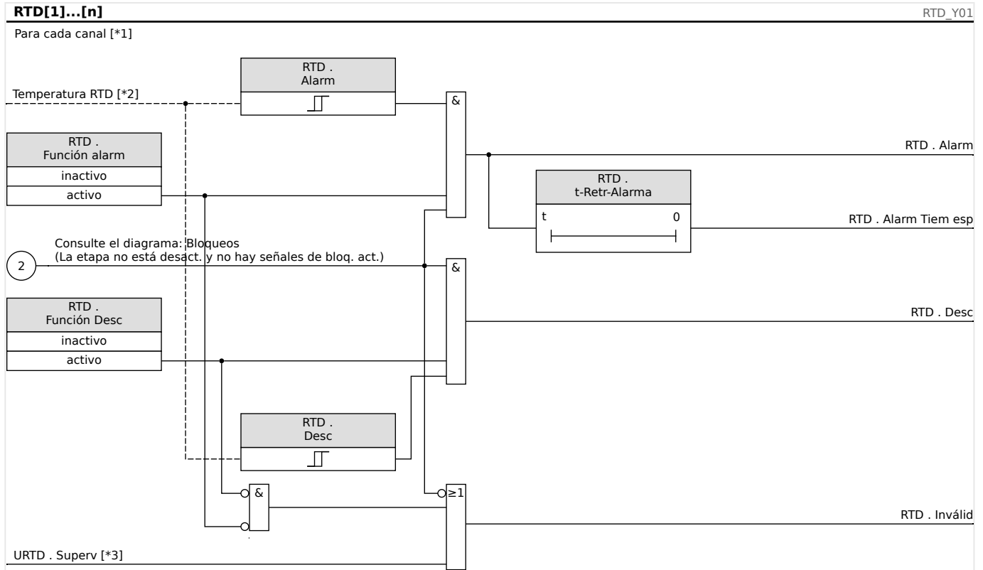
Fig. 67: El principio de funcionamiento general (alarma retrasada, desconexión sin retraso).
