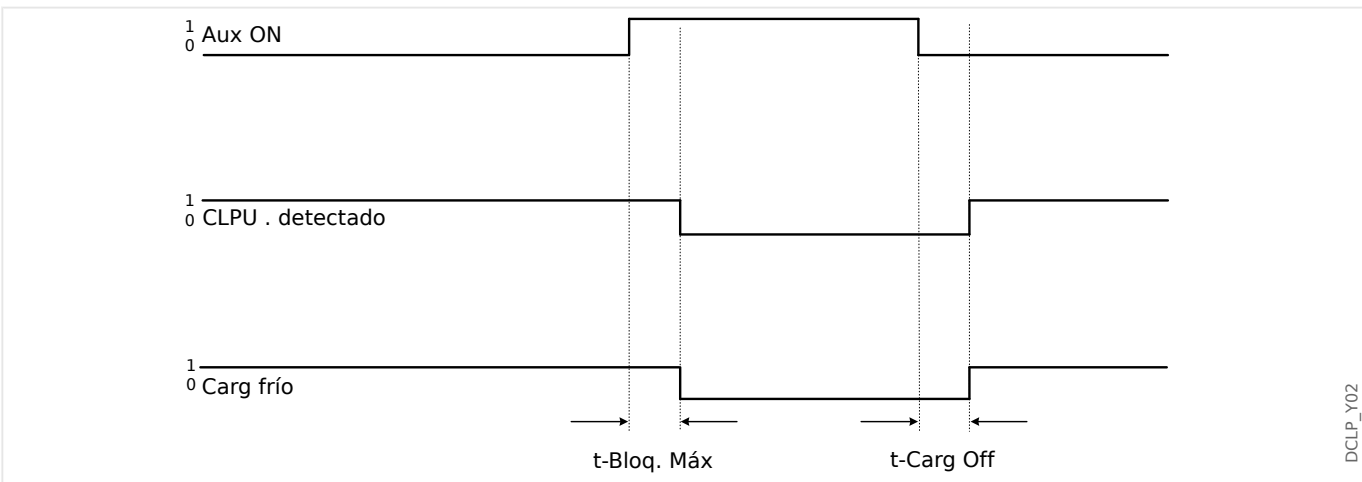
Fig. 65: Modo de ejemplo: Posición de interruptor.
