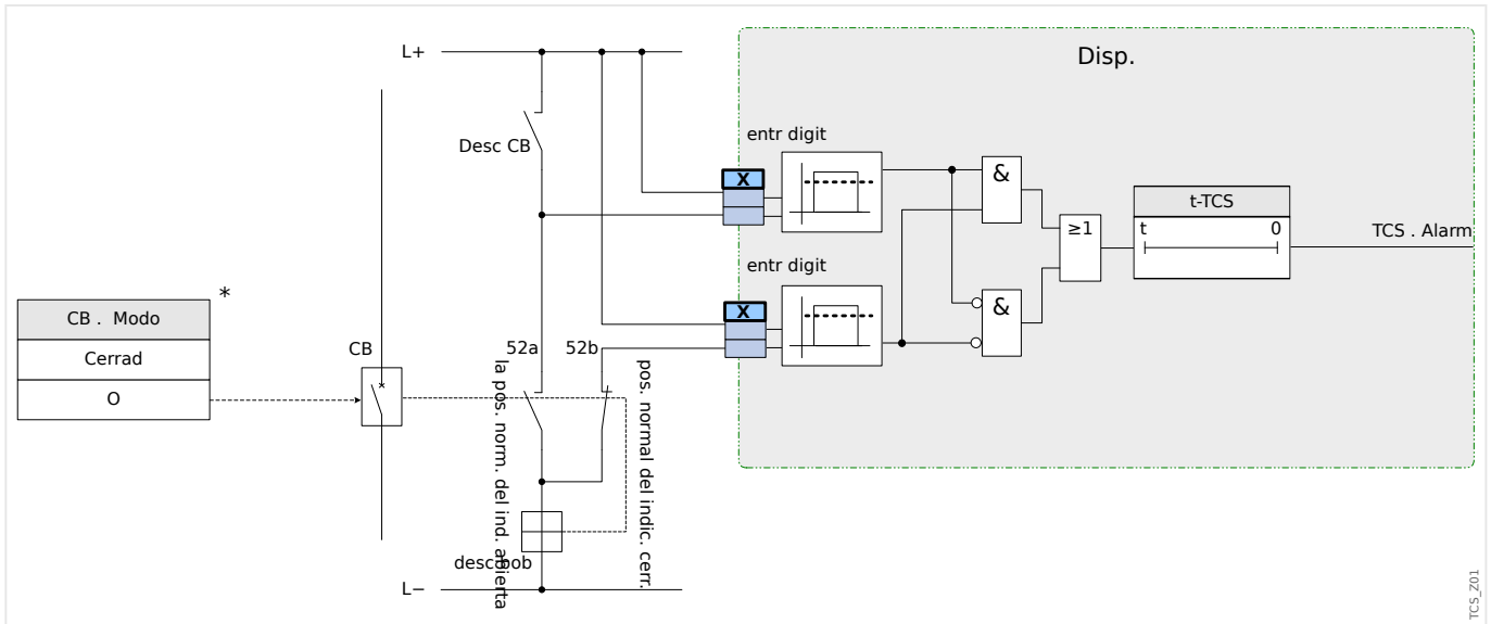
Fig. 68: Ejemplo de conexión: Supervisión del circuito de desconexión con dos contactos auxiliares CB »Aux ON« (52a) and »Aux OFF« (52b).
