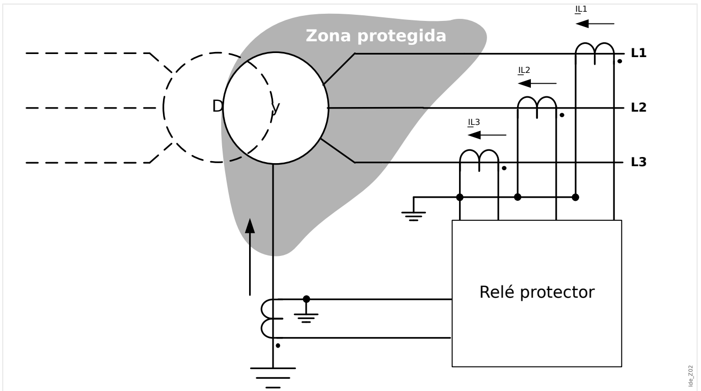
Fig. 52: Principio de protección de la protección de diferencial de corriente de tierra conectada al bobinado del lado wye del transformador
