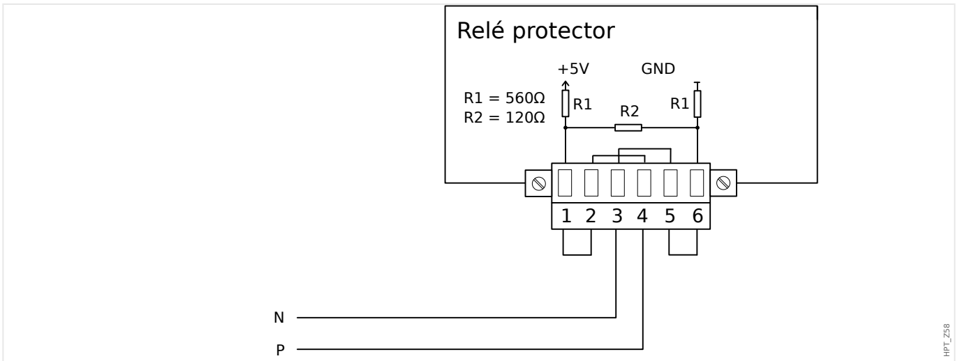
Fig. 32: Ejemplo de cableado, dispositivo en el final de BUS (ajuste de puentes de cable para activar el resistor de terminal integrado)
