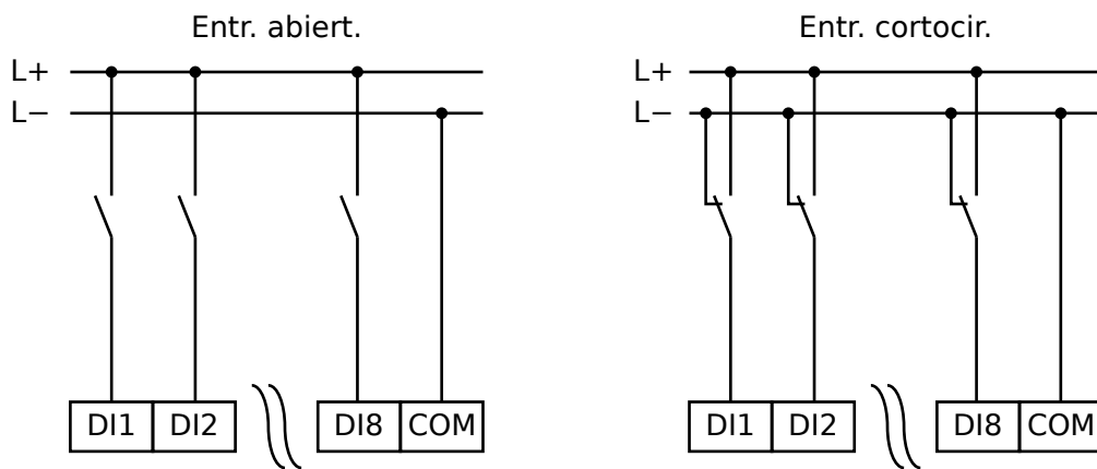
Fig. 90: Estado seguro de entradas digitales
