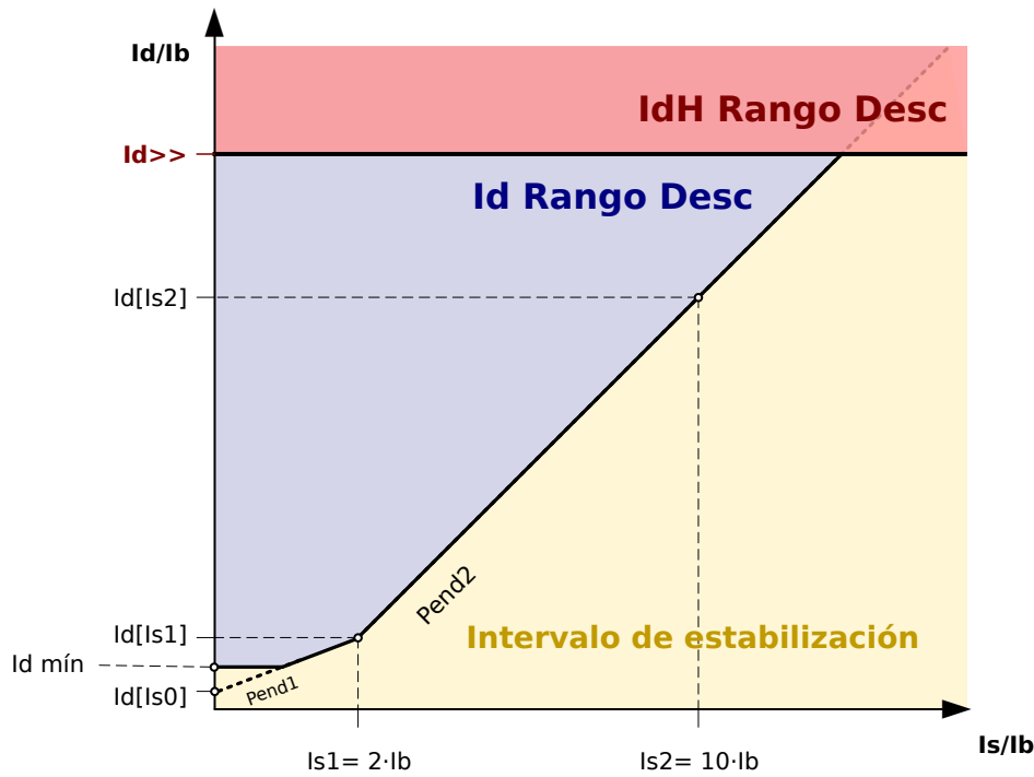
Fig. 51: Paso de protección de diferencial de ajuste alto no limitado I_{dH} .
