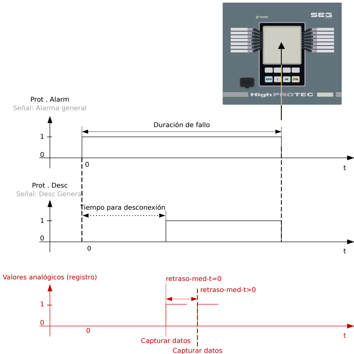
Fig. 81: Registrador de fallos: tiempos y duraciones.
