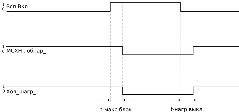
Рис. 57: Пример: Положение выключателя.
