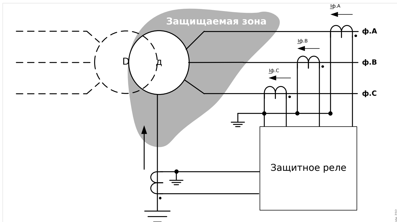
Рис. 52: Принцип работы дифференциальной токовой защиты обмоток трансформаторов, соединенных по схеме «звезда».
