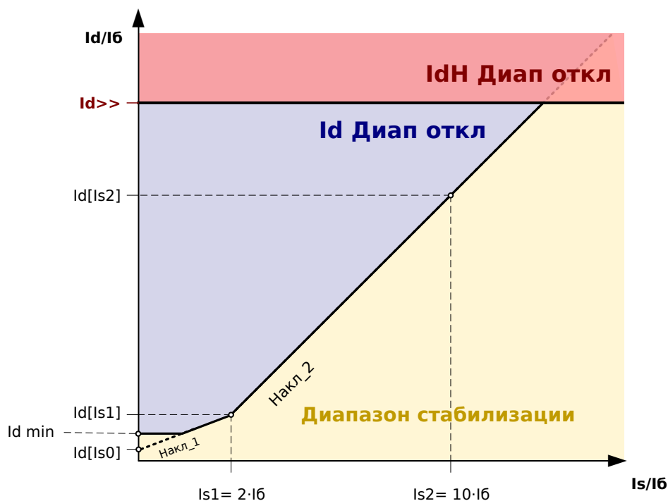
Рис. 51: Этап неограниченной дифференциальной защиты с высокой уставкой IdH.
