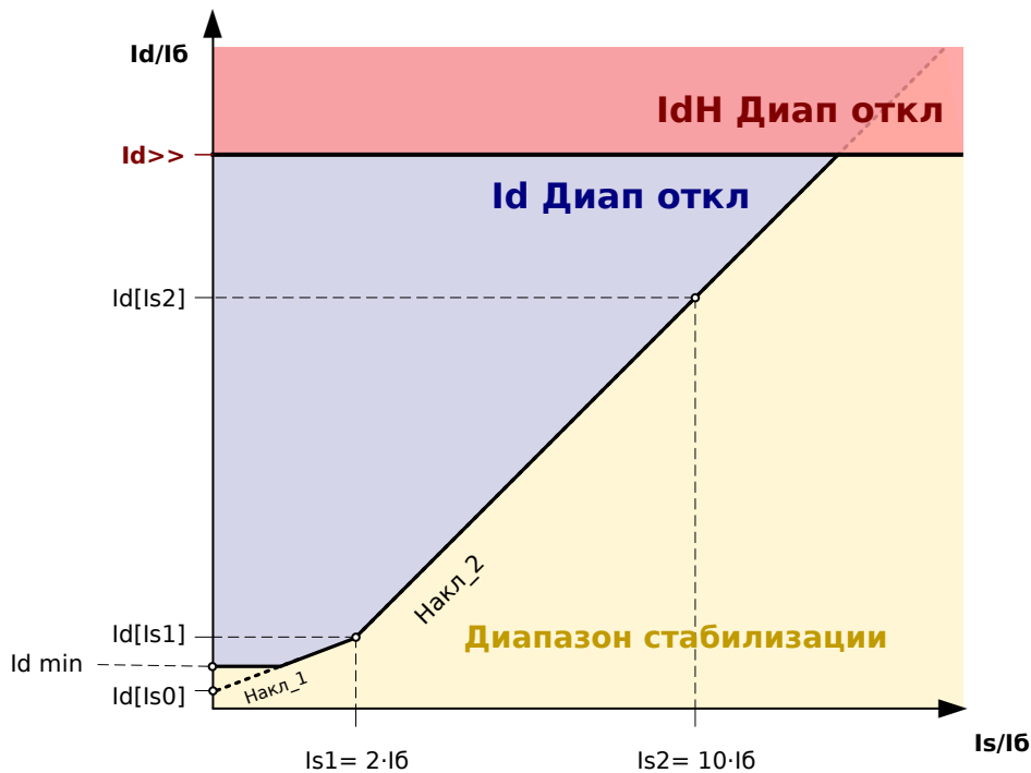
Рис. 48: Кривые отключения защитных функций «Id» (область синего цвета) и «IdH» (область красного цвета).
