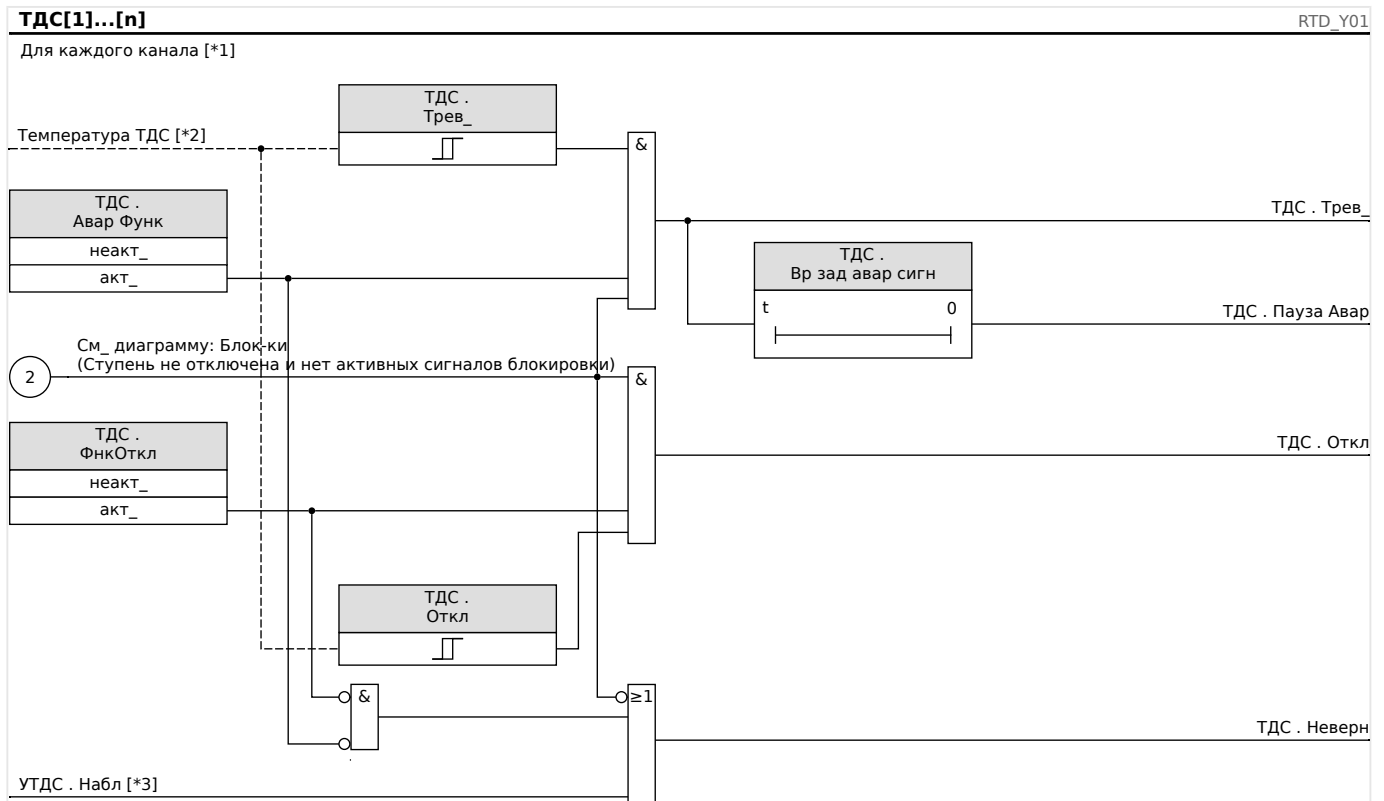
Рис. 59: Общий принцип работы (аварийный сигнал с задержкой, отключение без задержки).
