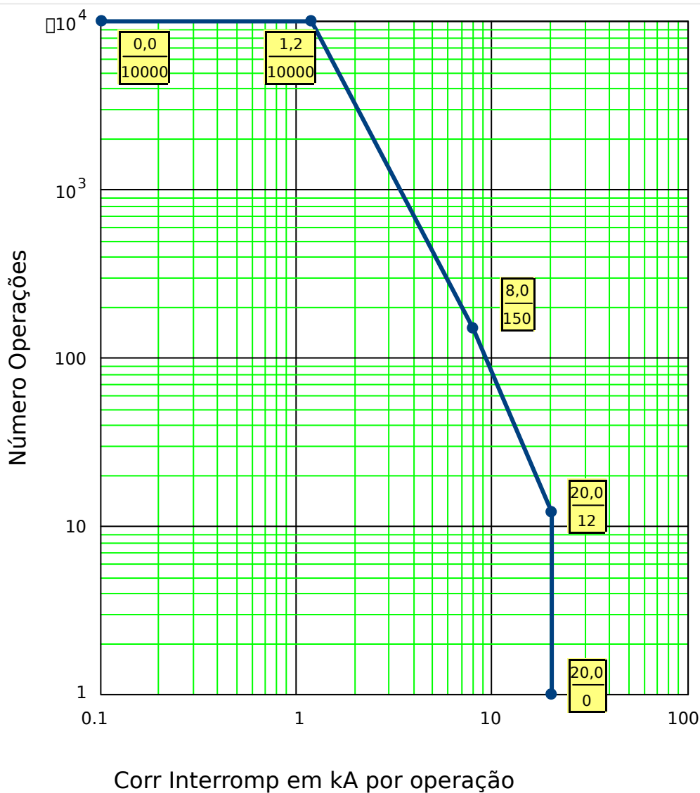
Fig. 68: Curva Manutenção de Disjuntor para Disjuntor normal 25kV
