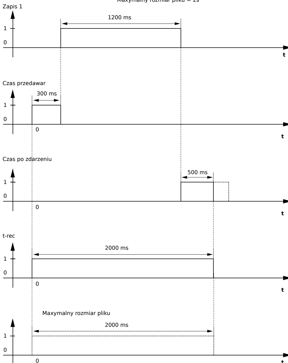
Rys. 71: Przykładowy wykres czasów pracy rejestratora zakłóceń I
