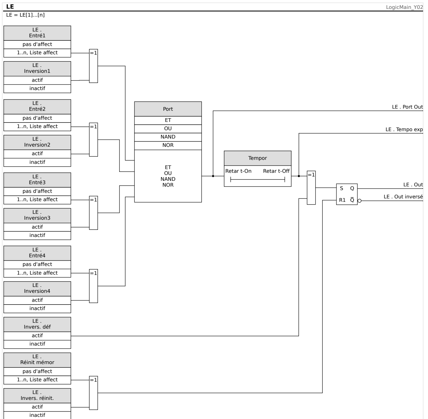
Fig. 75: Présentation détaillée - Diagramme logique global.
