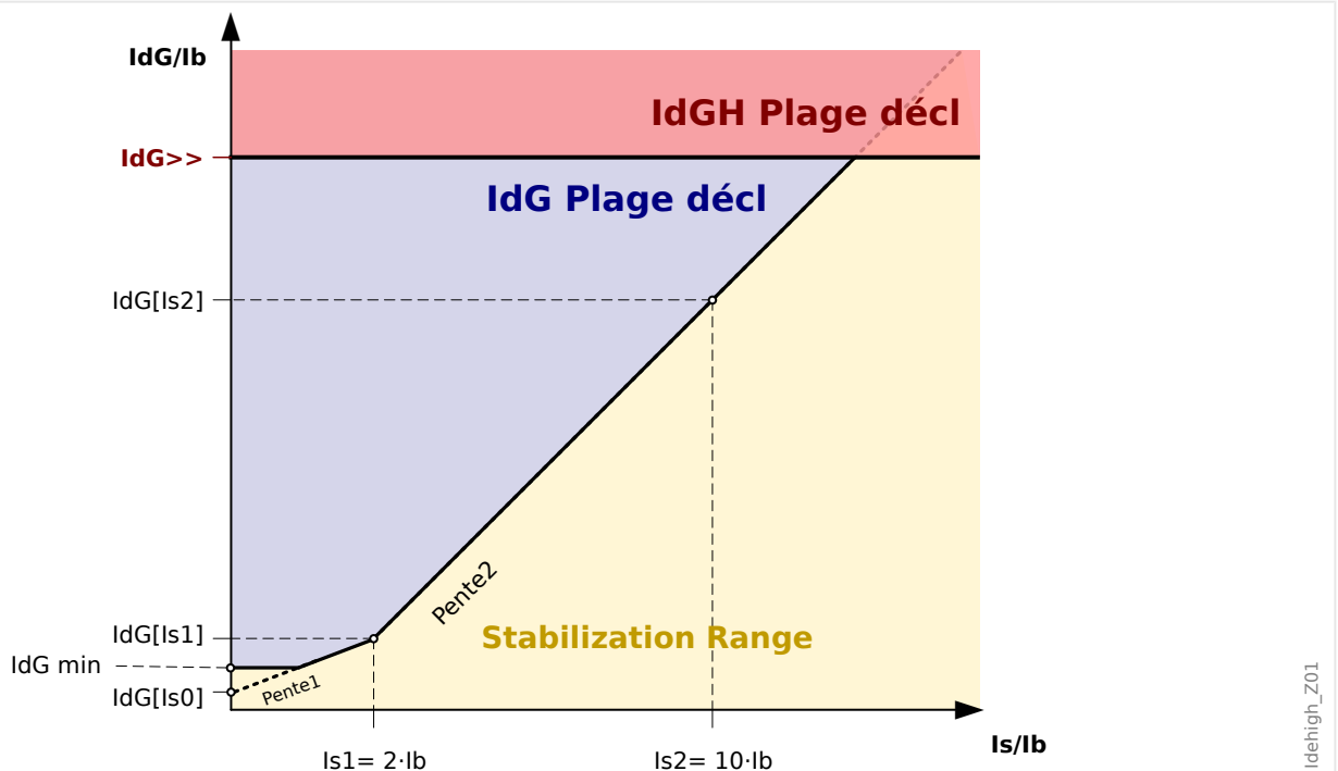
Fig. 53: Valeur d'excitation « I_{dG} » du courant différentiel à la terre en fonction du courant nominal « I_b » de l'objet de protection associé.
