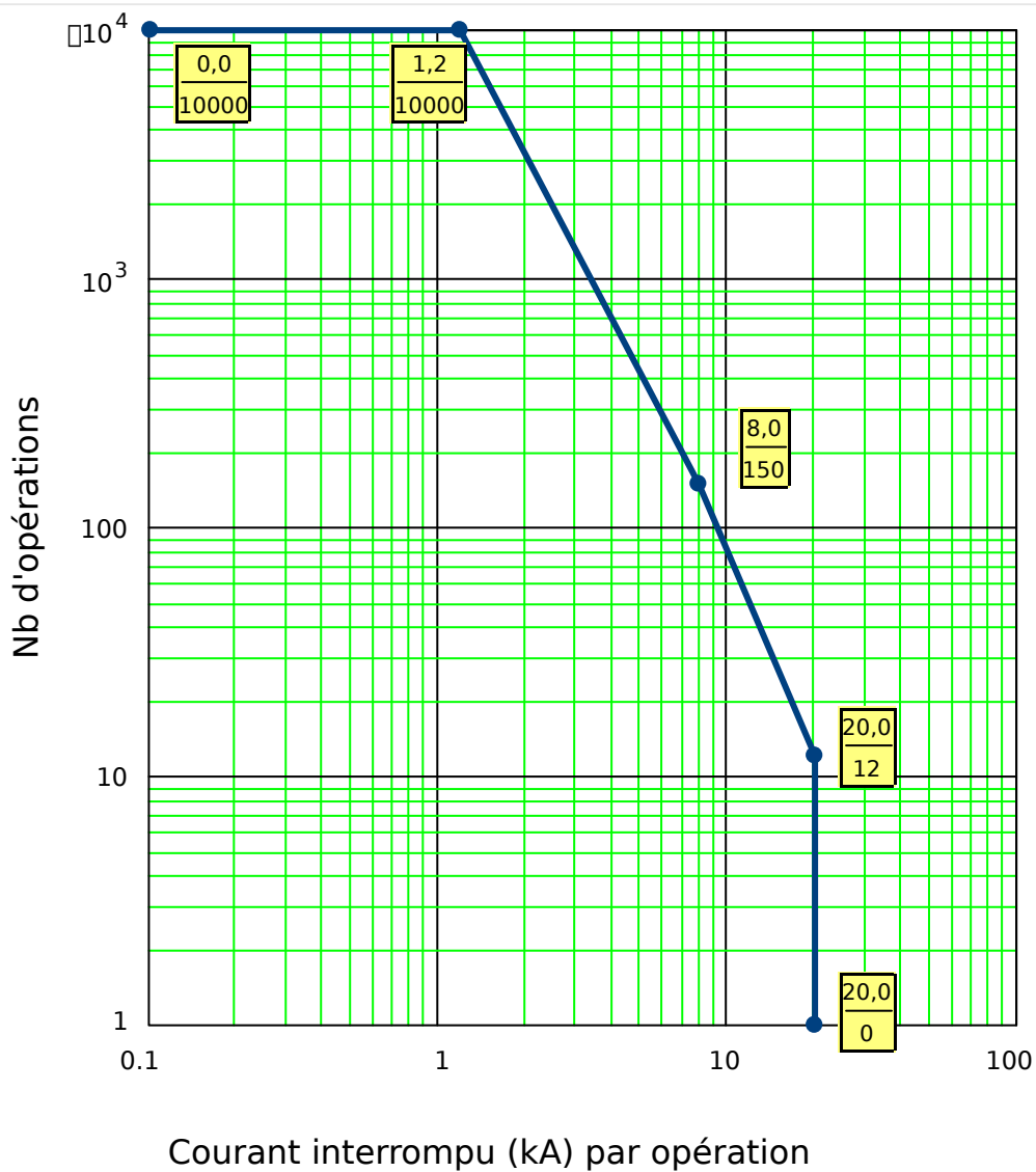
Fig. 68: Courbe de maintenance du disj pour un disj 25 ~kV typique
