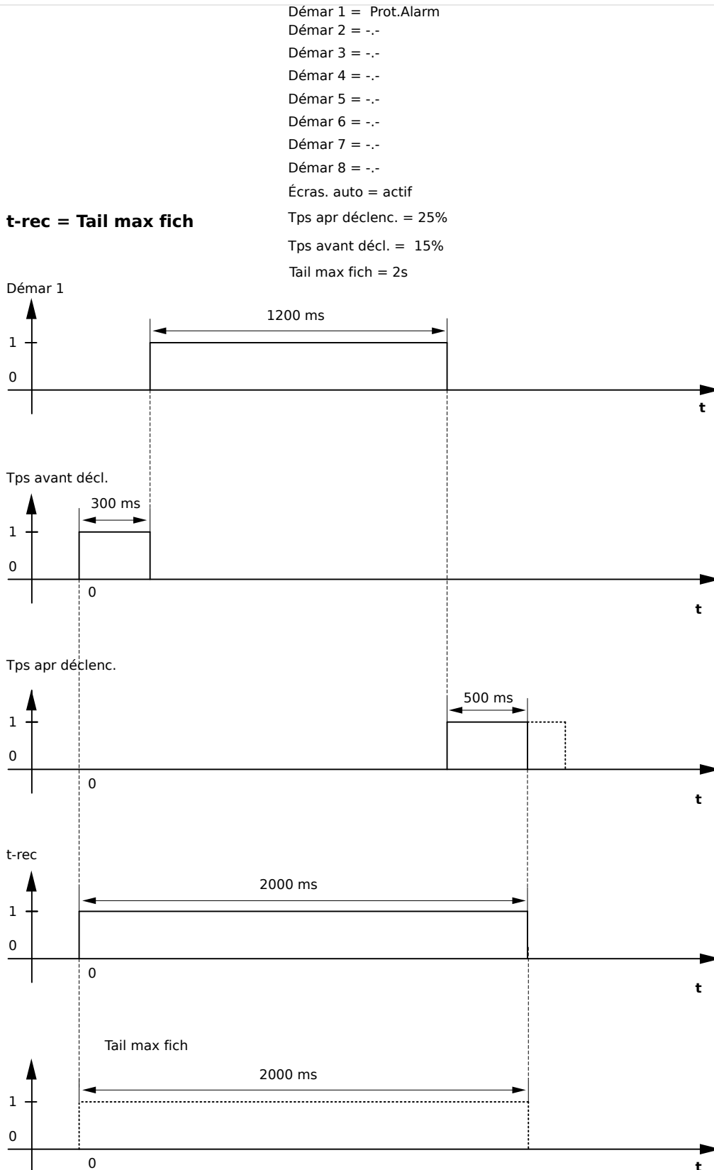
Fig. 71: Exemple de diagramme des temps de l'enregistreur de perturbations I
