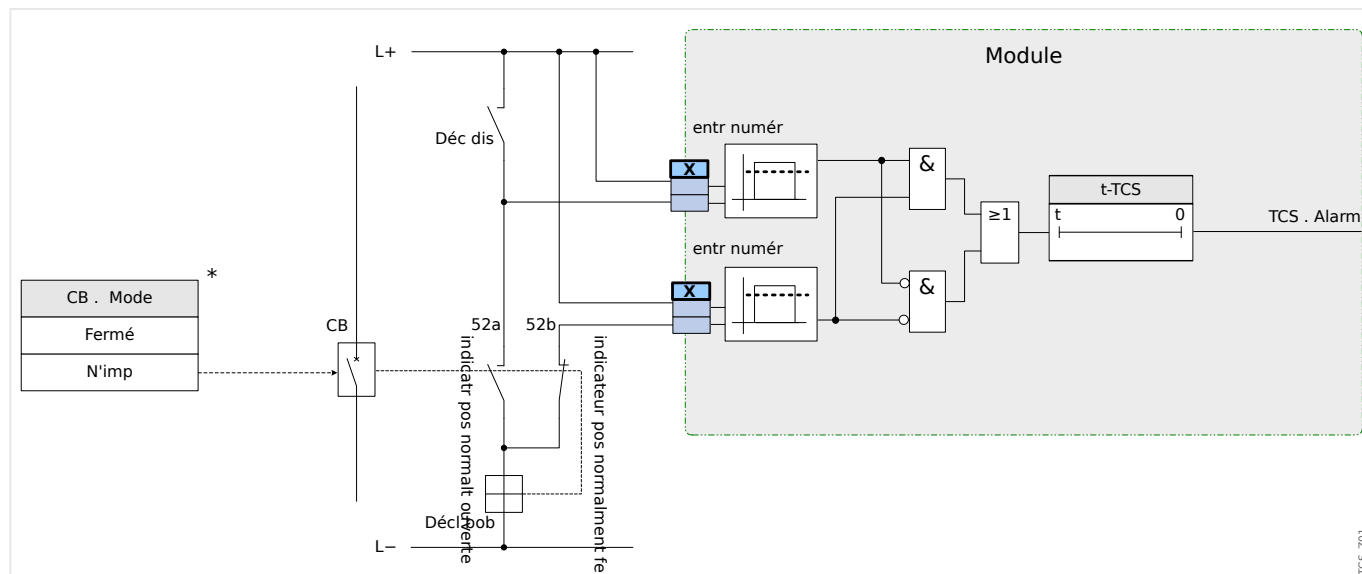
Fig. 60: Exemple de connexion : Surveillance du circuit de déclenchement avec de contacts auxiliaires de disjoncteur »Aux ON« (52a) et »Aux OFF« (52b).
