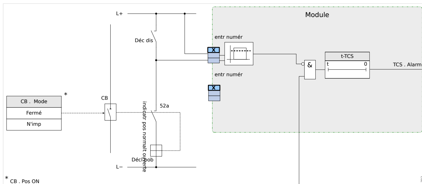
Fig. 61: Exemple de connexion : Surveillance du circuit de déclenchement avec un contact auxiliaire de disjoncteur »Aux ON« (52a).
