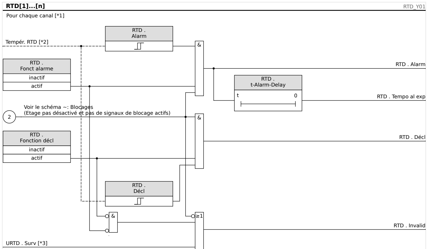
Fig. 59: Principe de fonctionnement général (alarme retardée, déclenchement non retardé).
