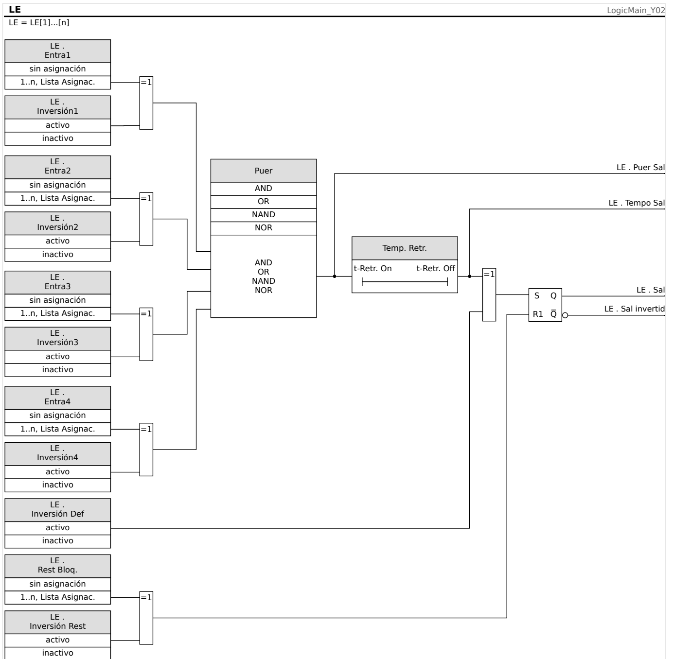
Fig. 75: Descripción detallada - Diagrama de lógica general.
