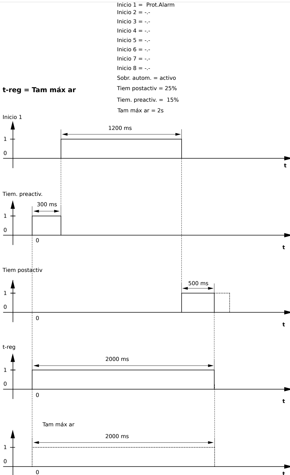
Fig. 71: Ejemplo 1: cuadro de intervalos del registrador de perturbaciones
