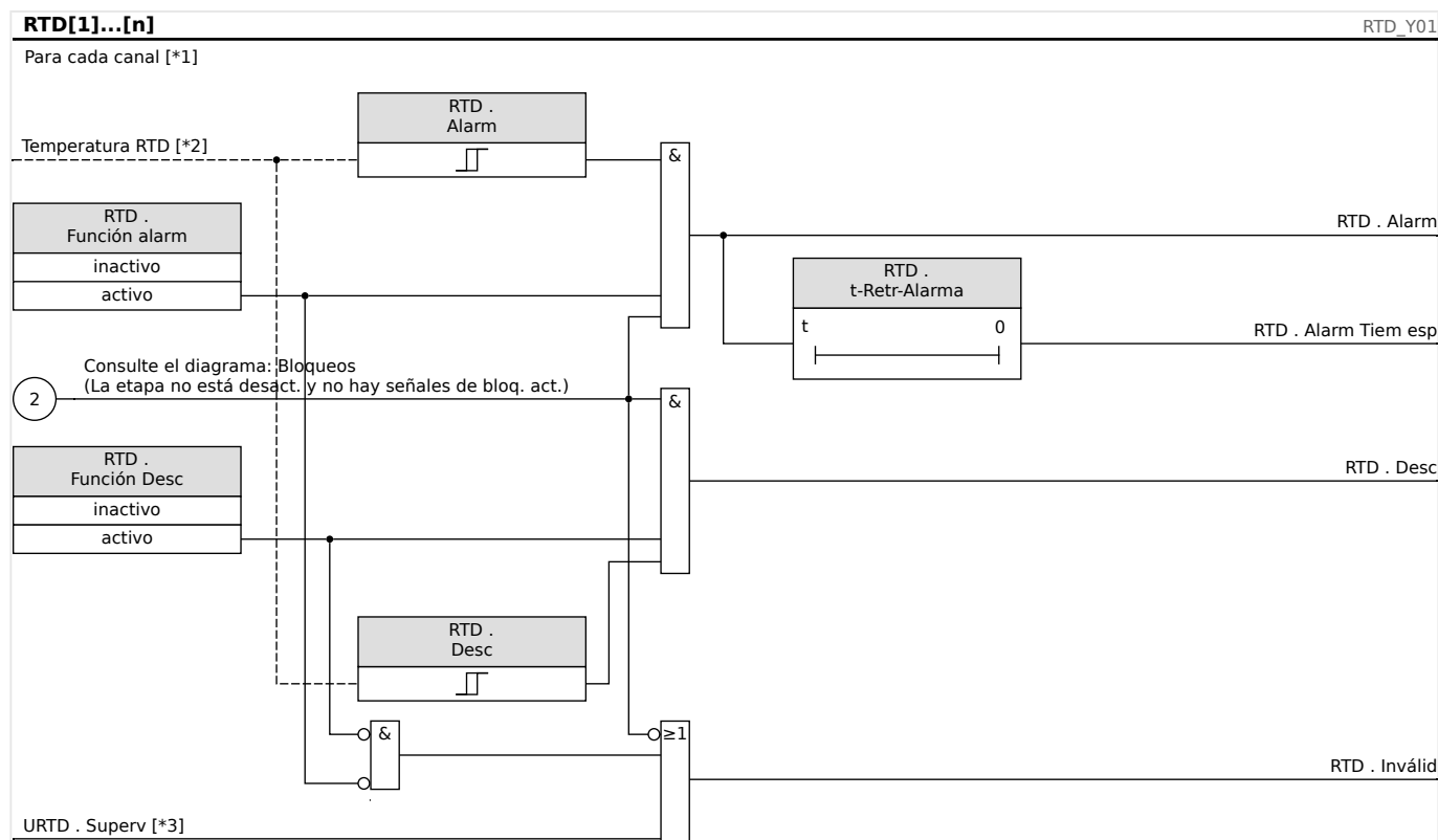
Fig. 59: El principio de funcionamiento general (alarma retrasada, desconexión sin retraso).
