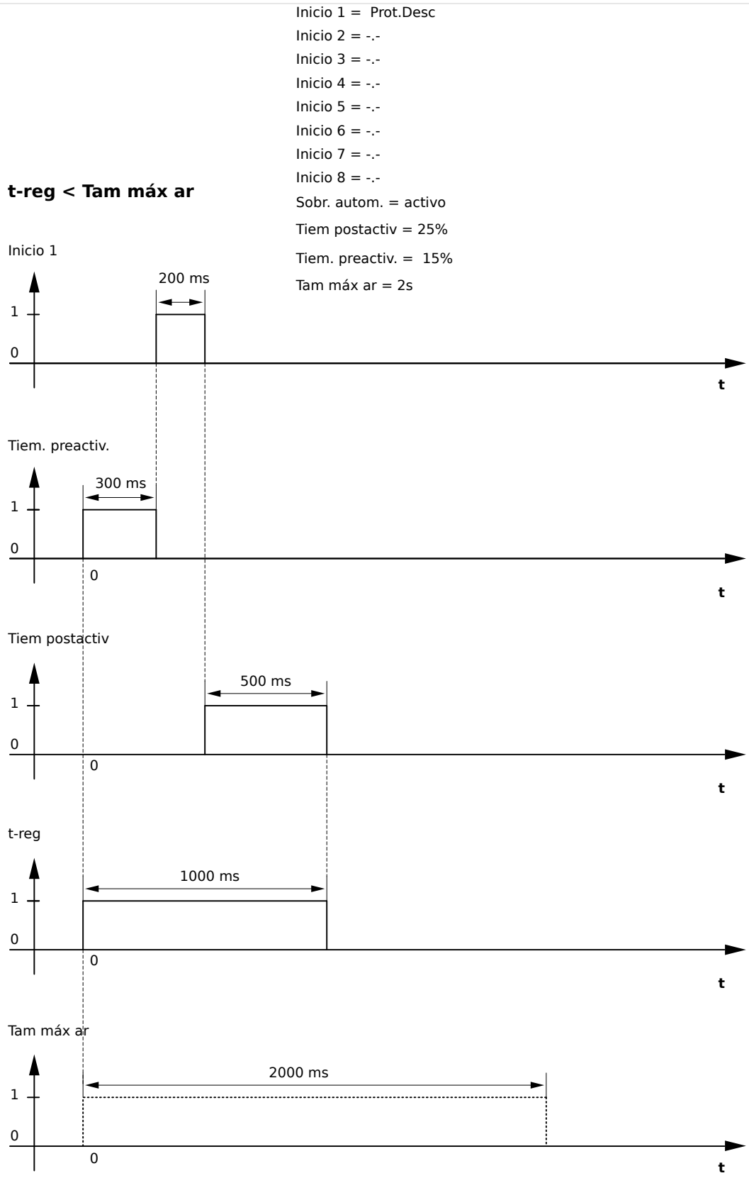
Fig. 72: Ejemplo 2: cuadro de intervalos del registrador de perturbaciones
