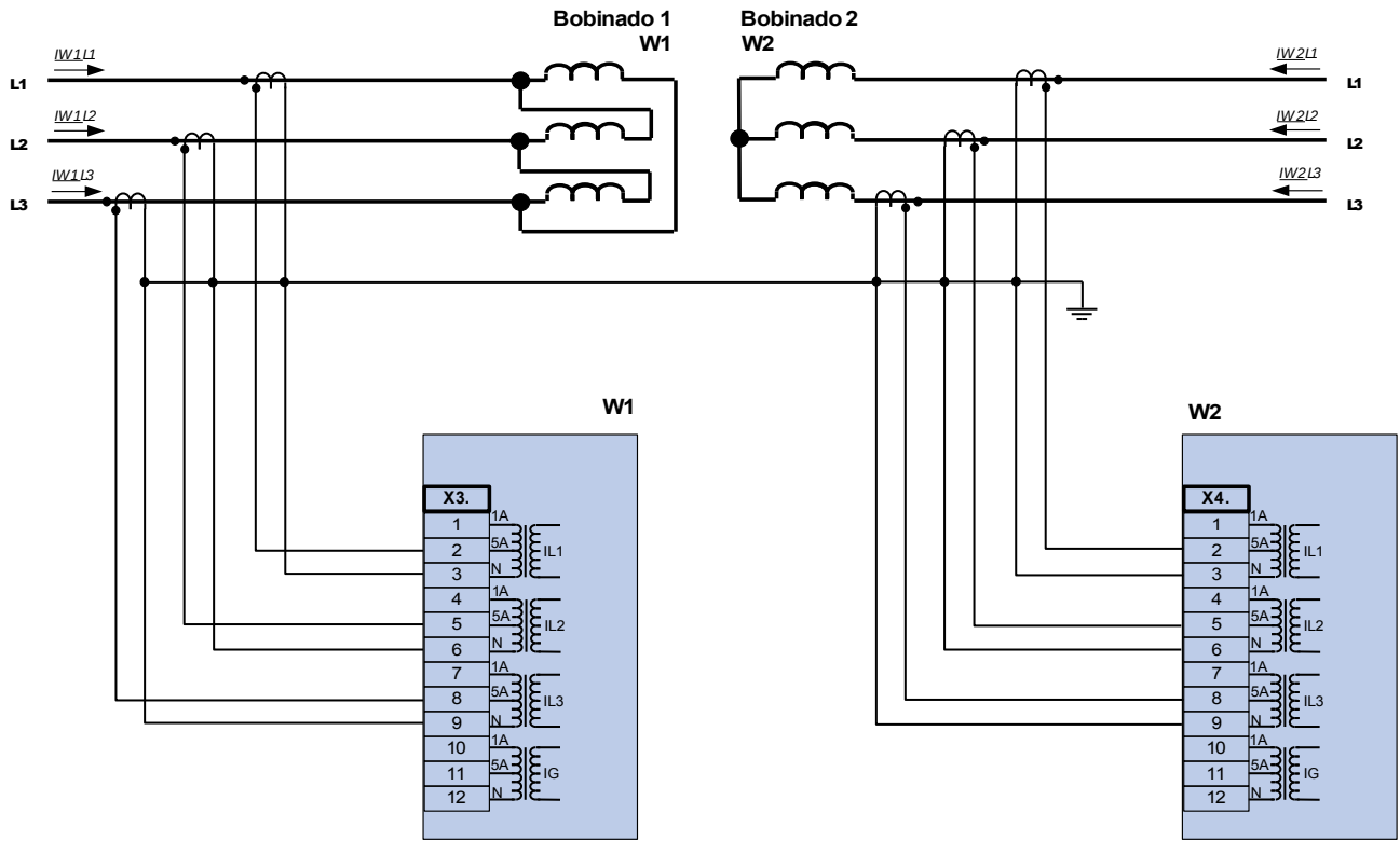
Medida corriente trifásica ; En secundario = 5 A.
