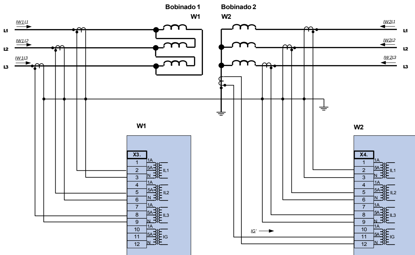
Medida corriente trifásica ; En secundario = 5 A.
