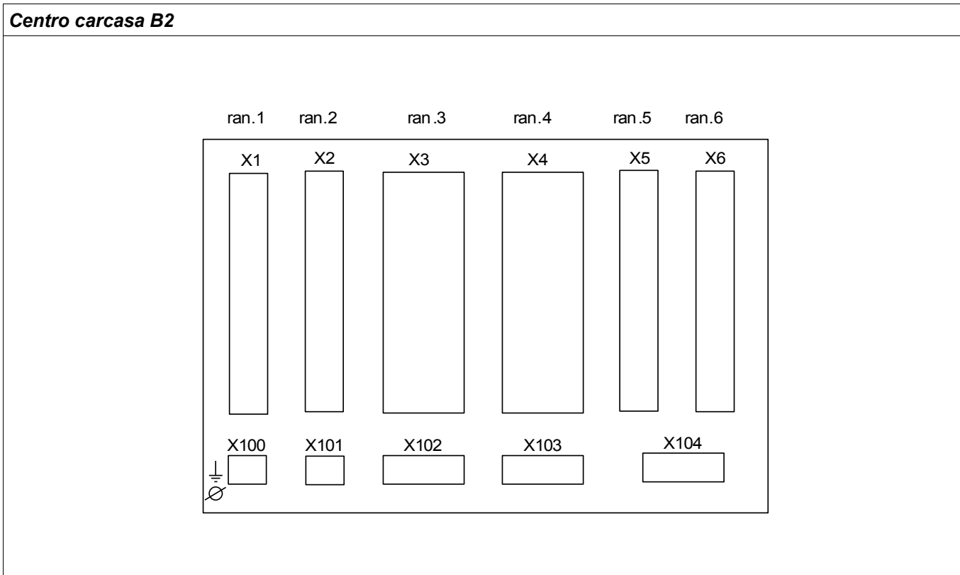
Vista posterior de carcasa B2
