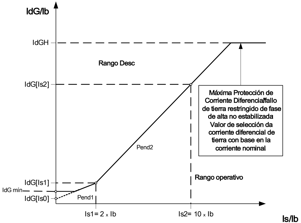
Elemento de protección diferencial de ajuste alto no estabilizado I_{dGH}
