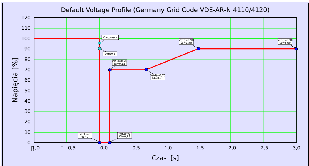
Rys. 88: Profil domyślny LVRT (typ I).
