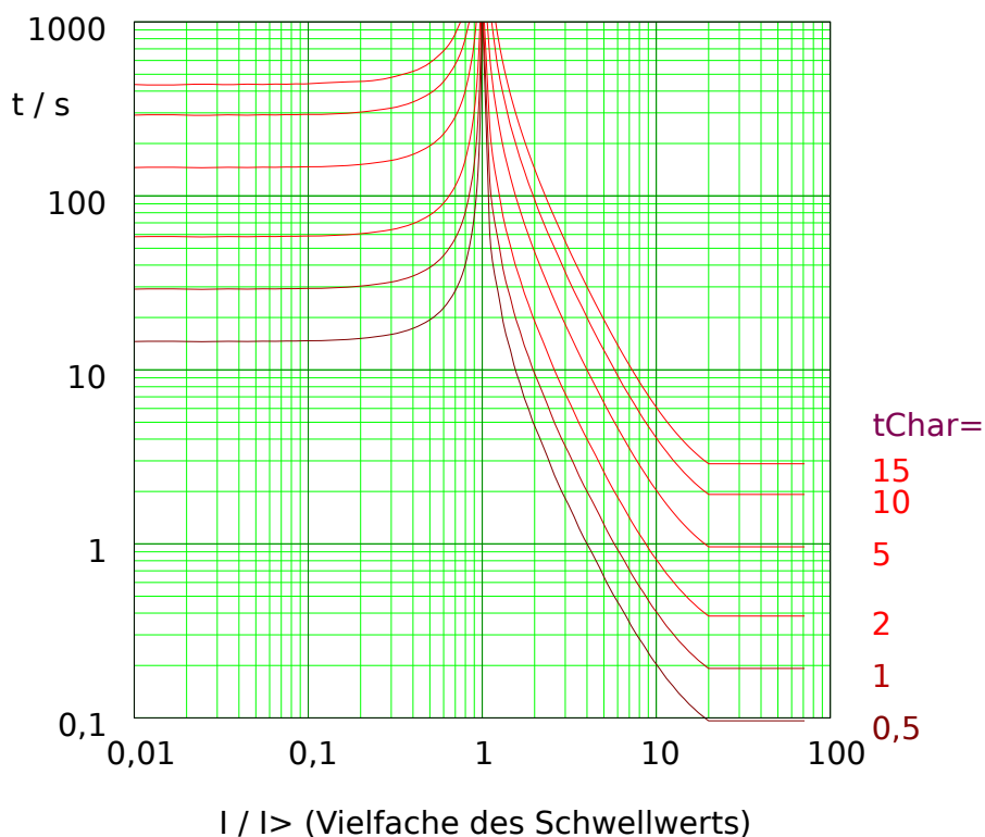
Abb. 77: EINV: Rückfallverzögerung (linke Hälfte, I < I_{>} ) und Auslöseverzögerung (rechte Hälfte, I > I_{>} ), Beispieldiagramm für I_{max} = 20 \cdot I_{>} .
