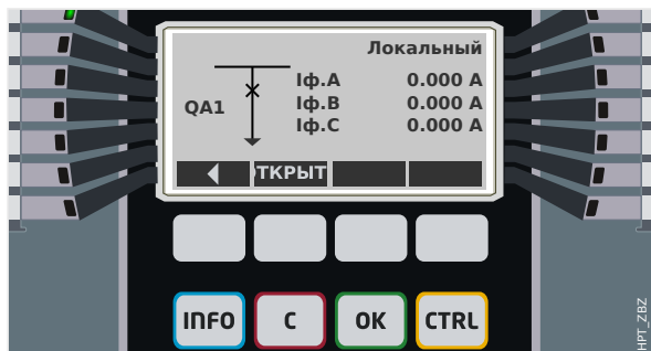
Рис. 118: Пример страницы управления, выключатель в замкнутом положении.
