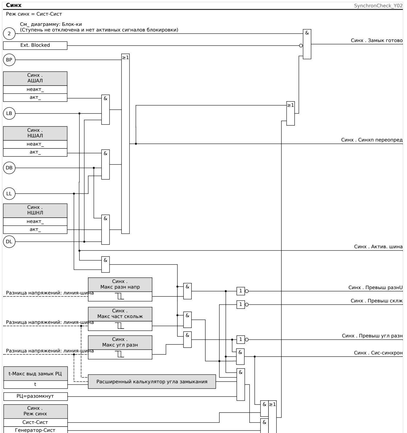
Рис. 111: Принцип работы модуля «Синх», «Сист-Сист».
