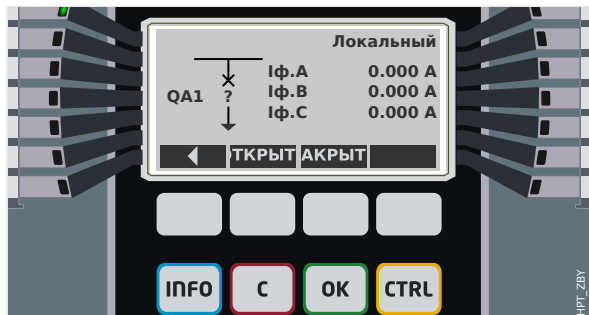
Рис. 119: Пример страницы управления, выключатель в аварийном (недопустимое состояние) положении.
