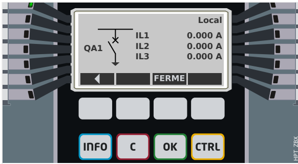
Fig. 120: Exemple de page de contrôle, avec le « disjoncteur » en position ouverte.
