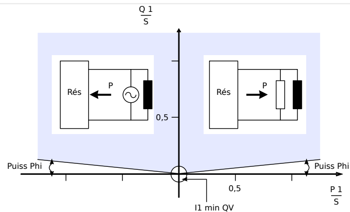
Fig. 90: Méthode 1 : Surveillance de l'angle de charge
