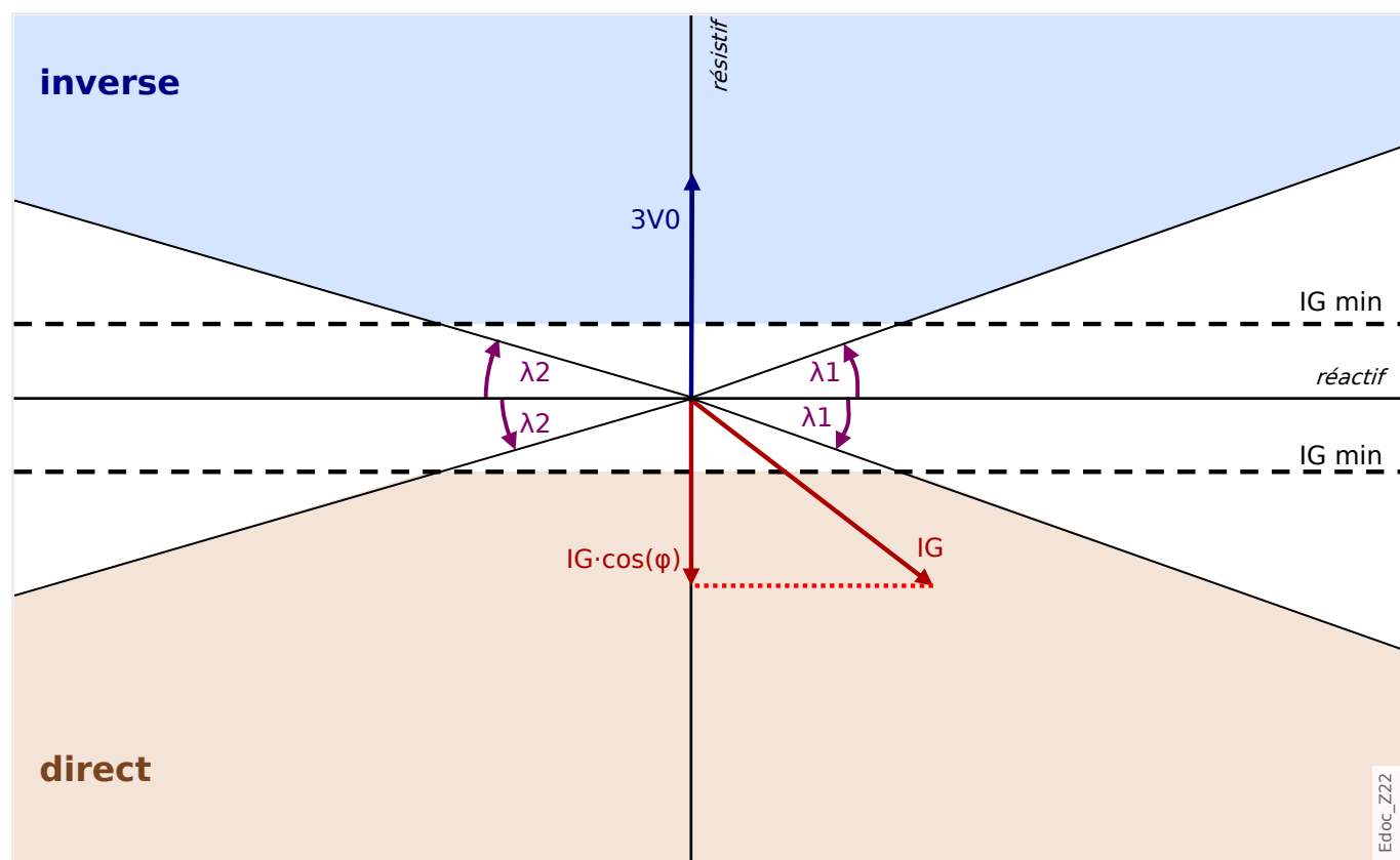
Fig. 65: Principe de détermination de la direction pour la méthode « \cos(\phi) ».
