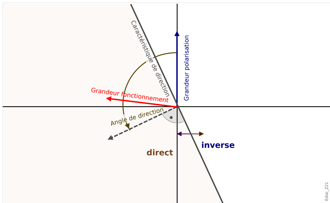
Fig. 63: Principe de détection de la direction pour toutes les méthodes excepté « \cos(\phi) », « \sin(\phi) ».
