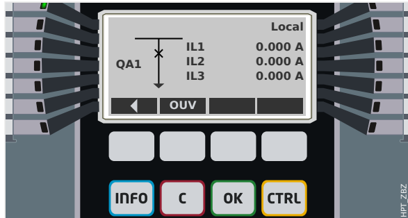
Fig. 118: Exemple de page de contrôle, avec le « disjoncteur » en position fermée.
