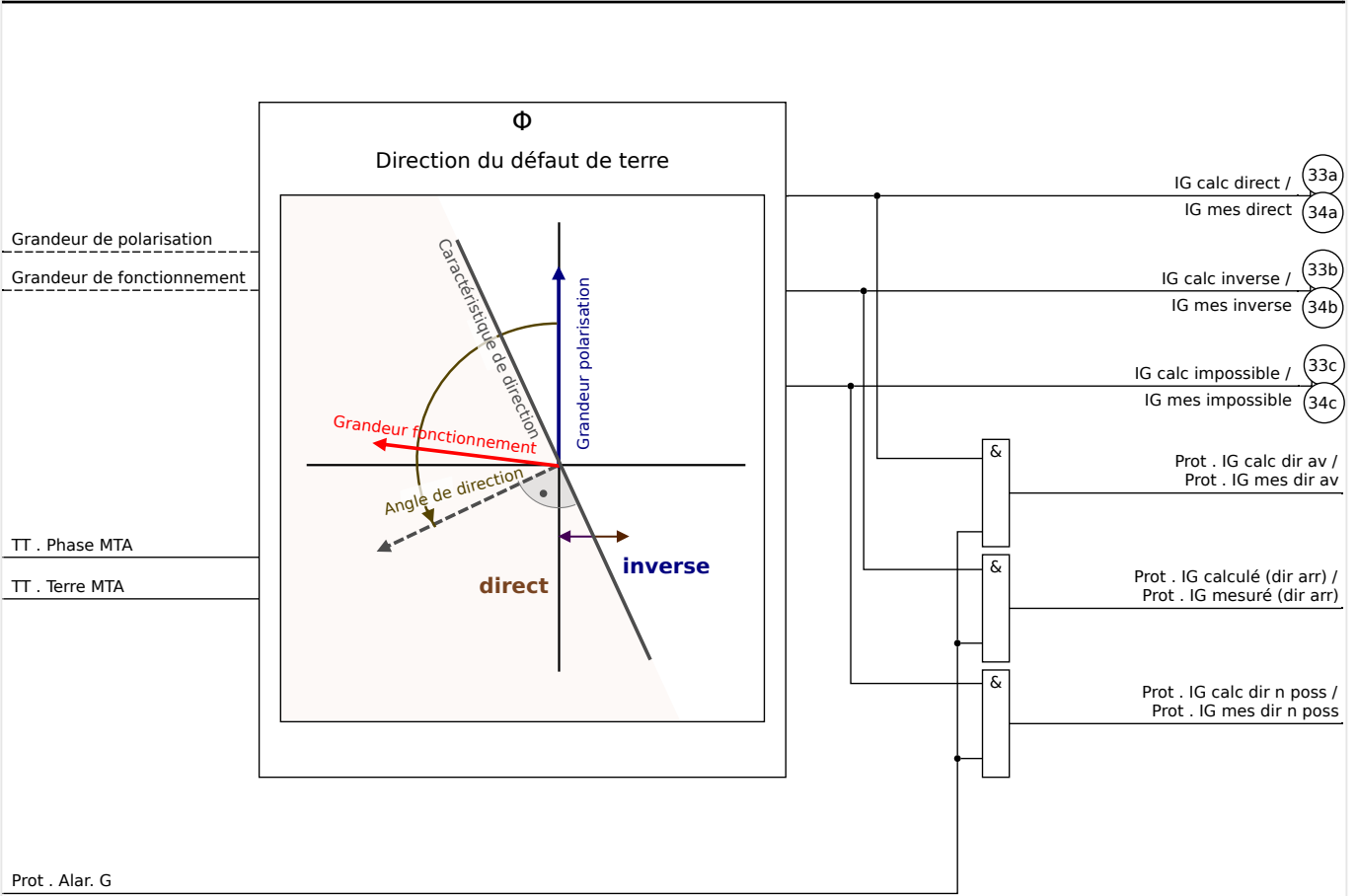
Fig. 64: Détermination de la direction pour toutes les méthodes excepté « \cos(\phi) », « \sin(\phi) ».
