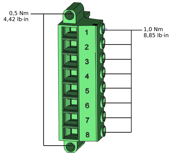
Fig. 139: Bornes de mesure de tension de la carte de mesure « TU » (↳ « TU - Entrées de mesure de tension »).
