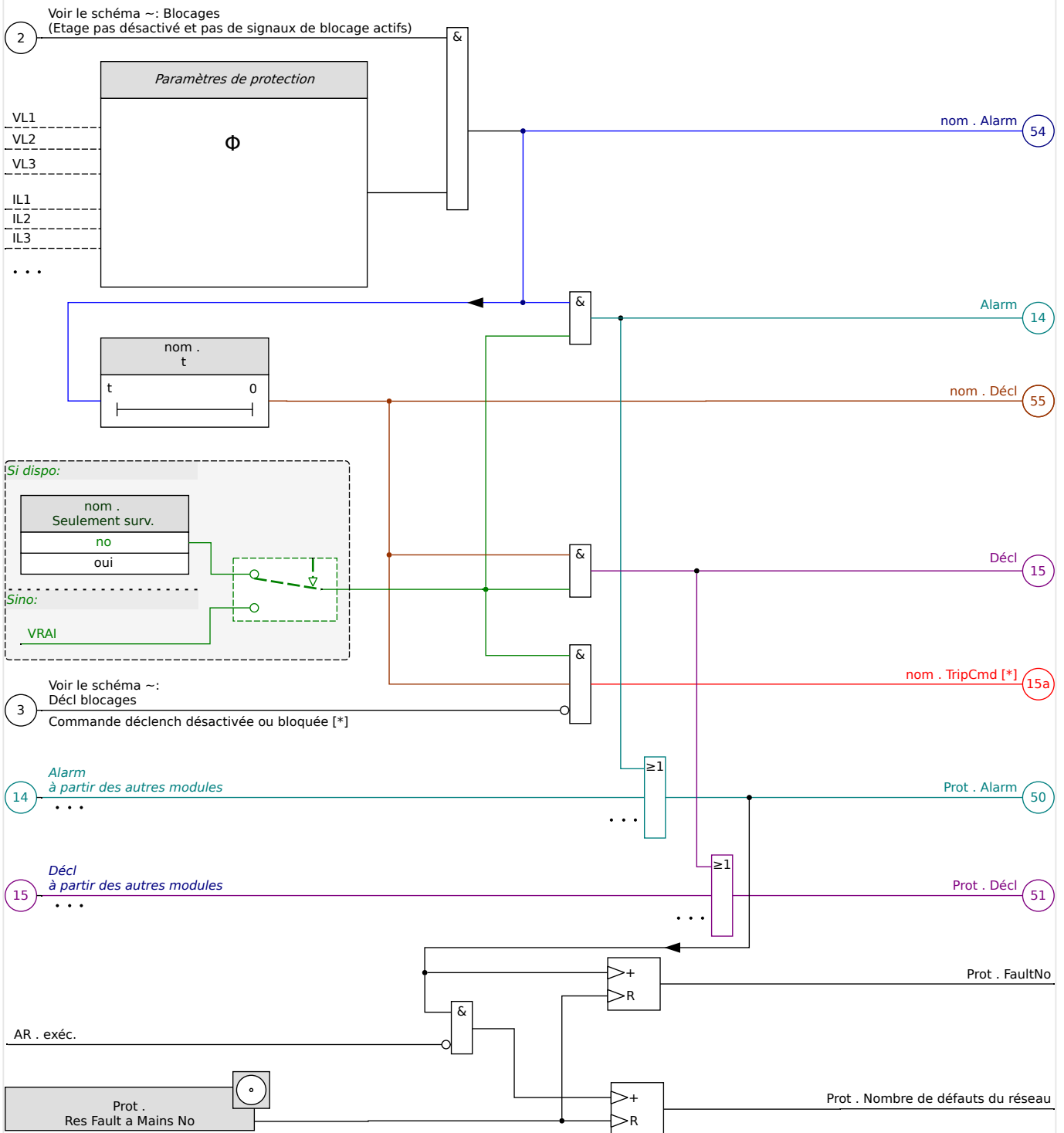
Fig. 60: Schéma de fonctionnalité des éléments de protection HighPROTEC.
