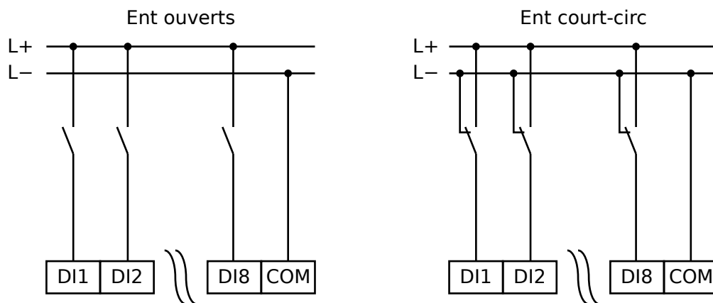
Fig. 141: État sécuritaire des entrées numériques
