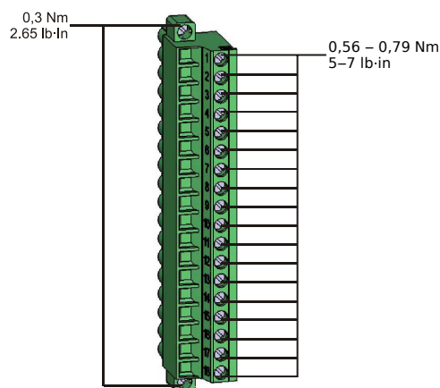
Fig. 140: Bornes de mesure de tension des cartes de mesure « TU-OR5 » et « TU-DI8 ».
