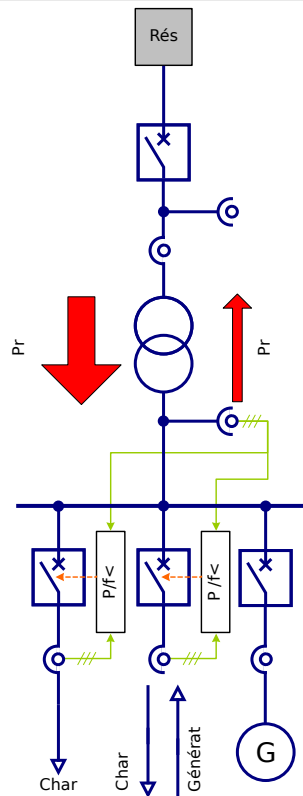
Fig. 95: Délestage de charge de sous-fréquence décentralisé au sein de réseaux avec alimentation temporaire.
