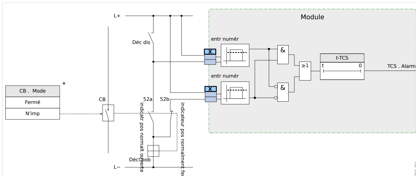
Fig. 114: Exemple de connexion : Surveillance du circuit de déclenchement avec de contacts auxiliaires de disjoncteur »Aux ON« (52a) et »Aux OFF« (52b).
