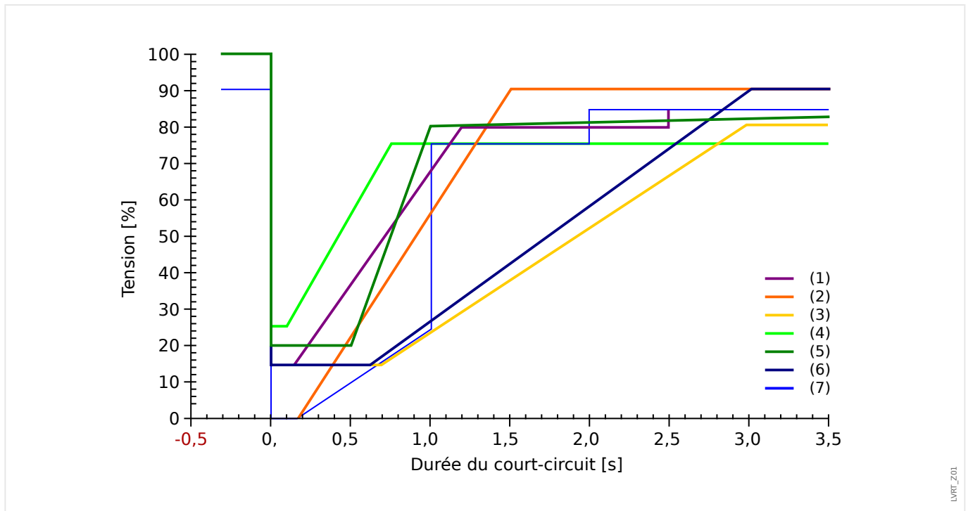
Fig. 76: Normes LVRT ; source : eBWK Bd. 60 (2008) N° 4. Auteurs: Dipl.-Ing. Thomas Smolka, Dr.-Ing. Karl-Heinz Weck, Zertifizierungstelle der FGH e.V., Mannheim, sowie Dipl.-Ing. (FH) Matthias Bartsch, Enercon GmbH, Aurich.
