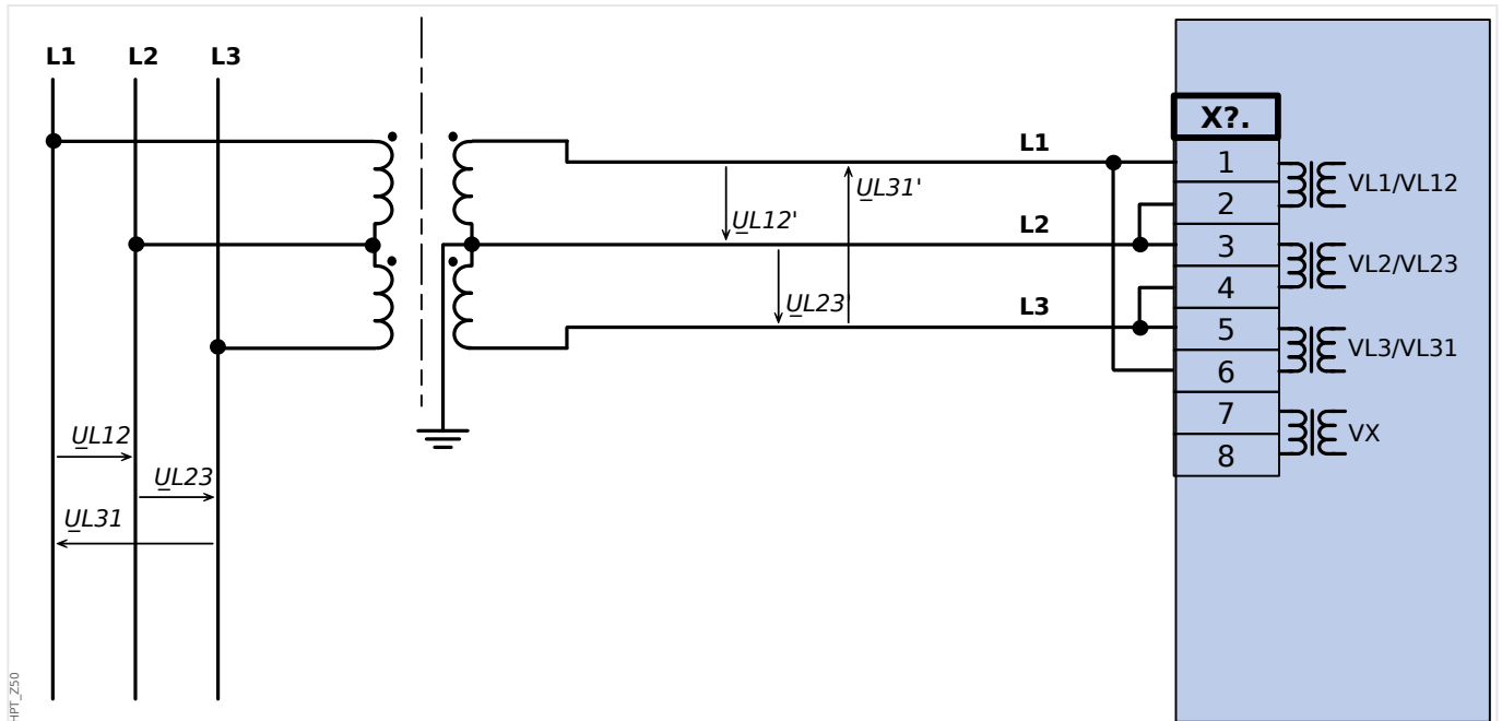
Fig. 34: Mesure de tension biphasée - câblage des entrées de mesure: "Triangou"
