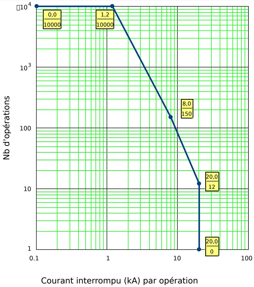
Fig. 123: Courbe de maintenance du disj pour un disj 25 ~kV typique
