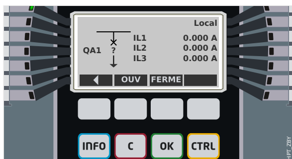
Fig. 119: Exemple de page de contrôle, avec le « disjoncteur » en position de dysfonctionnement (ou invraisemblable).
