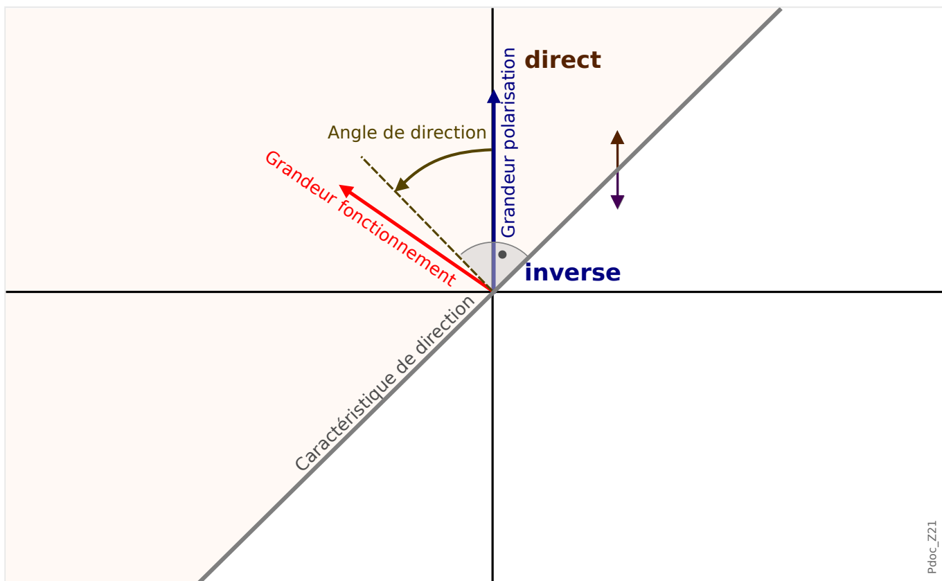
Fig. 61: Principe de la détection de la direction des défauts de phase.
