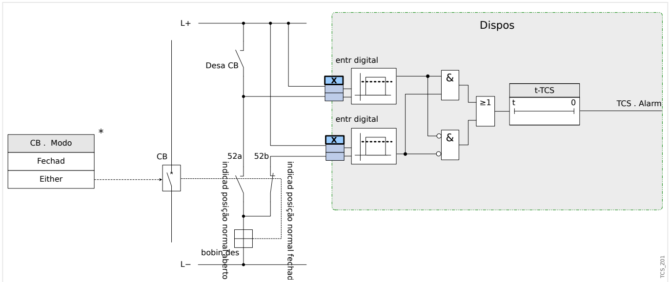
Fig. 123: Exemplo de conexão: Supervisão do circuito de disparo com dois contatos CB auxiliares »Aux ON« (52a) e »Aux OFF« (52b).
