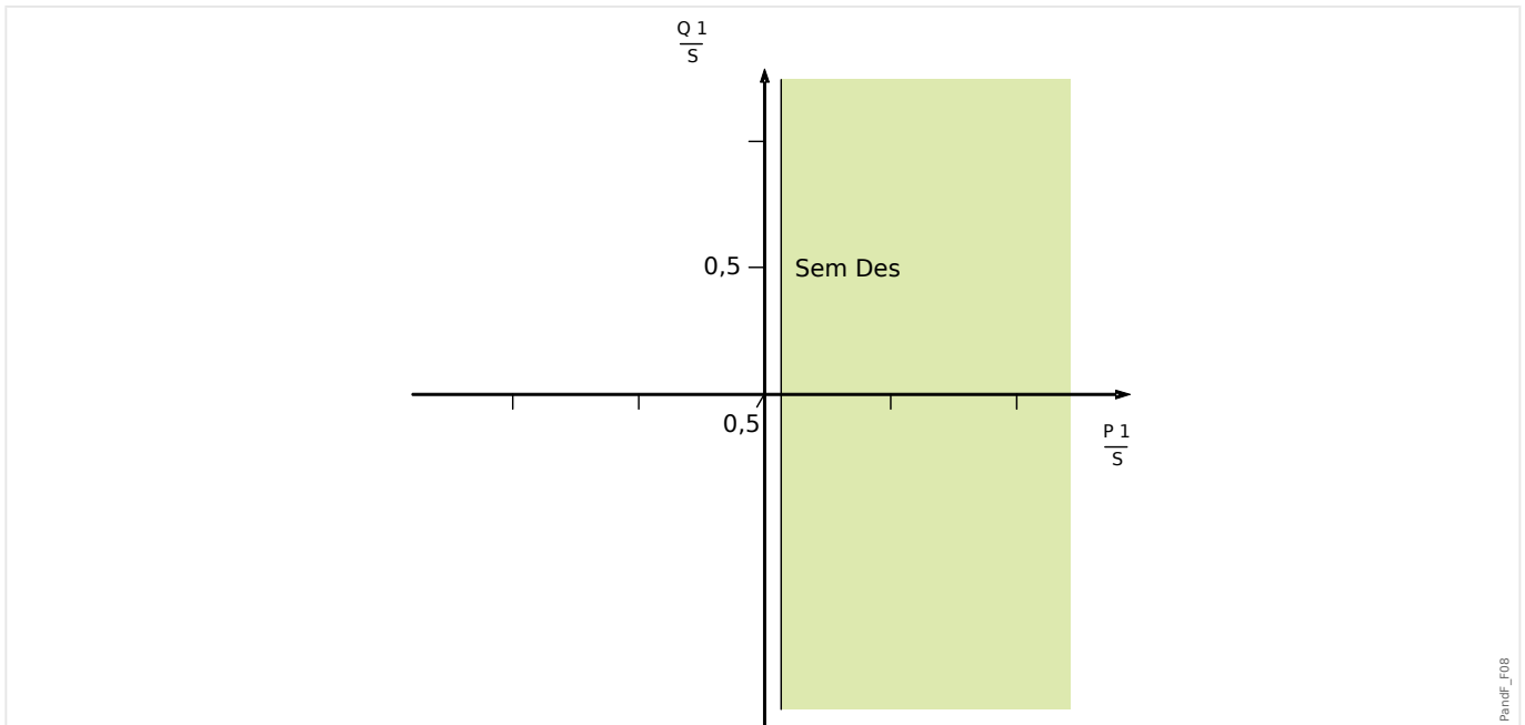
Fig. 108: Método 2 (Supervisão de Energia Ativa Pura): “Método UFLS” = “Superv. de Energia Ativa Pura”.
