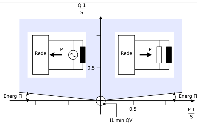
Fig. 99: Método 1: Supervisão Âng Energ.
