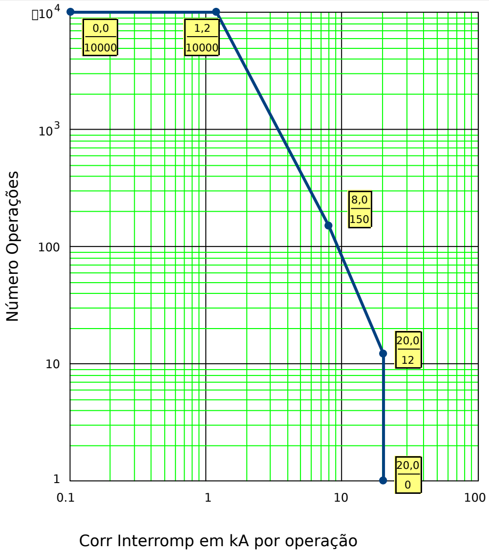
Fig. 132: Curva Manutenção de Disjuntor para Disjuntor normal 25kV
