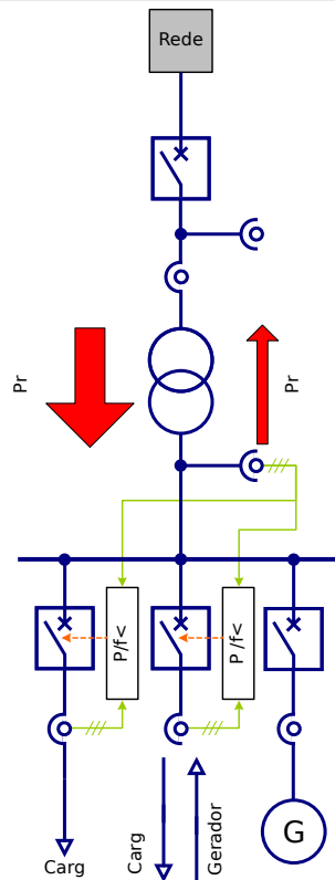
Fig. 104: Eliminação de carga de subfrequência descentralizada em redes com fornecimento temporário de energia.
