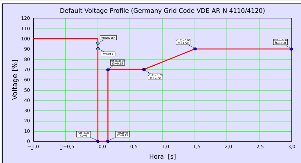
Fig. 88: Perfil padrão do LVRT (Tipo I).
