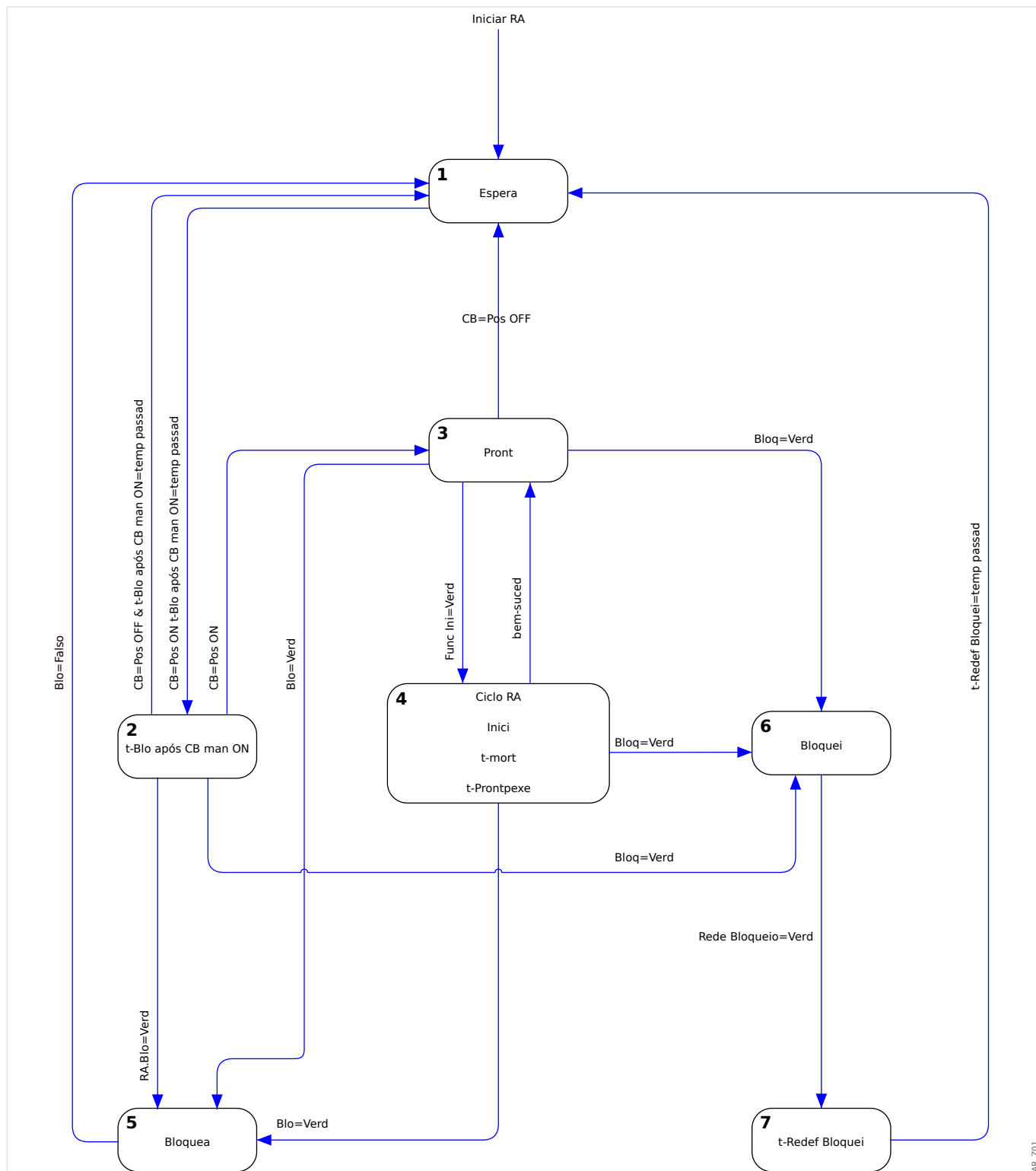
Fig. 109: Diagrama de estado de transição
