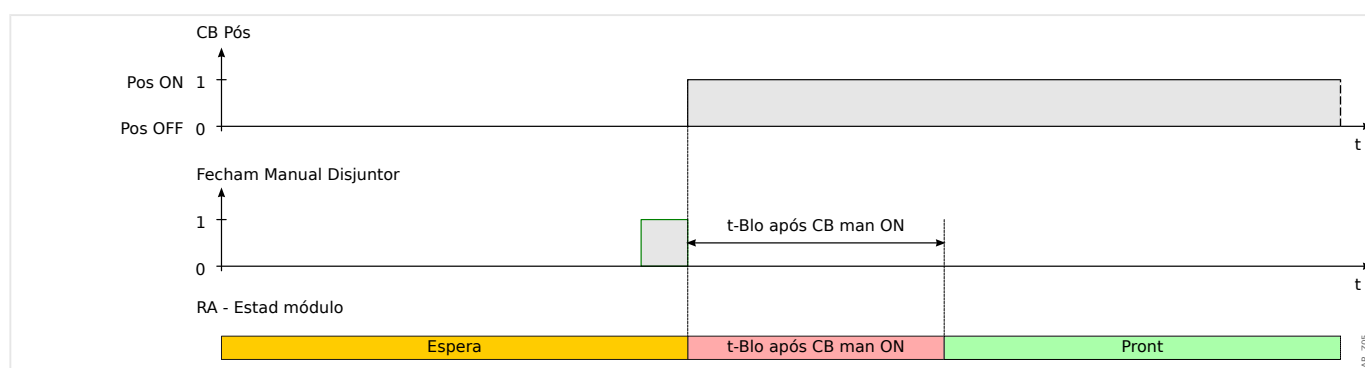
Fig. 113: Estados de religamento automático durante fechamento manual do disjuntor
