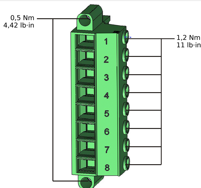
Rys. 146: Zaciski pomiaru napięcia karty pomiarowej „TU” (↳ „2.6.1 TU – wejścia do pomiaru napięcia”).
