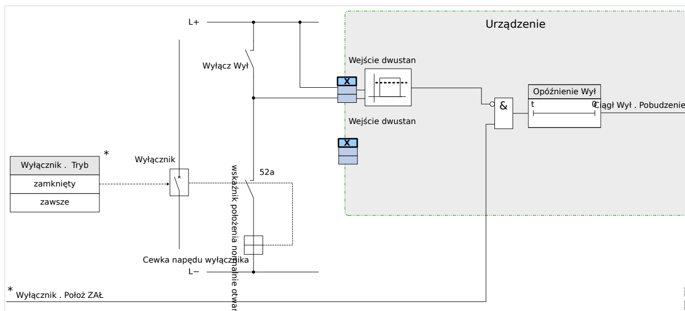
Rys. 124: Przykład okablowania: Układ kontroli ciągłości obwodów wyłącznika z tylko jednym stykiem pomocniczym wyłącznika „Położ ZAŁ” (52a).
