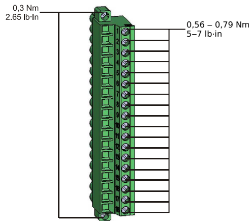
Rys. 147: Zaciski pomiaru napięcia kart pomiarowych „TU-OR5” i „TU-DI8”.
